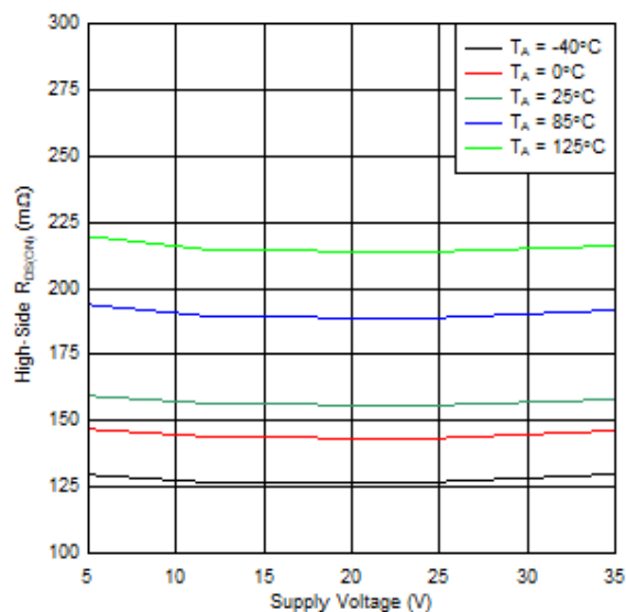
図 6-7. ハイサイド R_{DS(ON)} と電源電圧
