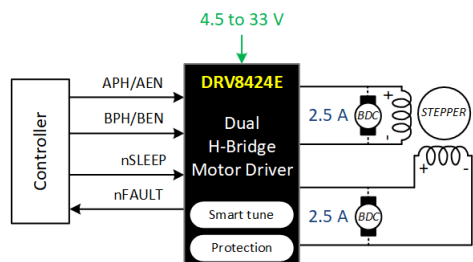
DRV8424E の概略回路図
