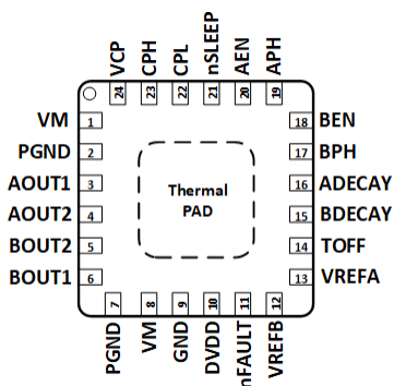
図 5-2. RGE パッケージ 24 ピン VQFN (露出サーマル・パッド付き) 上面図 DRV8424E、DRV8425E
