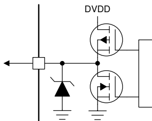
図 7-24. プッシュプル出力構造 (SDO)
