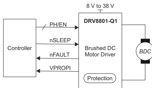
概略回路図
