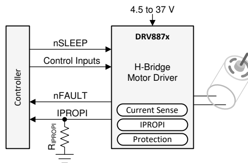
概略回路図
