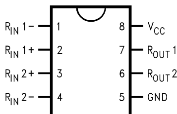
接続図
