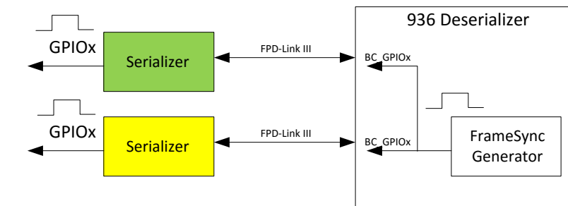
图 7-18. Internal FrameSync
