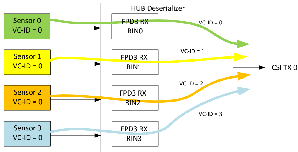
図 7-11. VC-ID Mapping Example 1
