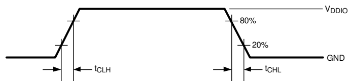
图 6-3. LVCMOS Transition Times
