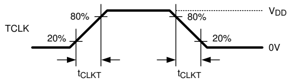
図 5-4. シリアルライザの入力クロック 遷移時間
