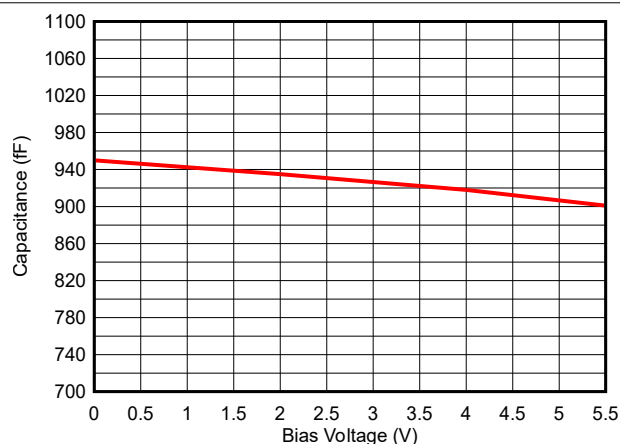
図 5-5. バイアス電圧と静電容量との関係
