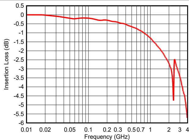
図 5-8. 挿入損失
