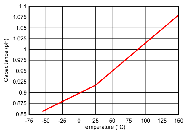
図 5-6. 温度と容量との関係
