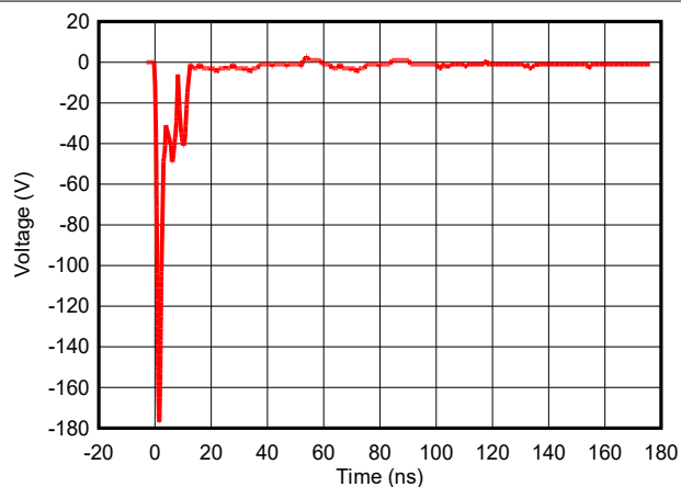
図 5-4. -8kV クランプ IEC 波形
