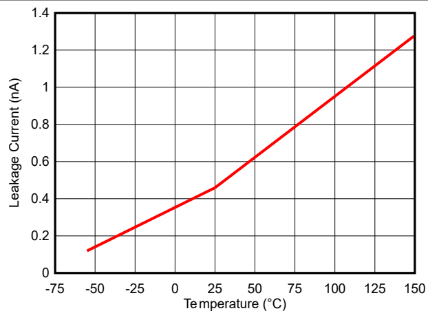
図 5-7. 温度とリーク電流との関係
