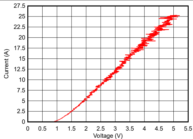
図 5-2. 負の TLP 曲線
