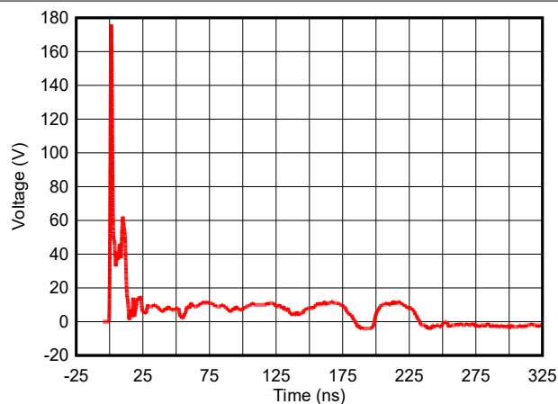
図 5-3. +8kV クランプ IEC 波形
