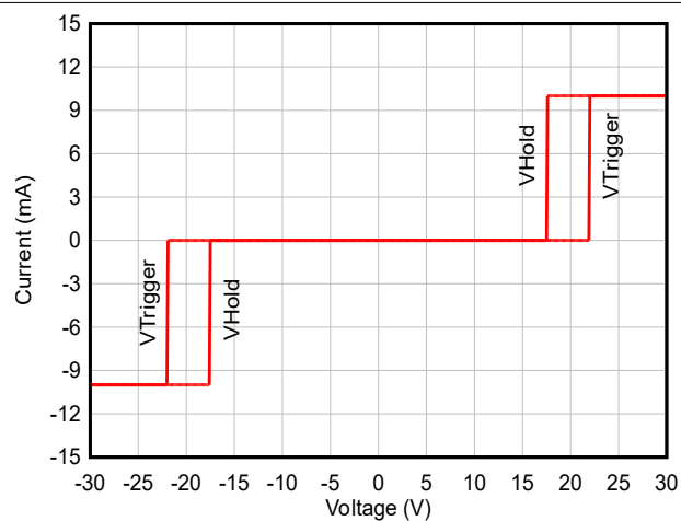
図 5-8. DC-IV 曲線
