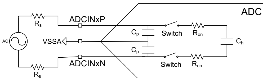
図 6-36. 差動入力モデル
