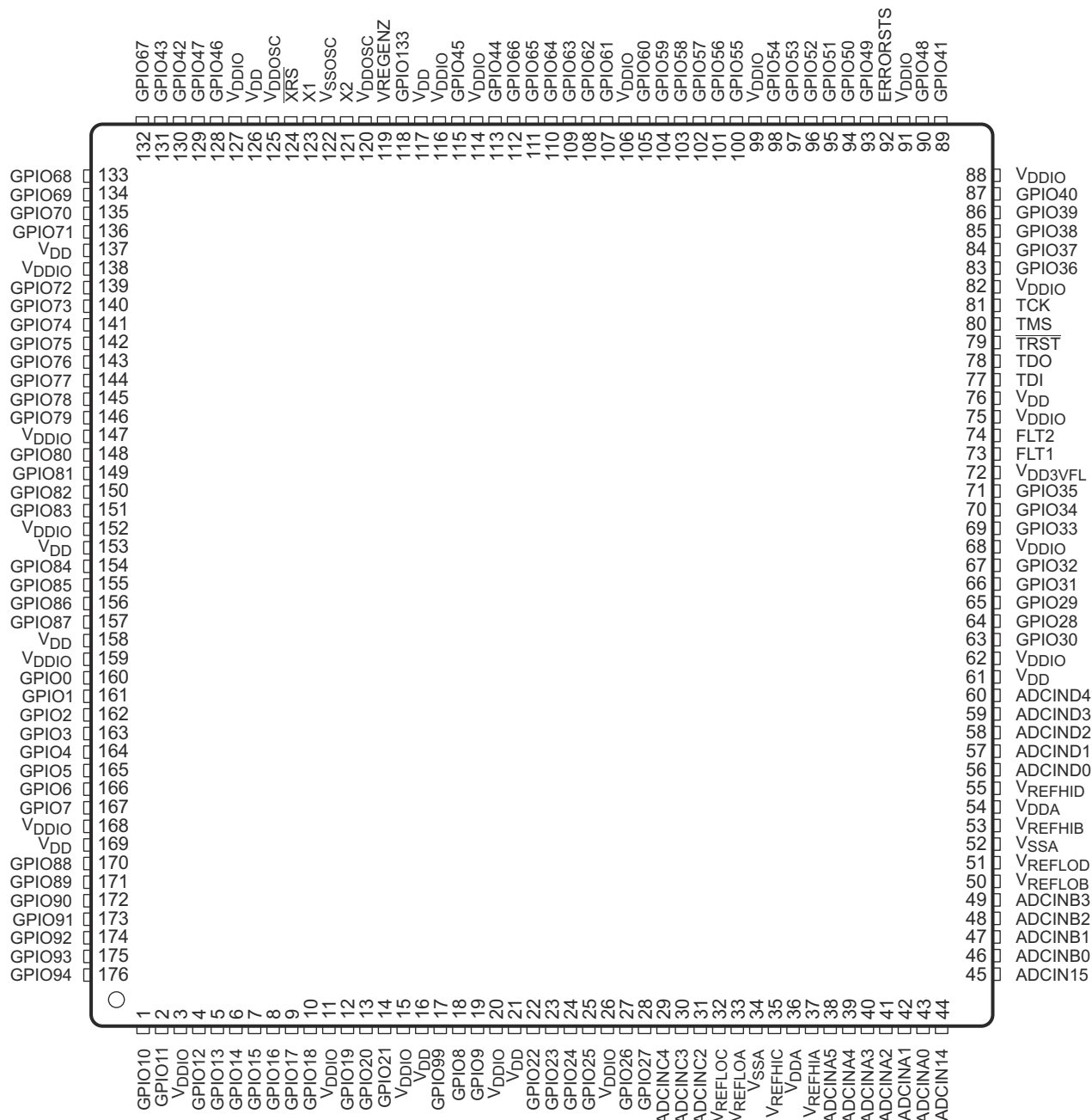
図 5-1. 176 ピン PTP PowerPAD 熱的に強化された薄型クワッド フラットバック (上面図)
