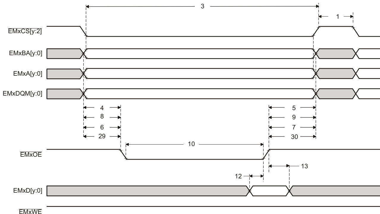
図 6-26. 非同期メモリ読み取りタイミング
