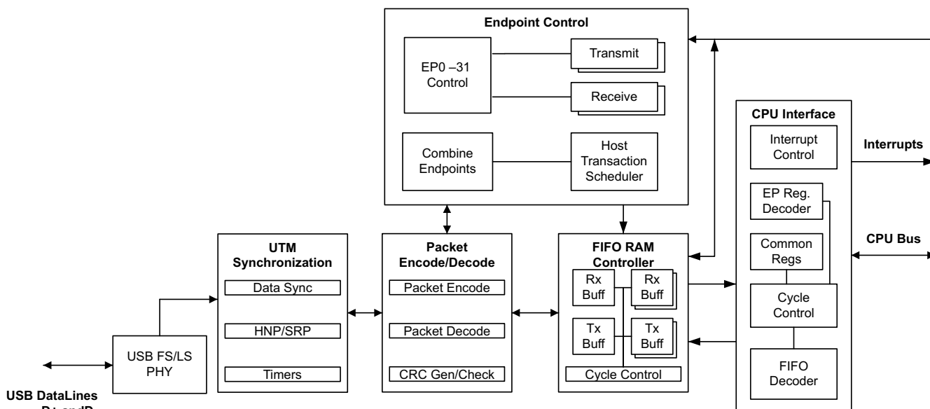
図 6-79. USB ブロック図
