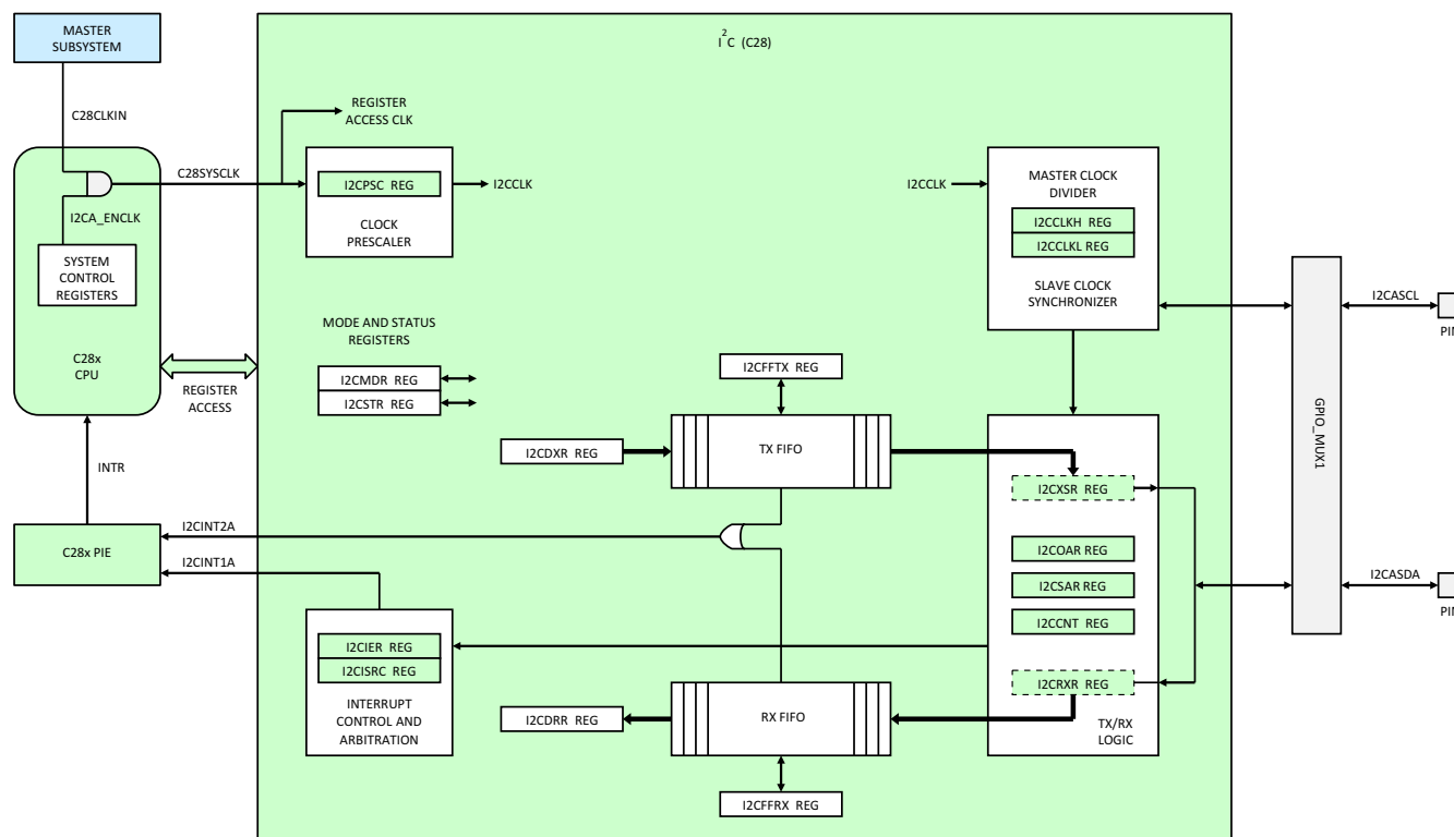
図 7-48. I2C (C28x)
