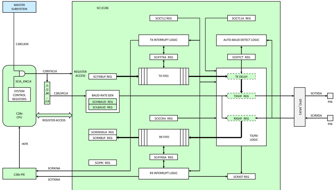
7-49. SCI (C28x)
