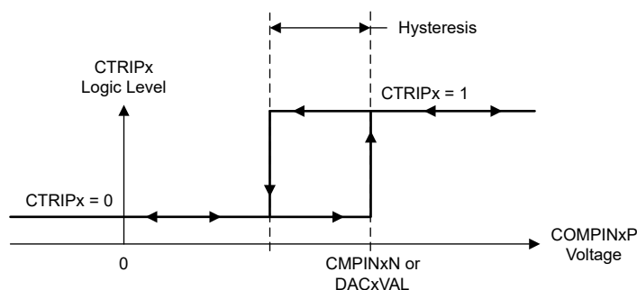
図 6-57. CMSS コンパレータのヒステリシス
