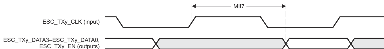
図 6-93. EtherCAT 送信インターフェースのタイミング (MII 動作)
