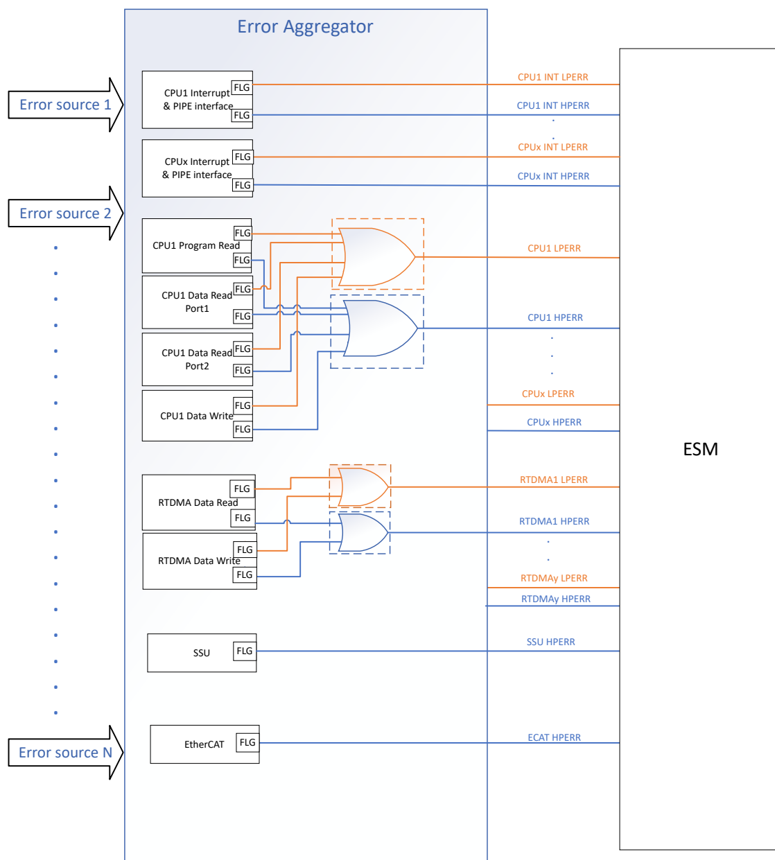
図 7-5. エラー アグリゲータ インターフェイス
