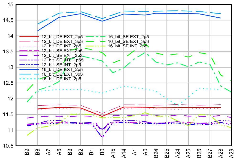
図 6-39. 100 ピン PZS のチャンネルあたりの ENOB – ADC チャンネル A および B
