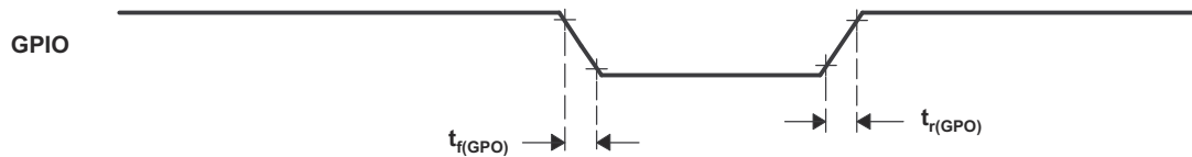
図 6-20. 汎用出力のタイミング
