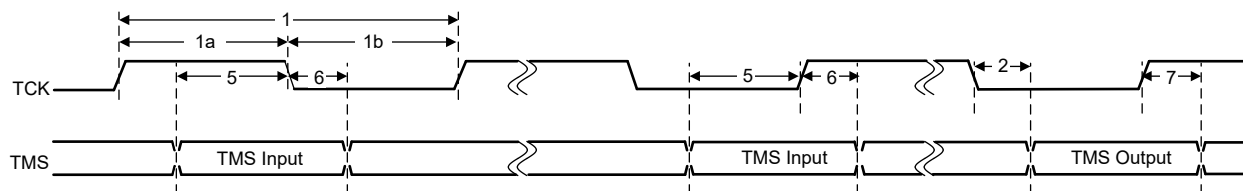
図 6-19. SWD のタイミング
