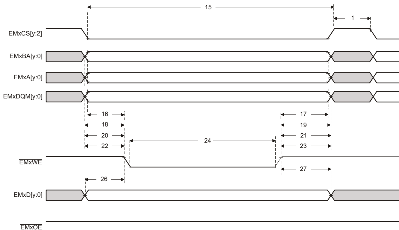
図 6-30. 非同期メモリ書き込みタイミング
