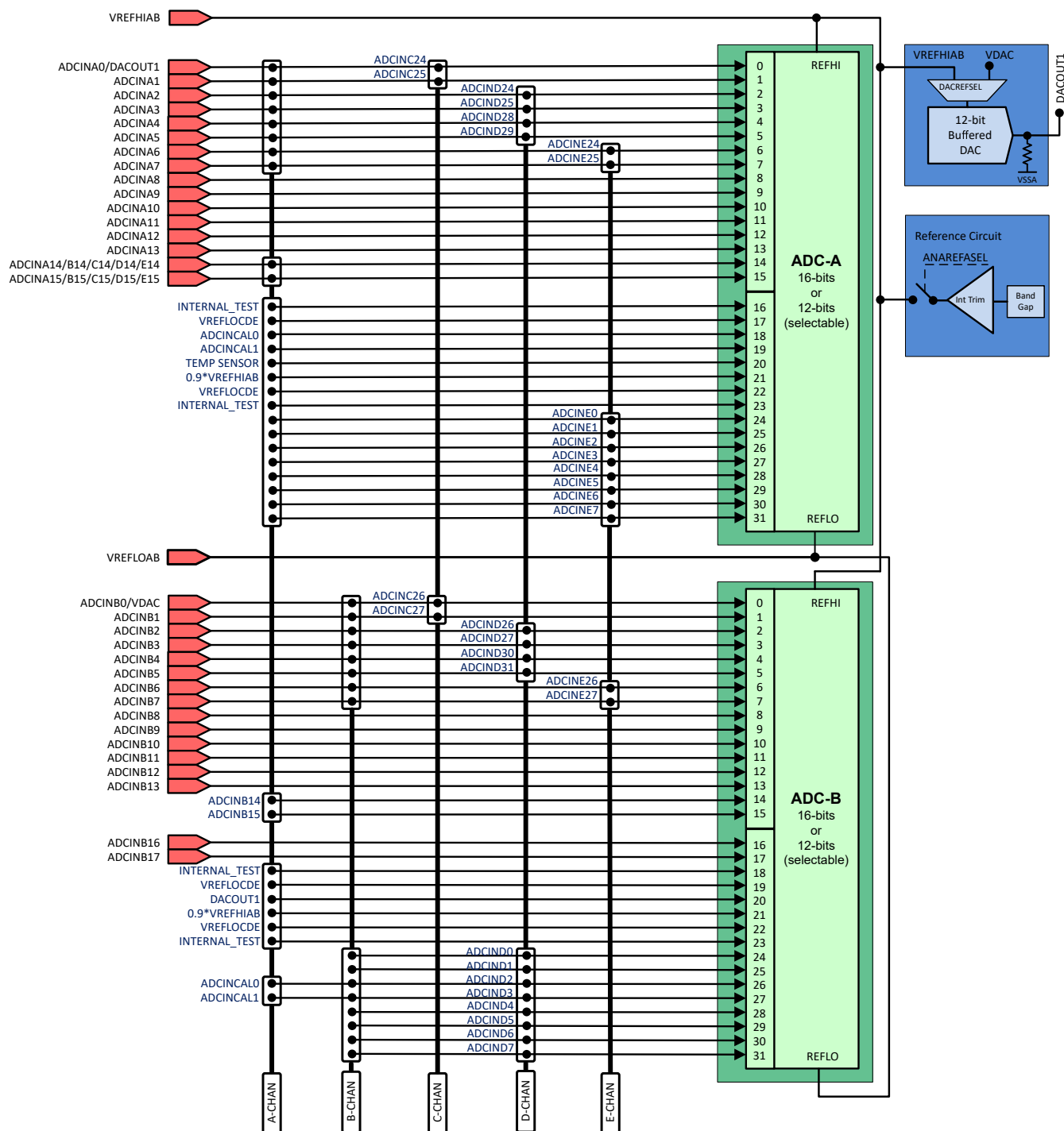
図 6-32. アナログ サブシステムのブロック図 (ADC A および ADC B)
