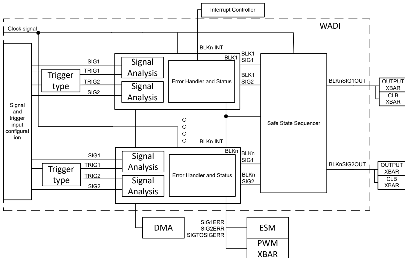
図 7-18. WADI のブロック図
