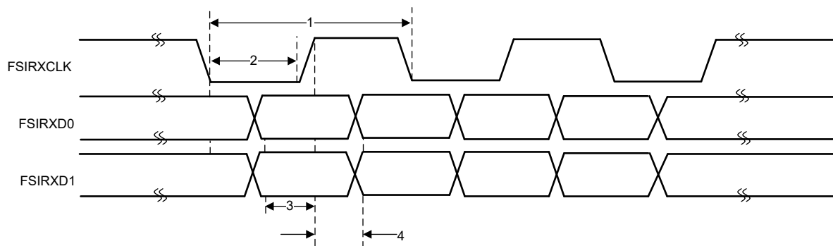
図 6-80. FSIRX タイミング
