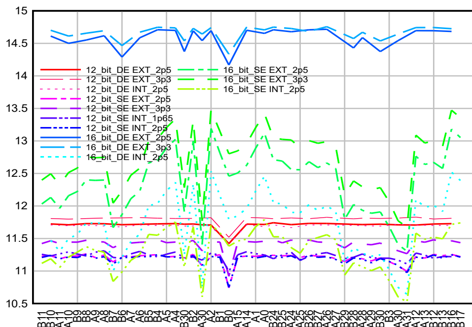
図 6-45. 256 ピン ZEX のチャンネルあたりの ENOB – ADC チャンネル A および B
