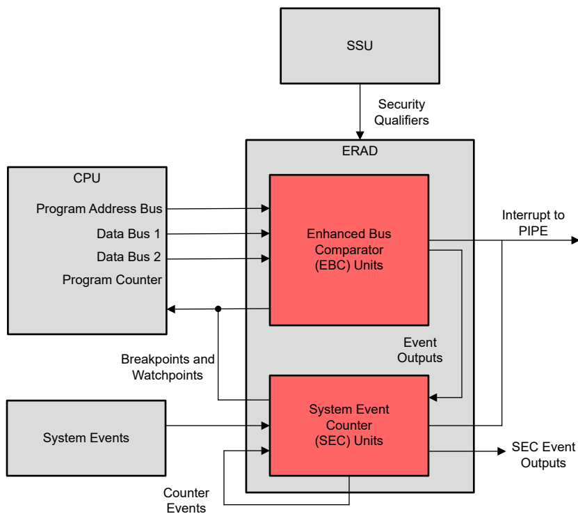
図 7-19. ERAD システムの概要
