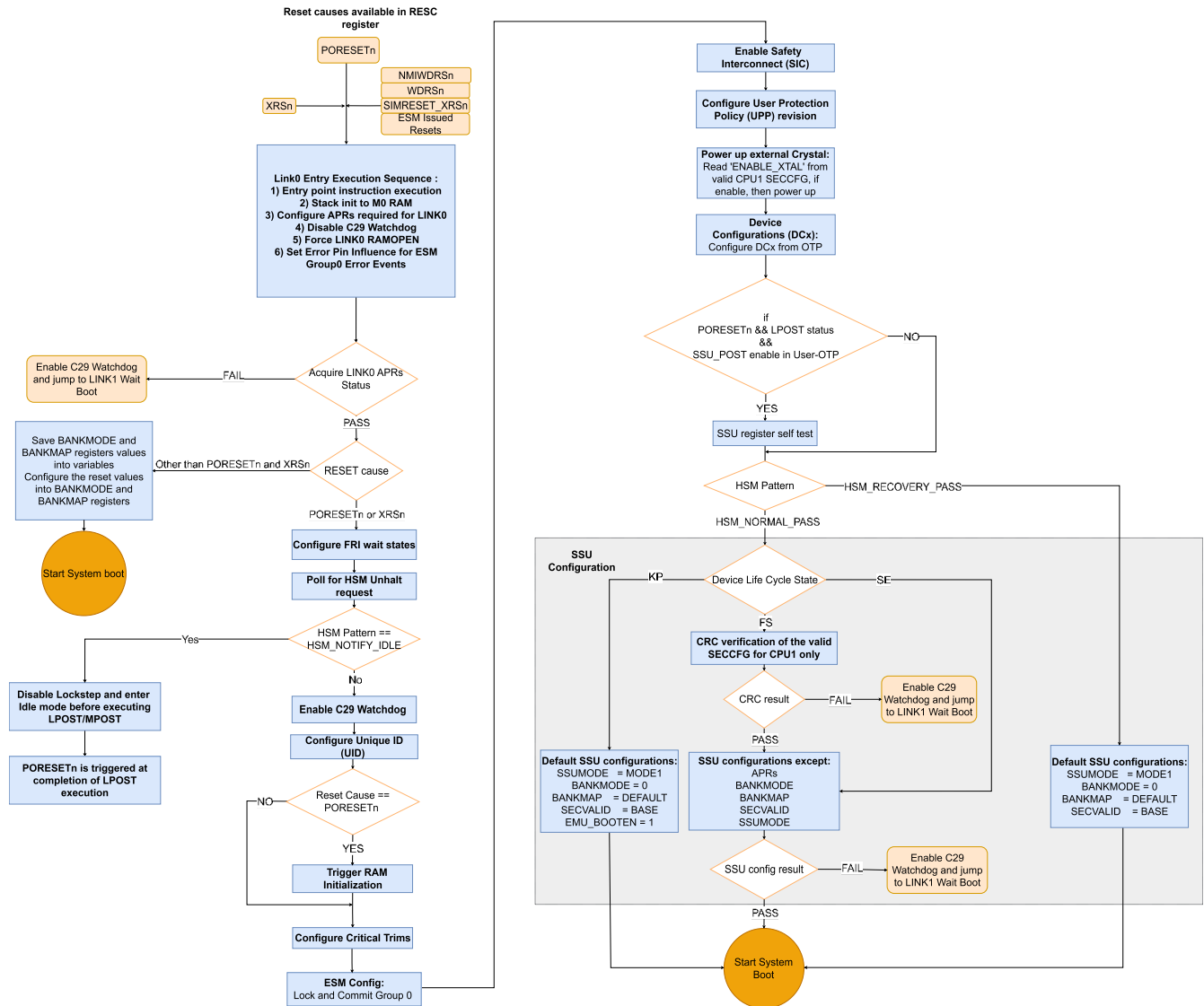
図 7-8. リセットからシステム ブートまでのデバイス ブート フロー
