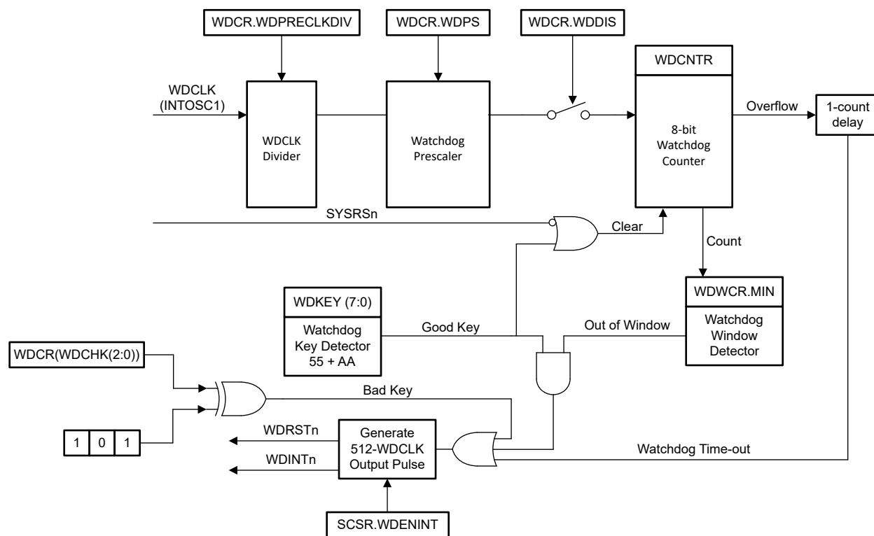
図 7-21. ウィンドウ ウォッチドッグ
