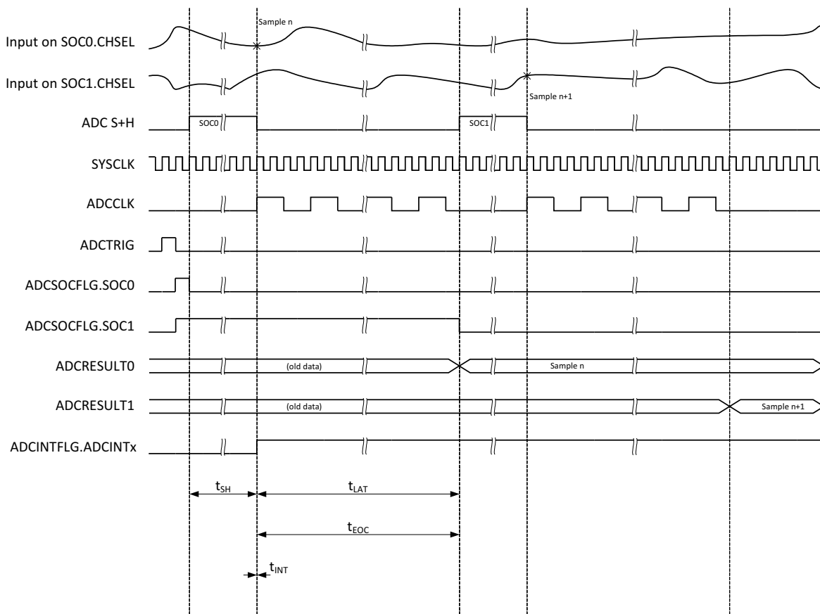
図 6-51. 16 ビット モードの Early 割り込みモードでの ADC タイミング
