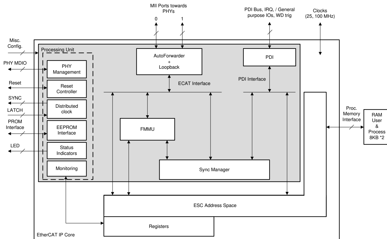
図 6-91. EtherCAT IP のブロック図
