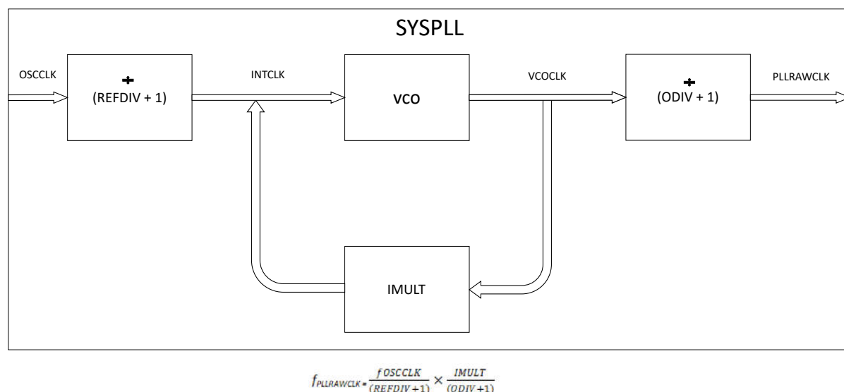
図 6-10. SYSPLL
