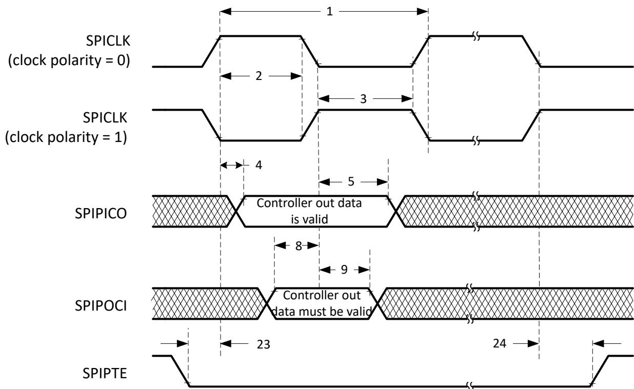
図 6-86. SPI コントローラ・モードの外部タイミング (クロック位相 = 0)
