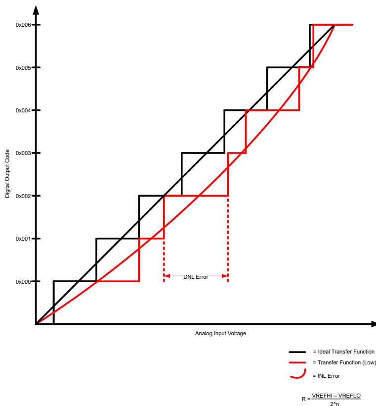
図 6-38. ADC の INL と DNL
