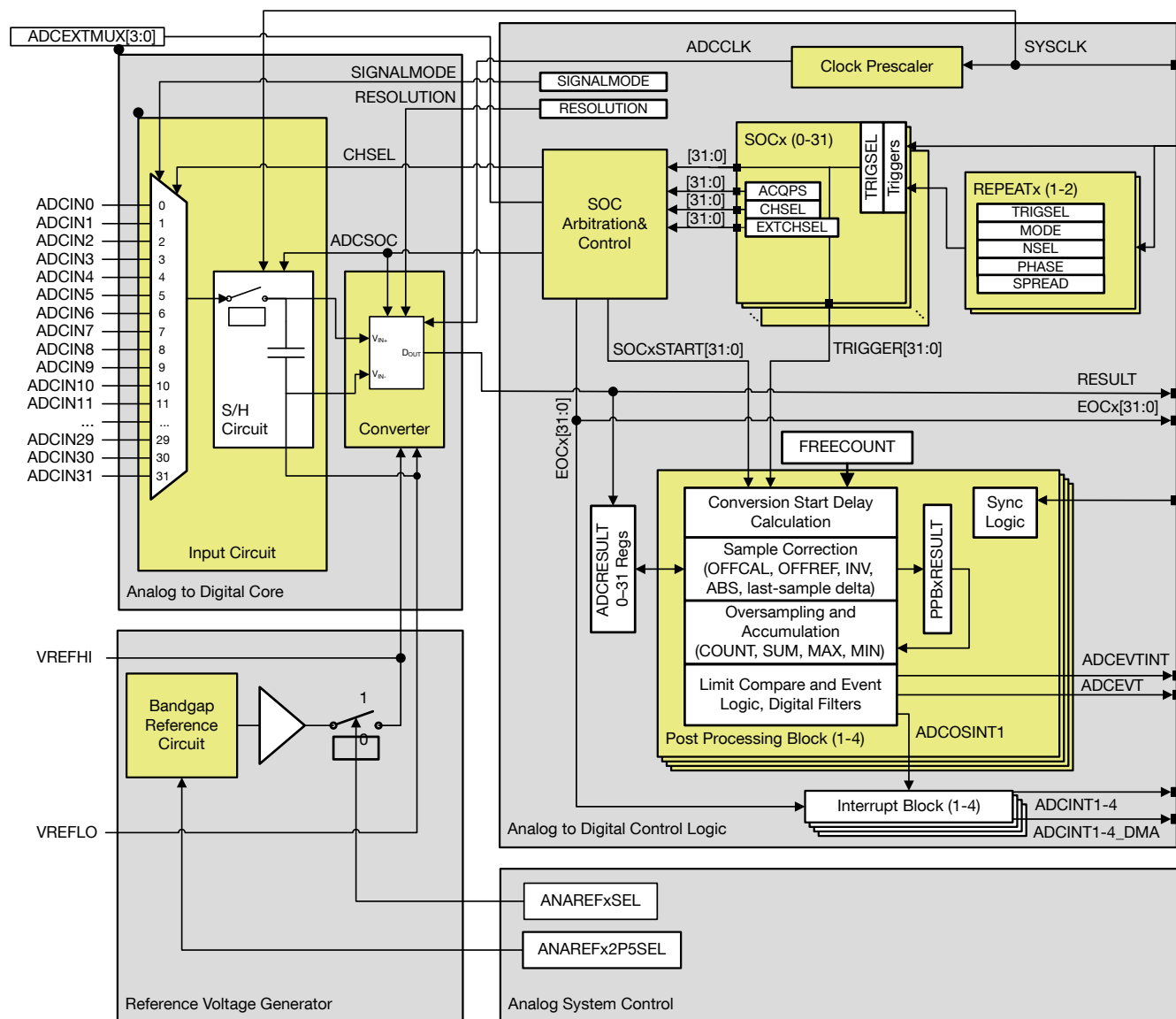
図 6-35. ADC モジュールのブロック図
