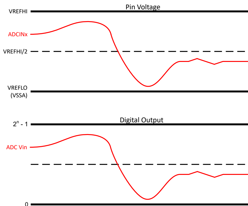
図 6-37. シングルエンド信号モード
