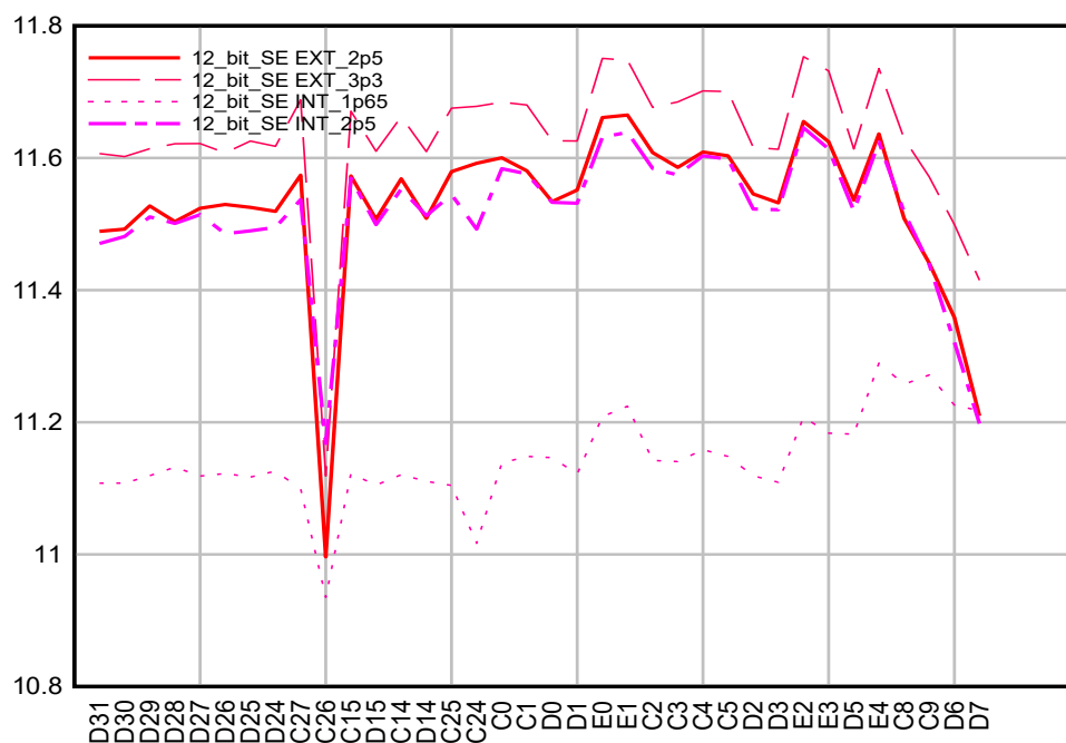
図 6-42. 144 ピン RFS のチャンネルあたりの ENOB – ADC チャンネル C、D、および B
