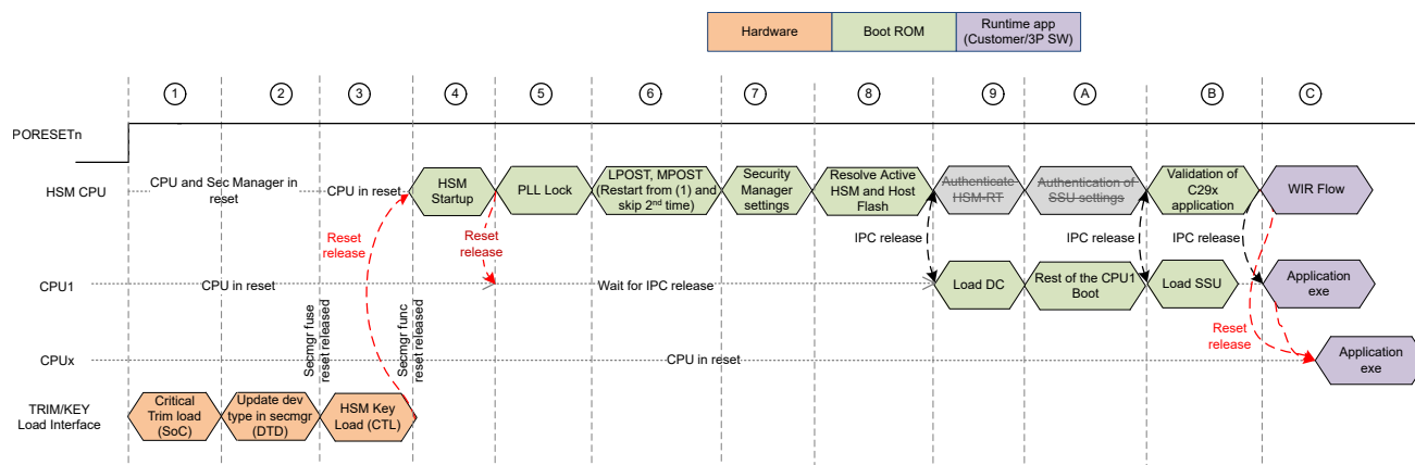
図 7-6. HS-FS デバイスのブートフロー図
