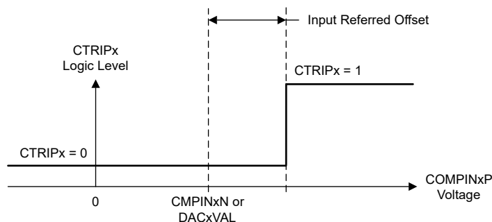
図 6-56. CMPSS コンパレータの入力換算オフセット
