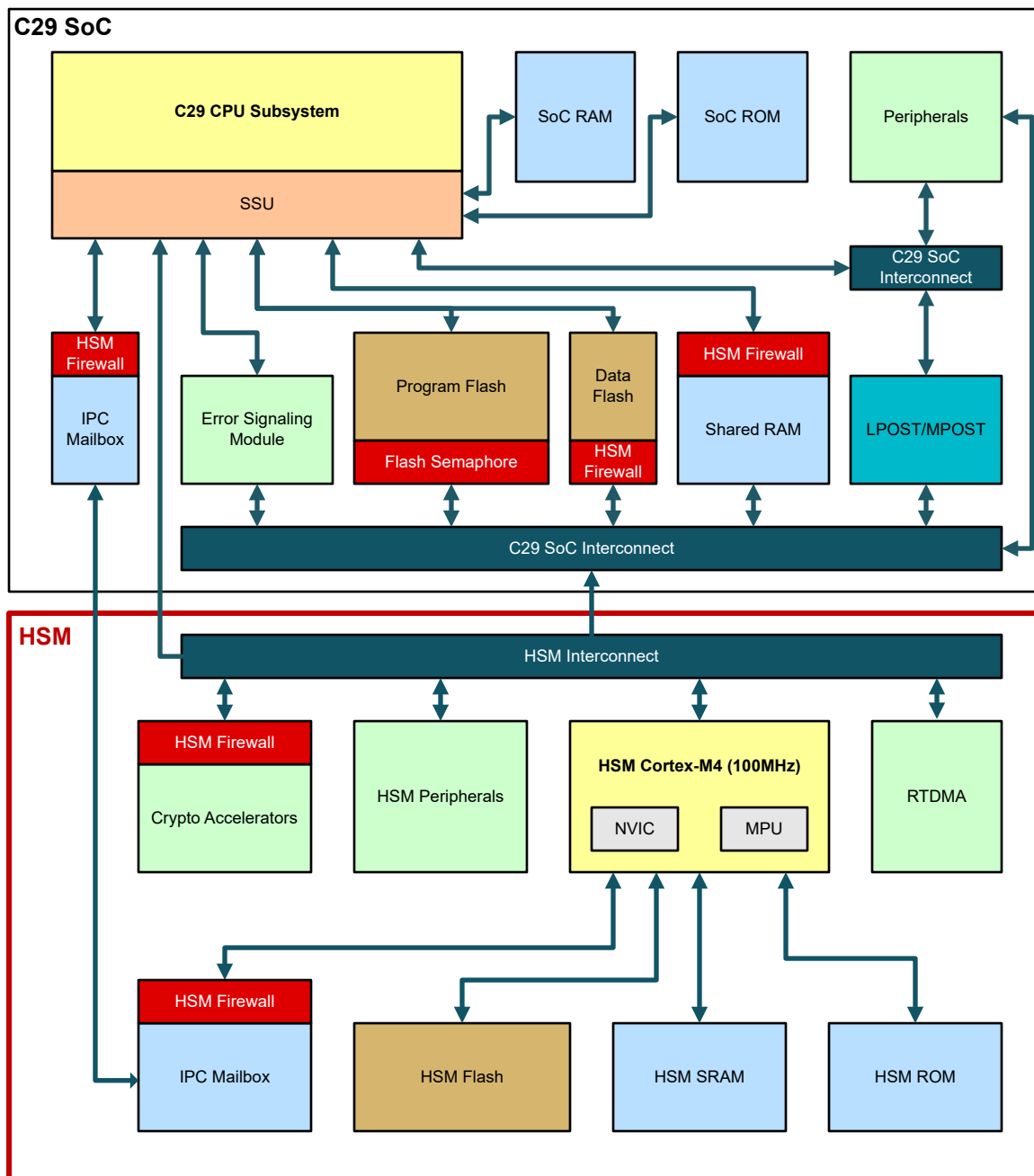
図 7-12. デバイスの概略ブロック図
