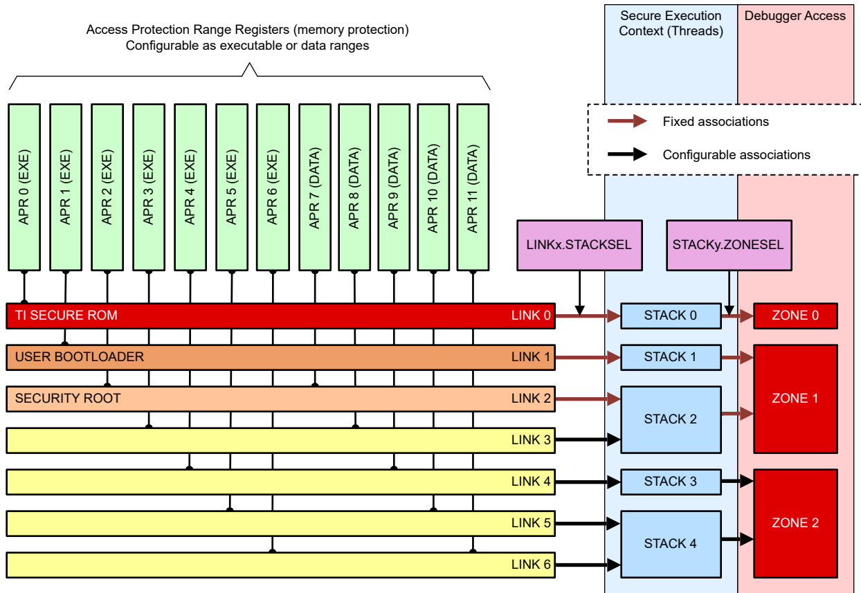
図 7-14. SSU 概念図 (概略版)
