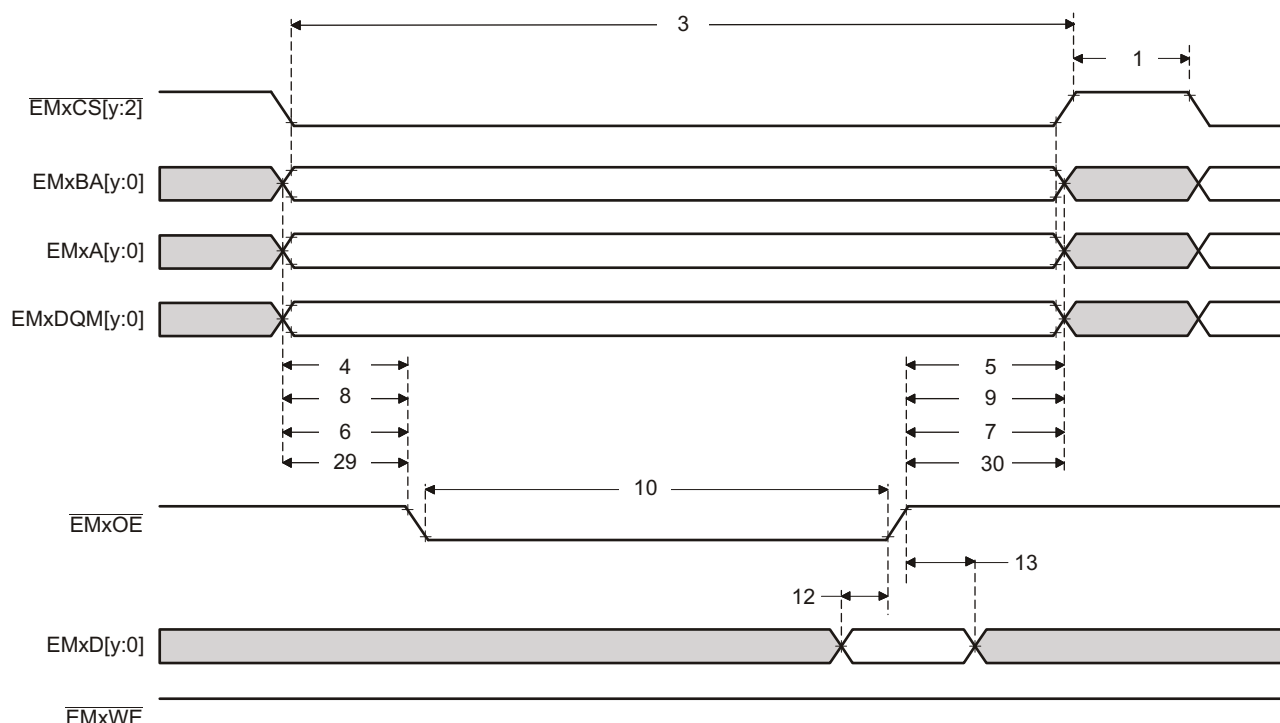
図 6-28. 非同期メモリ読み取りタイミング
