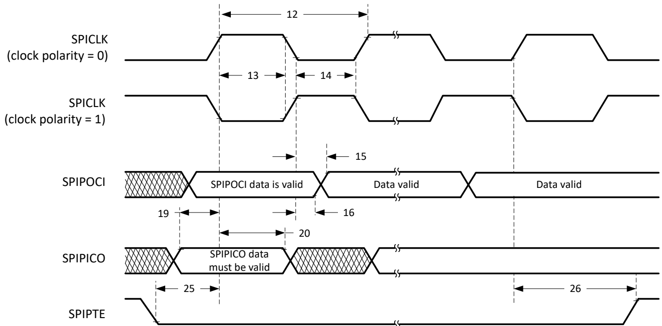
図 6-89. SPI ペリフェラル・モードの外部タイミング (クロック位相 = 1)
