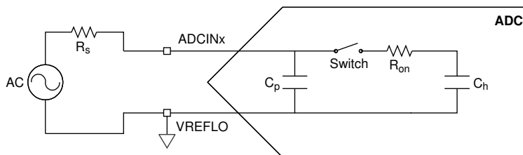
図 6-47. シングルエンド入力モデル
