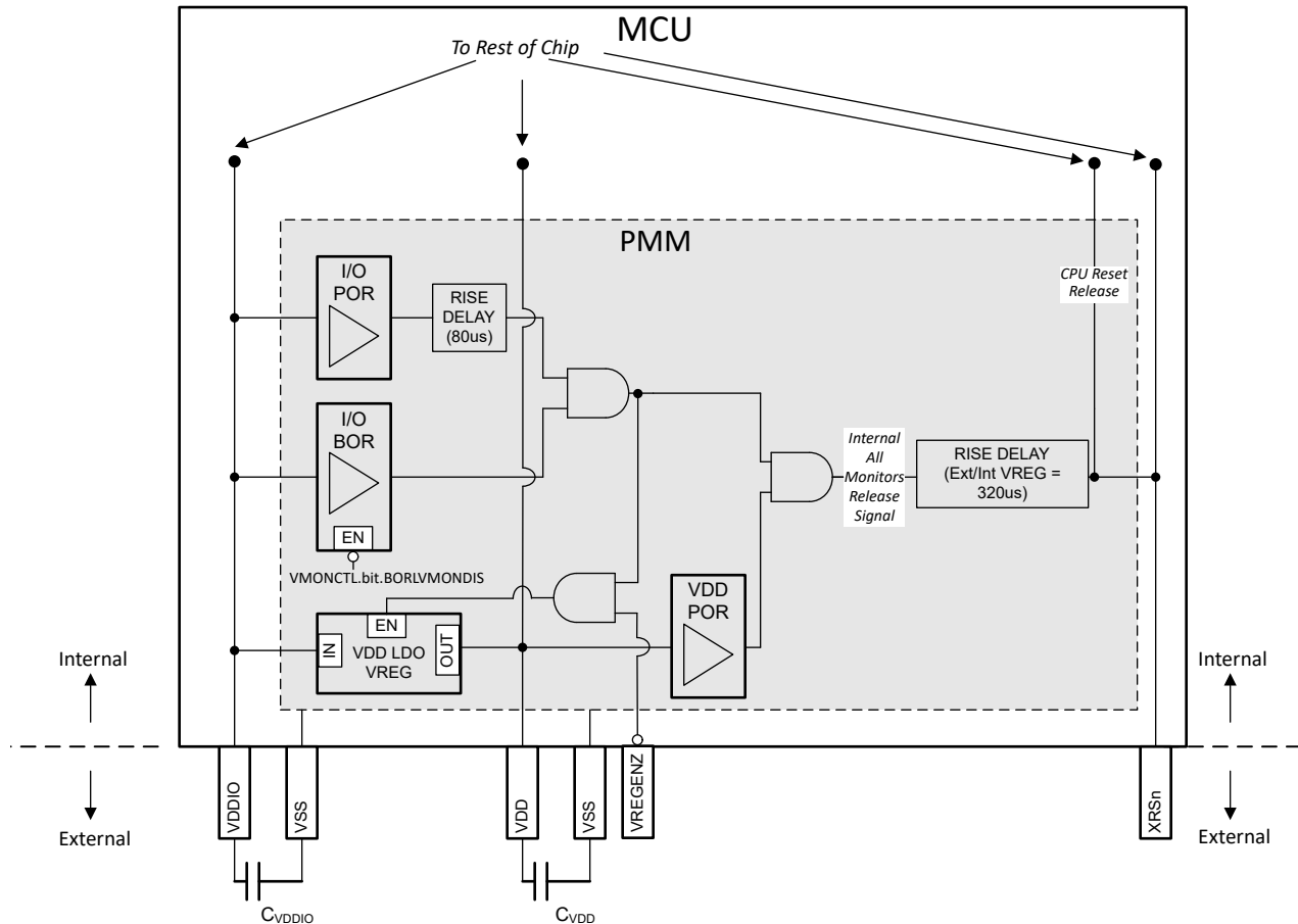
図 6-2. PMM のブロック図
