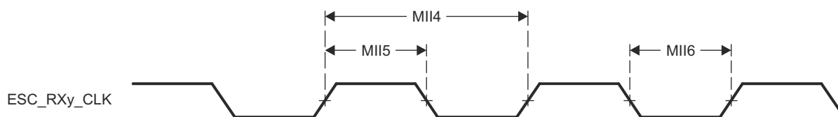
図 6-94. EtherCAT 受信クロックのタイミング (MII 動作)
