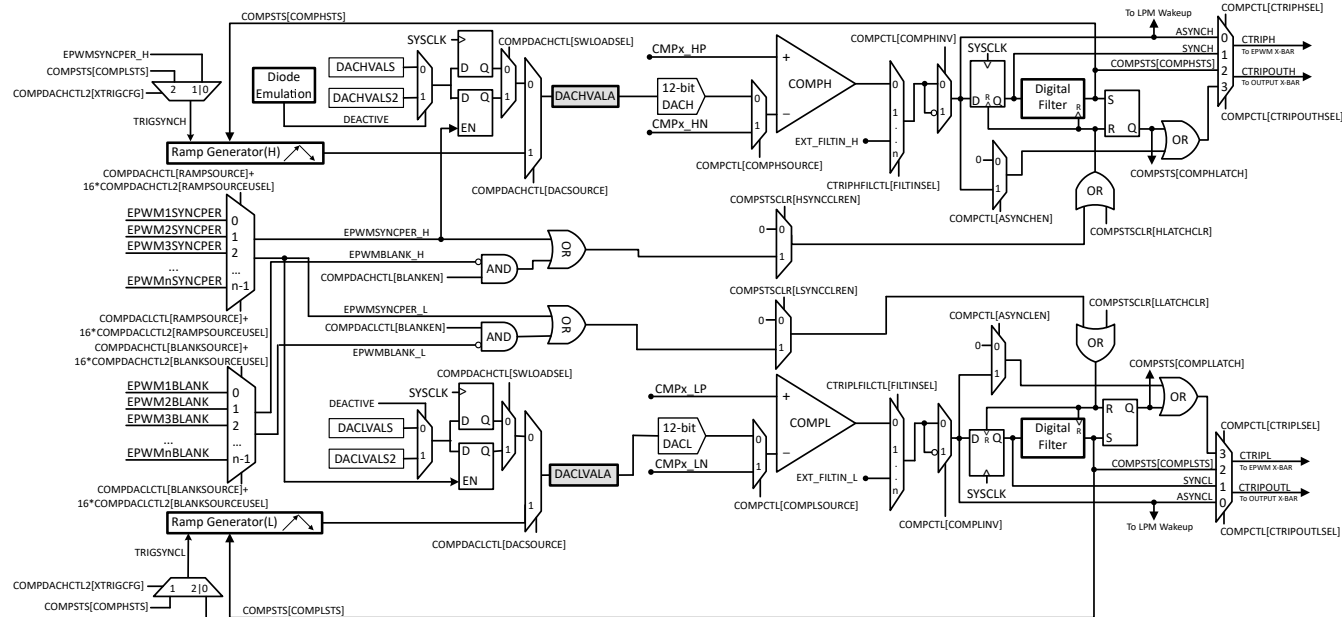
図 6-54. CMPSS モジュールのブロック図
