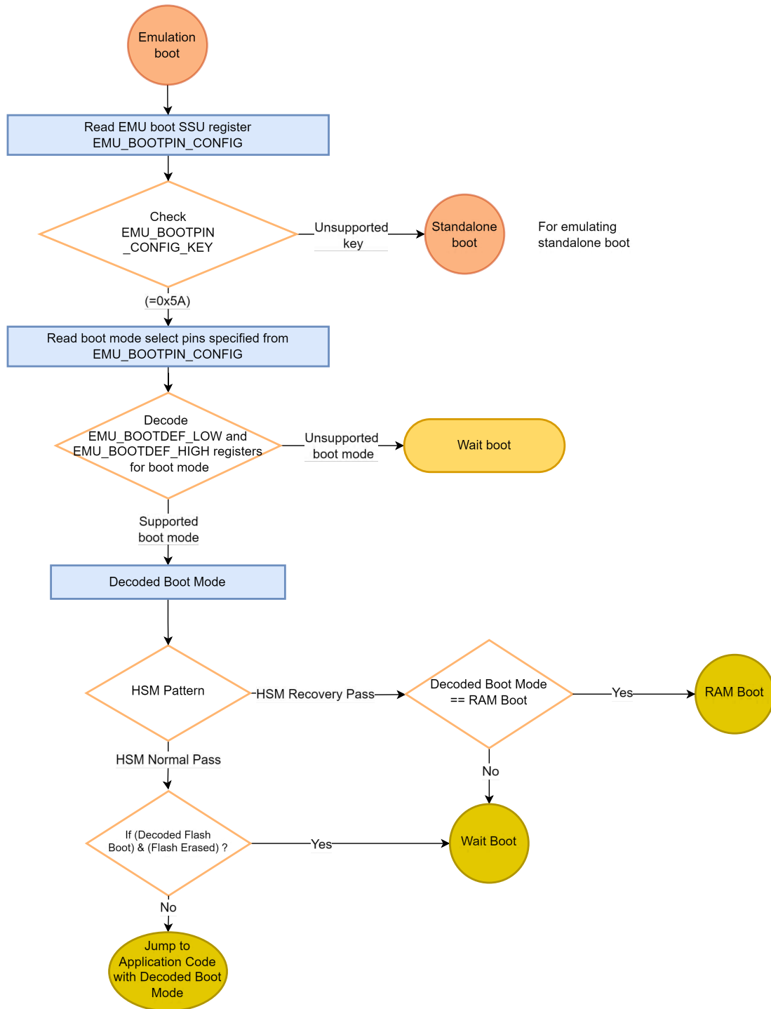
図 7-10. エミュレーション ブート フロー
