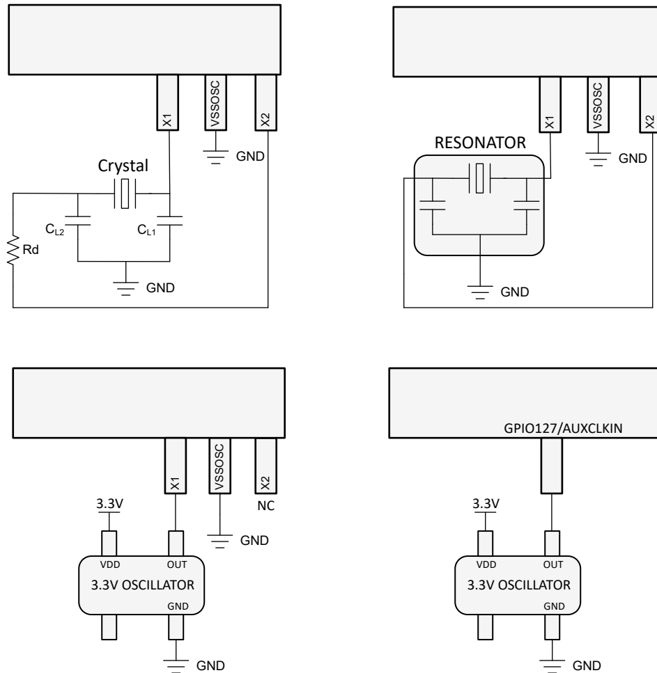
図 6-11. 入力クロックの F29H85x、F29P58x および F29P32x デバイスへの接続
