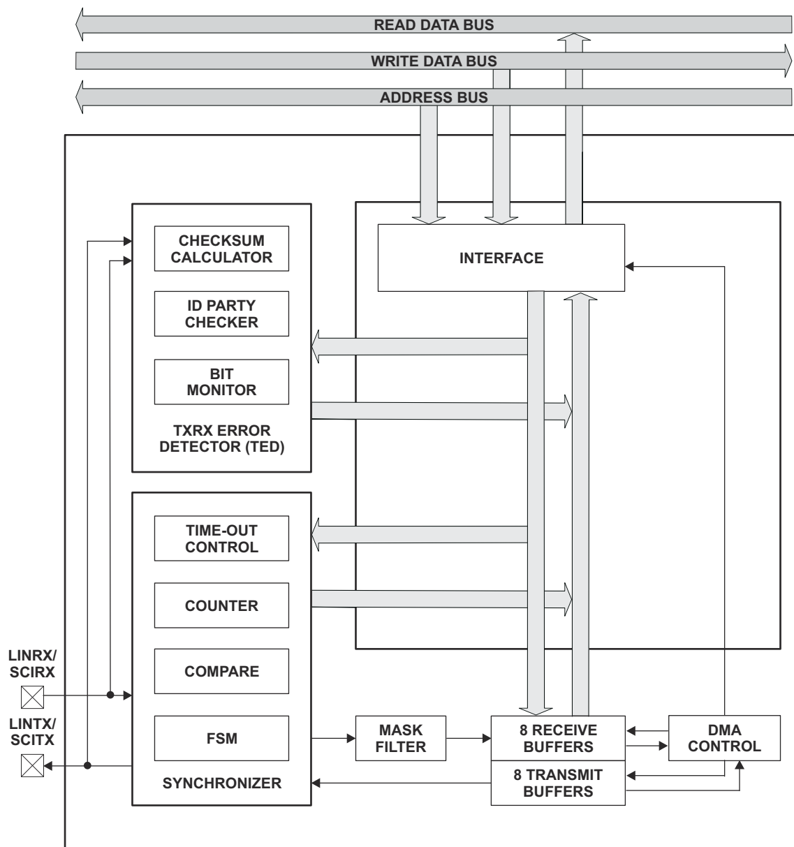
図 6-90. LIN のブロック図
