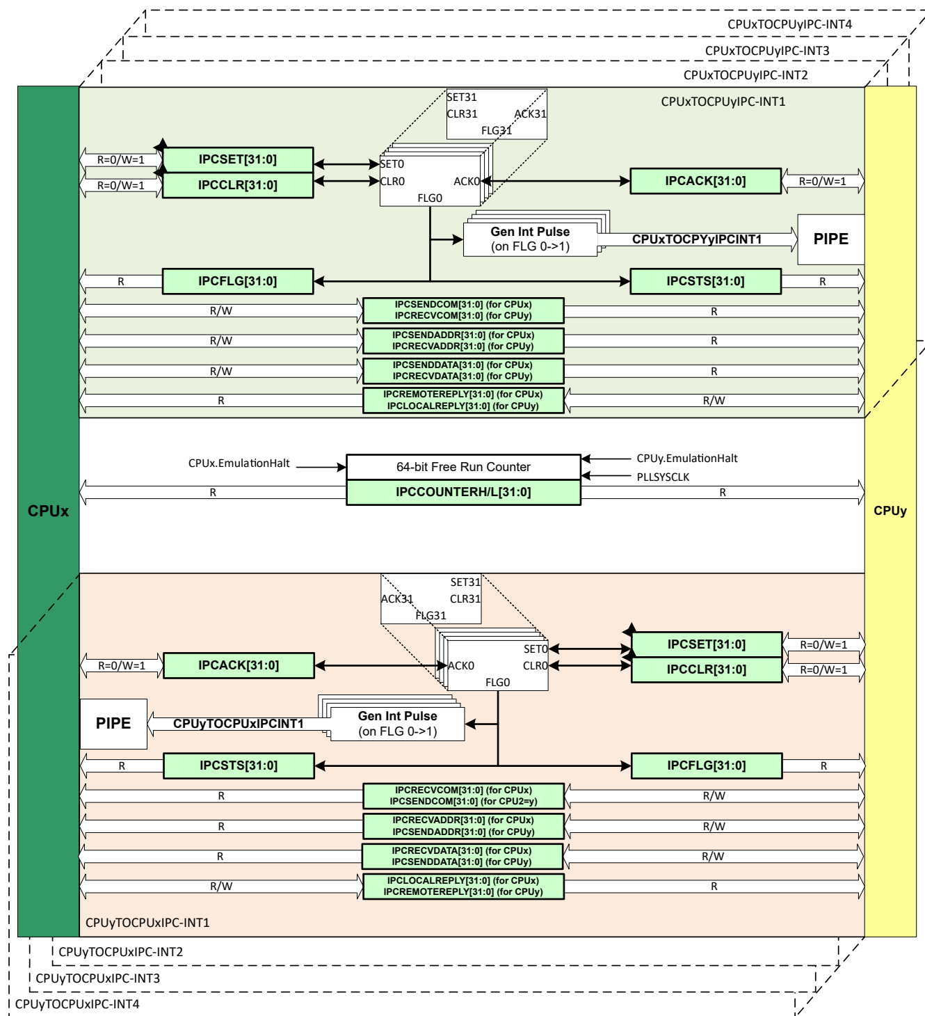
図 7-20. IPC モジュール アーキテクチャ
