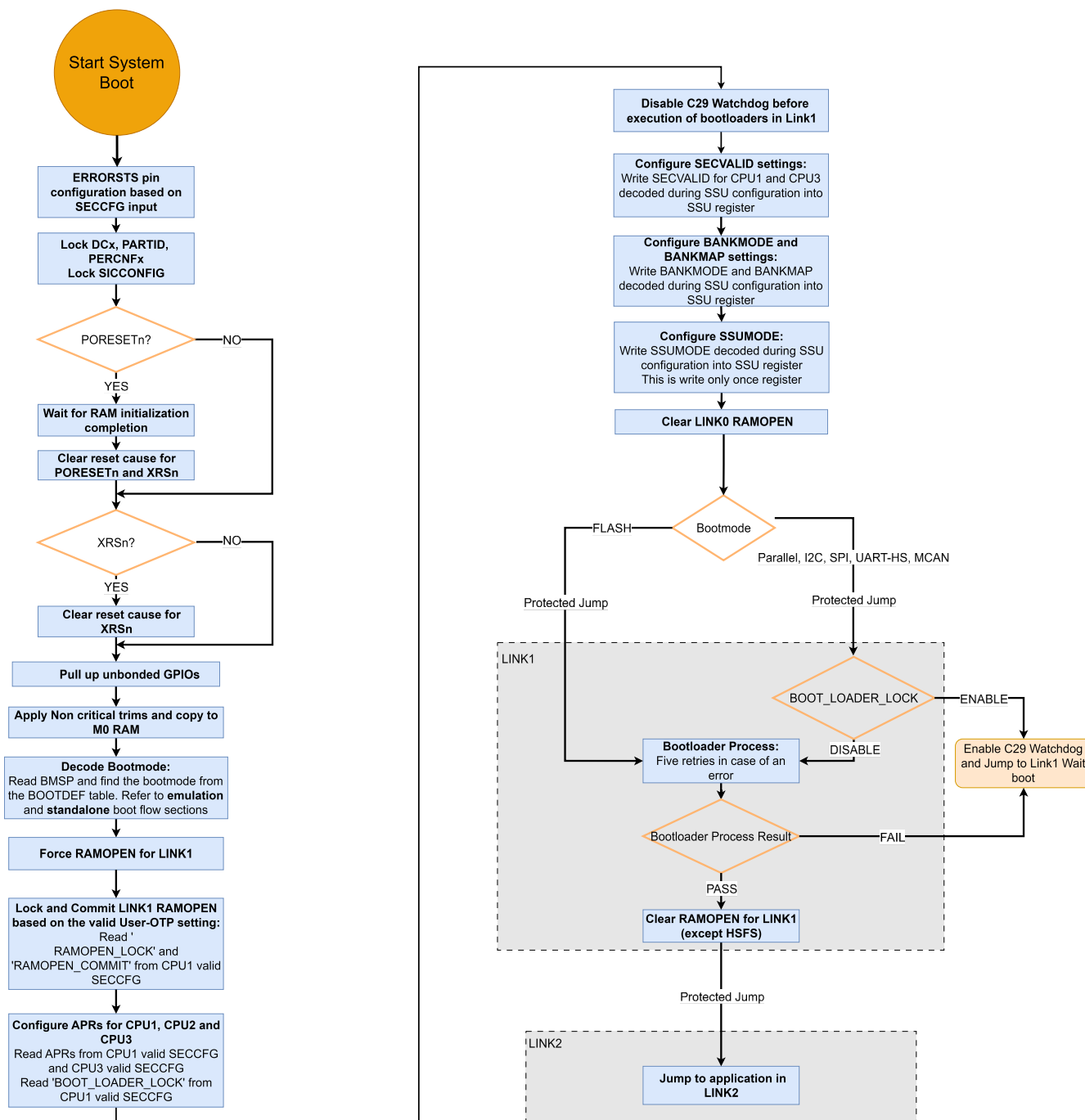
図 7-9. アプリケーション コードまでのシステム ブート フロー
