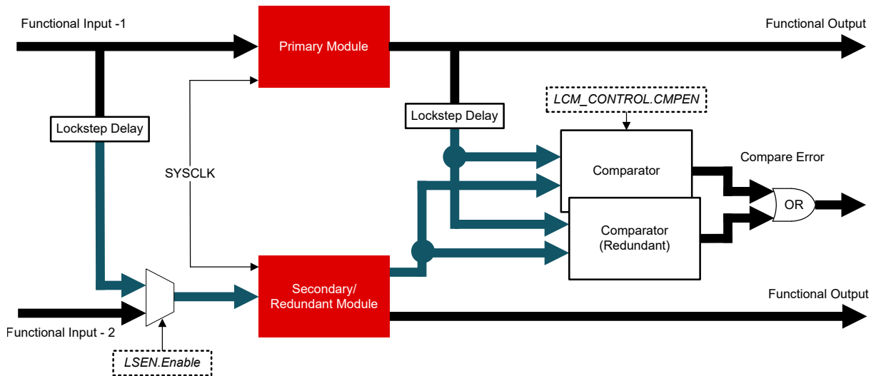
図 7-23. LCM のブロック図
