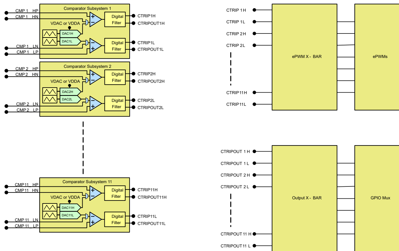
図 6-53. CMPSS の接続
