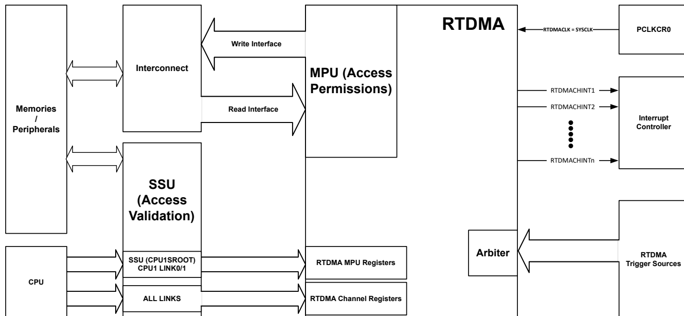
図 6-23. RTDMA のブロック図
