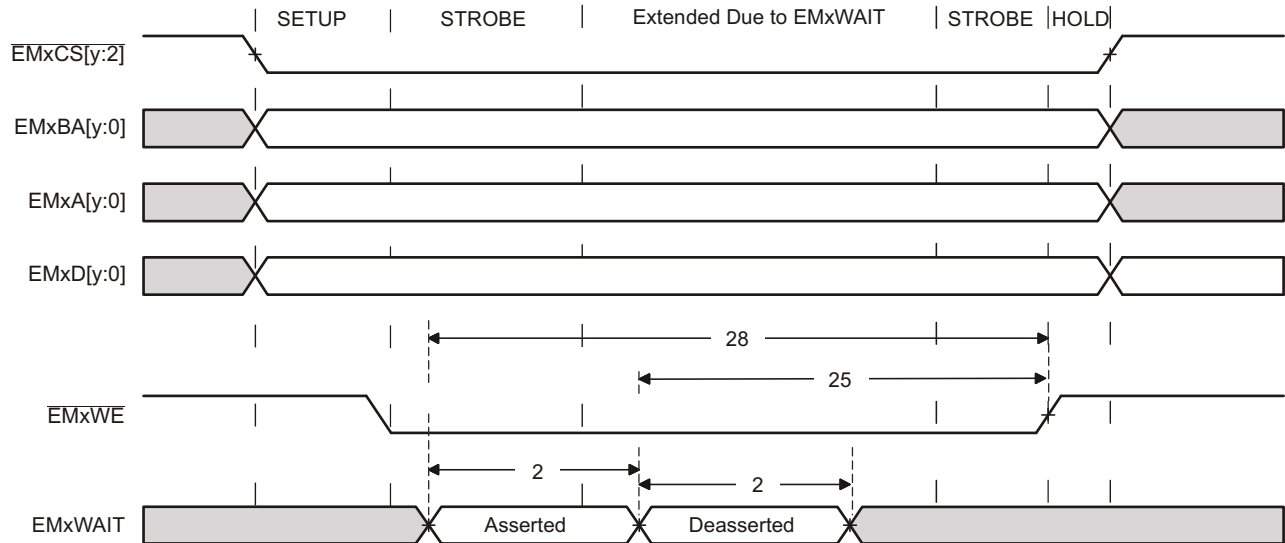
図 6-31. EMxWAIT 書き込みタイミング要件
