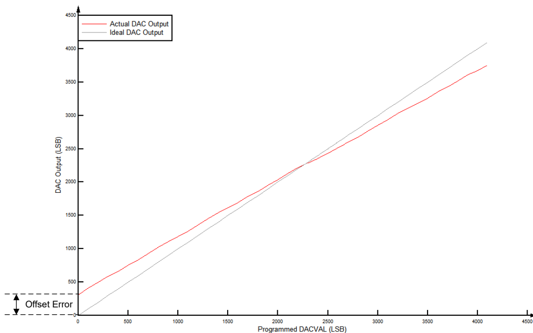
図 6-58. CMPSS DAC の静的オフセット
