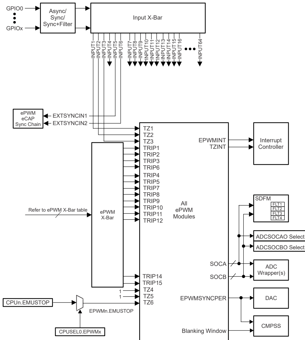
図 6-67. ePWM トリップ入力の接続
