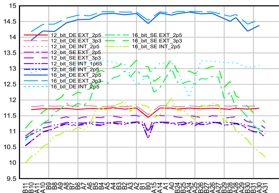
図 6-43. 176 ピン PTS のチャンネルあたりの ENOB – ADC チャンネル A および B
