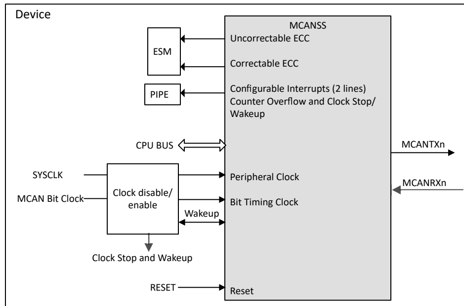
図 6-74. MCAN モジュールの概要
