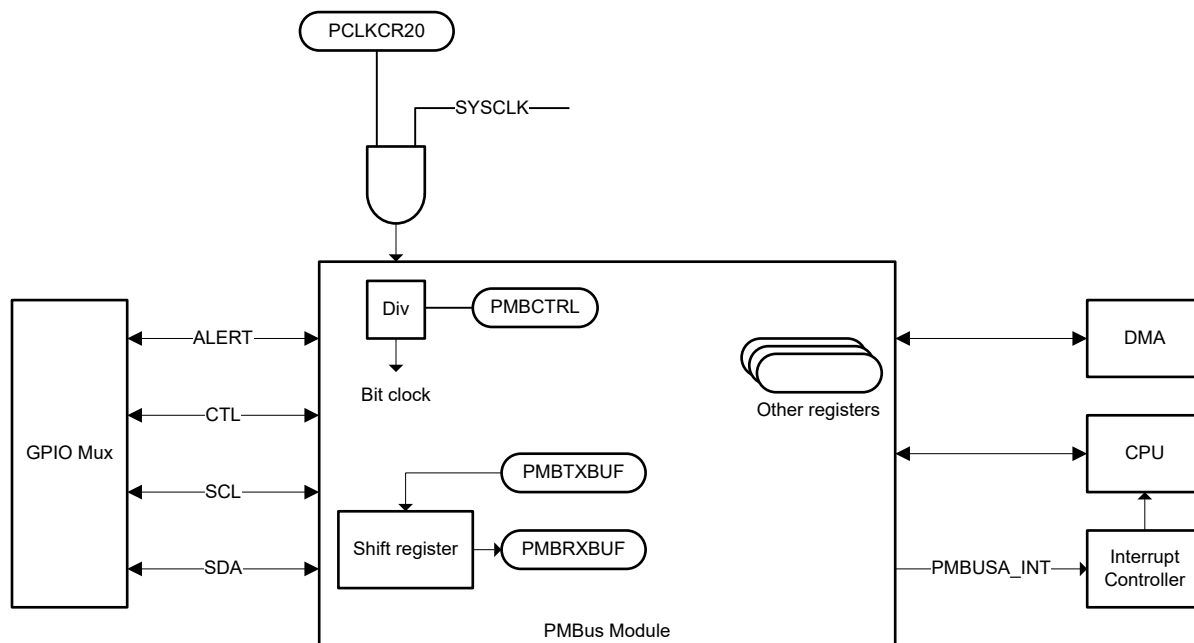
図 6-84. PMBus のブロック図
