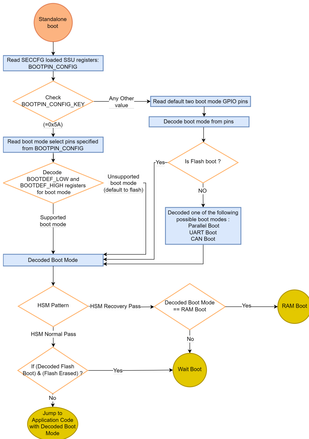
図 7-11. スタンドアロン ブートフロー
