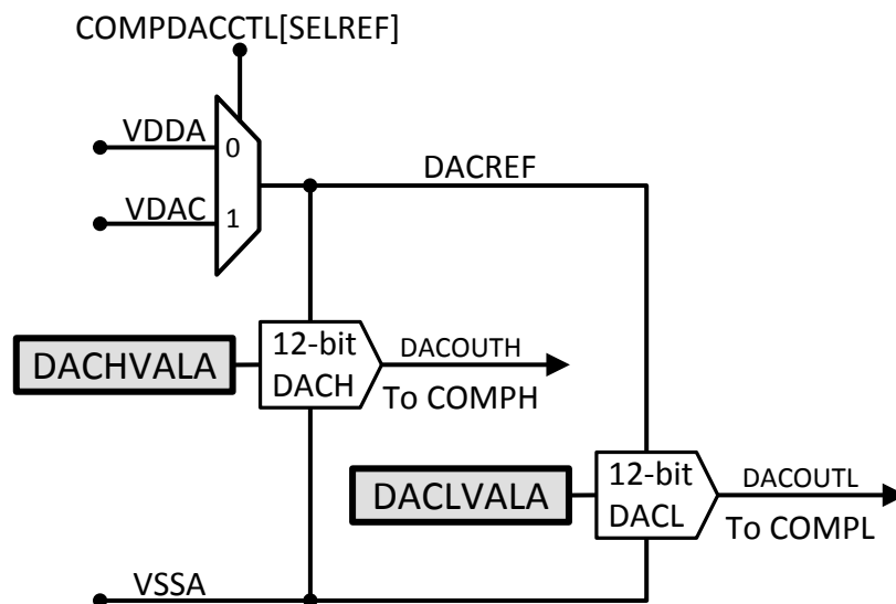
図 6-55. リファレンス DAC のブロック図
