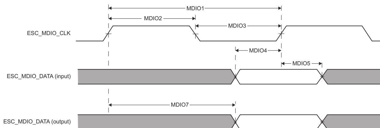
図 6-96. EtherCAT MDIO のタイミング図
