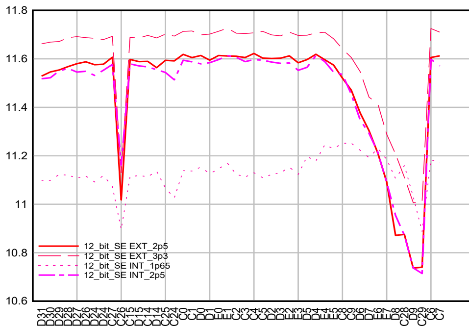
図 6-44. 176 ピン PTS のチャンネルあたりの ENOB – ADC チャンネル C、D、および B
