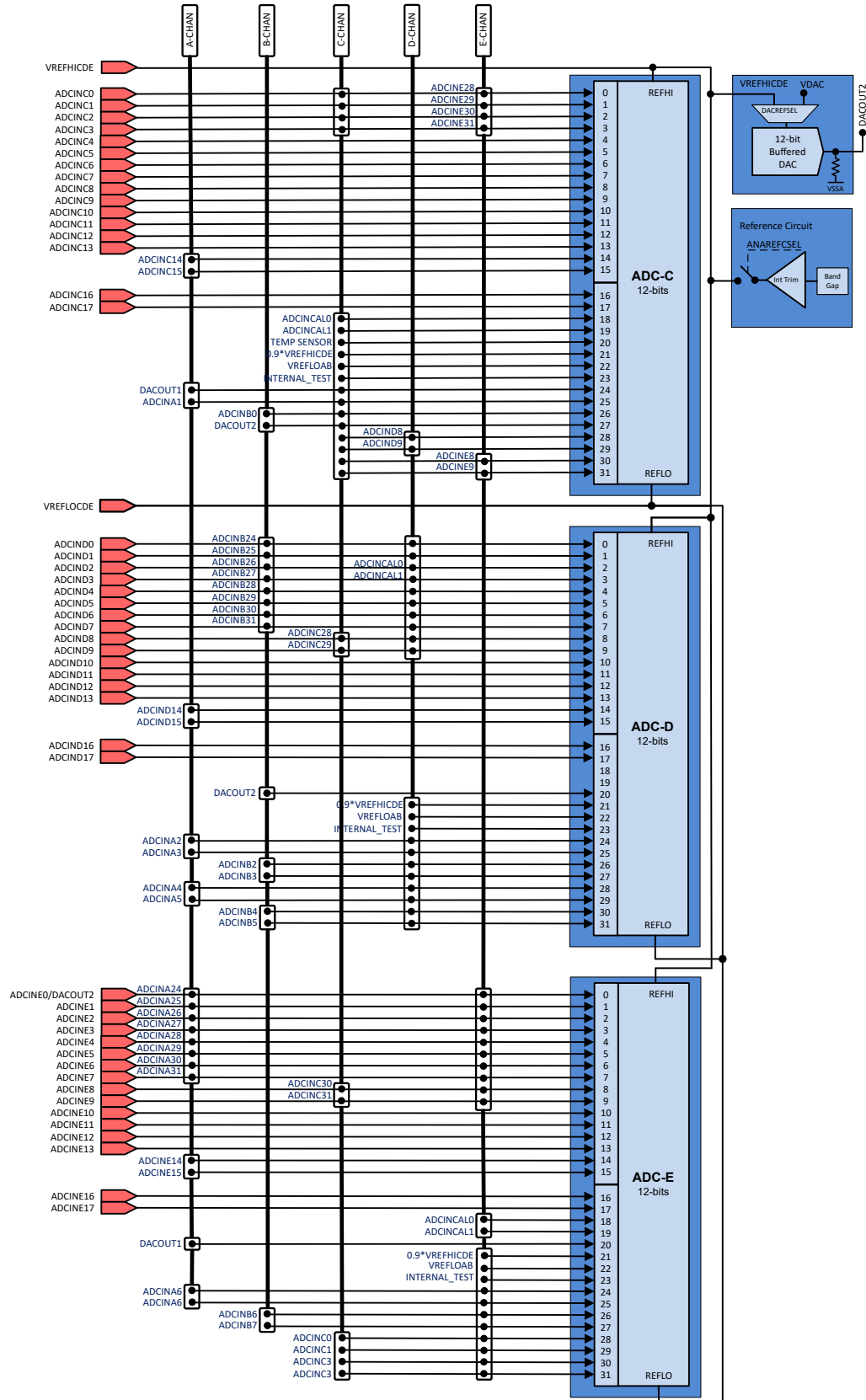
図 6-33. アナログ サブシステムのブロック図 (ADC C、ADC D、ADC E)
