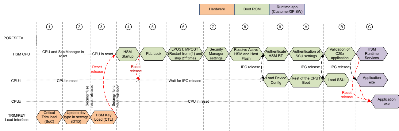
図 7-7. HS-SE のセキュア ブートフロー図
