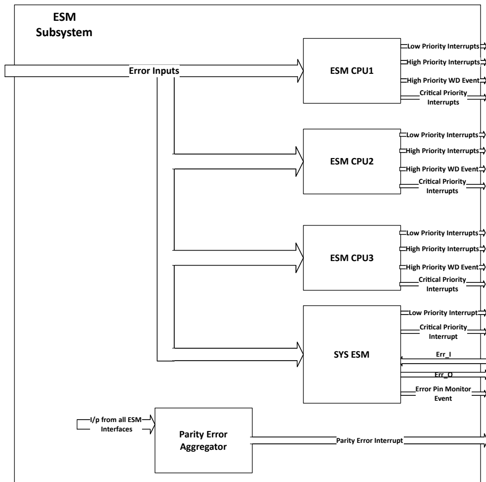
図 7-3. ESM-SS のブロック図
