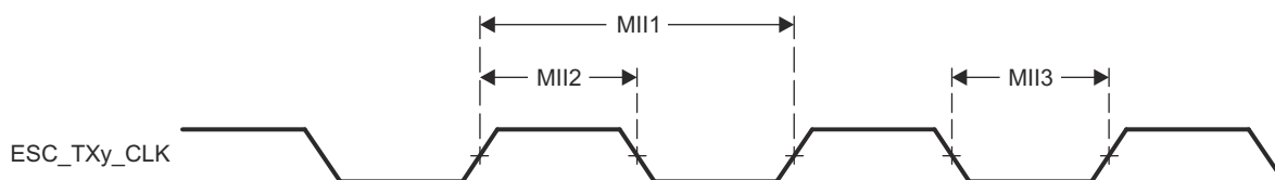
図 6-92. EtherCAT 送信クロックのタイミング (MII 動作)
