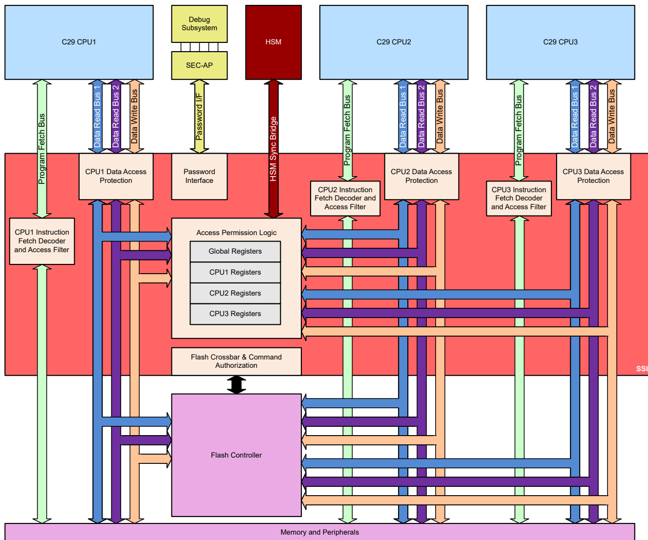
図 7-13. C29 リアルタイム セキュリティ アーキテクチャのブロック図
