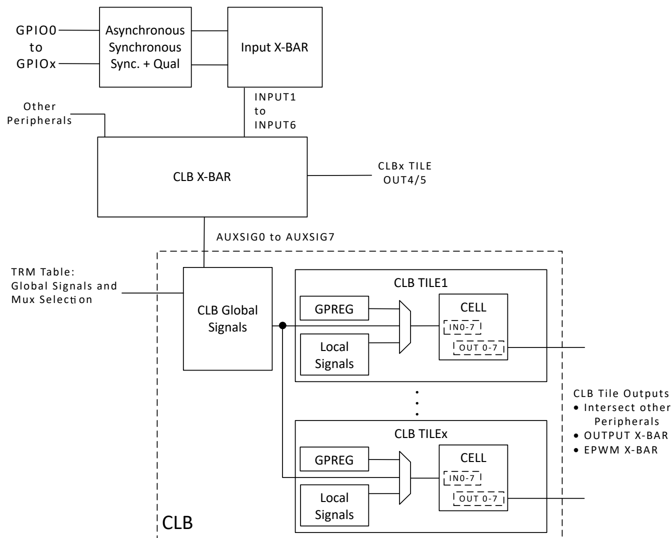
図 7-22. GPIO から CLB へのタイル接続
