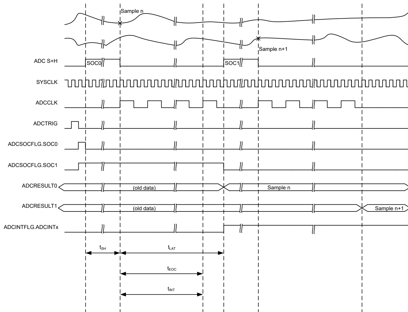
図 6-52. 16 ビット モードの Late 割り込みモードでの ADC タイミング (SYSCLK サイクル)
