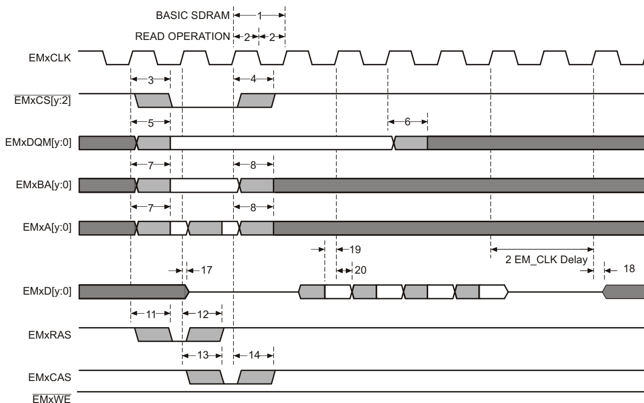
図 6-26. 基本的な SDRAM 読み取り動作
