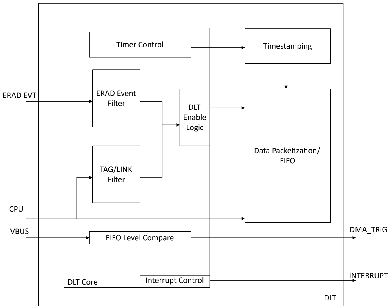
図 7-17. DLT のブロック図
