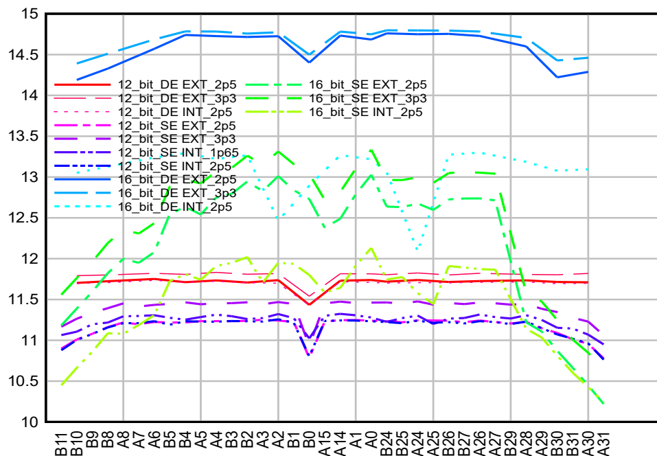
図 6-41. 144 ピン RFS のチャンネルあたりの ENOB – ADC チャンネル A および B
