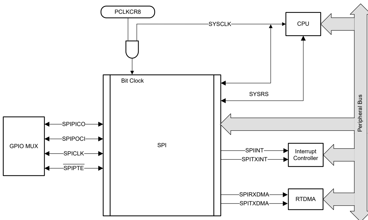
図 6-85. SPI CPU インターフェイス
