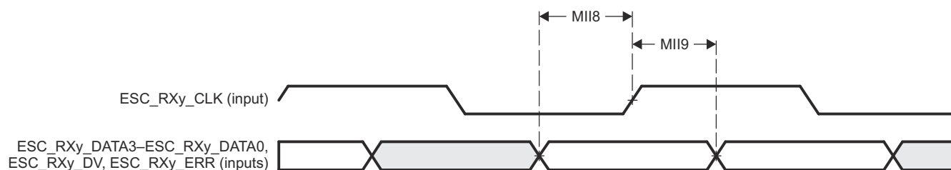
図 6-95. EtherCAT 受信インターフェースのタイミング (MII 動作)
