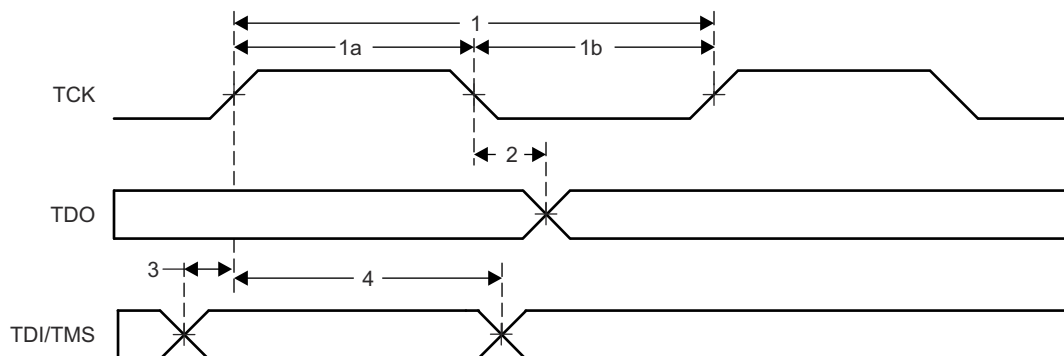
図 6-18. JTAG のタイミング
