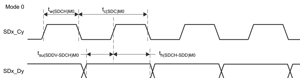
図 6-73. SDFM タイミング図 - モード 0
