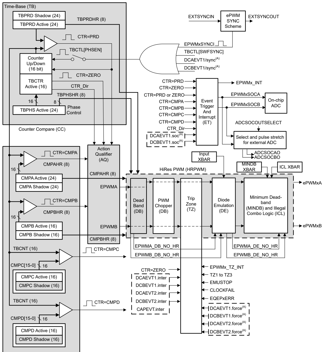
図 6-66. ePWM サブモジュールおよび重要な内部信号の相互接続
