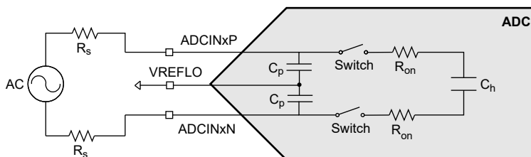
図 6-48. 差動入力モデル
