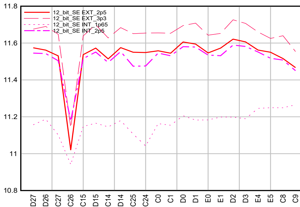
図 6-40. 100 ピン PZS のチャンネルあたりの ENOB – ADC チャンネル C、D、および B
