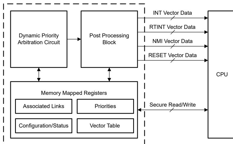
図 7-15. PIPE アーキテクチャ
