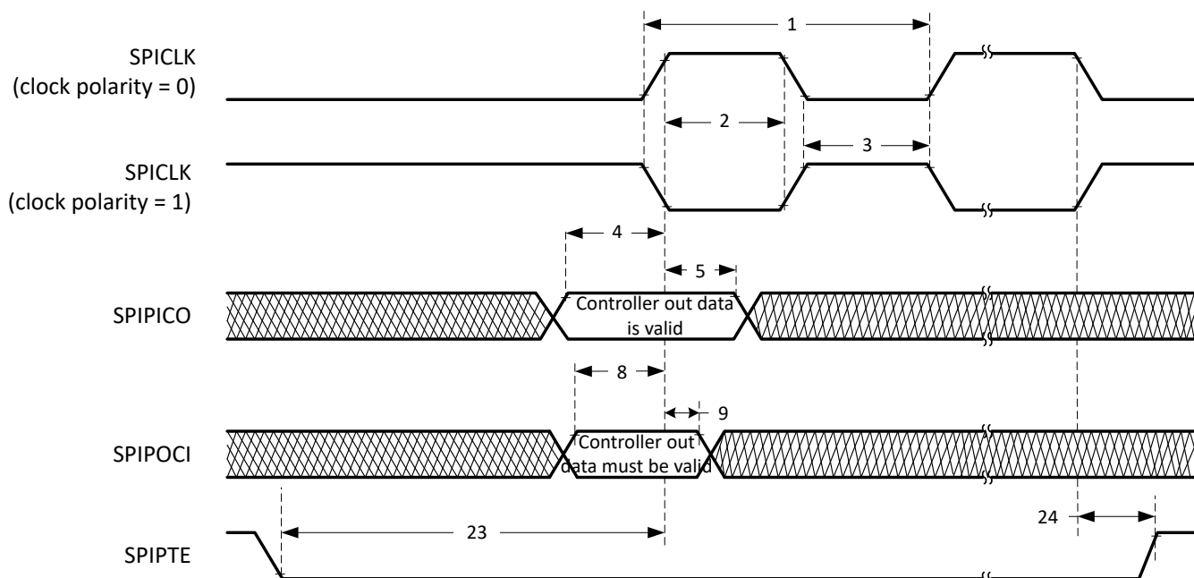
図 6-86. SPI コントローラ・モードの外部タイミング (クロック位相 = 0)
