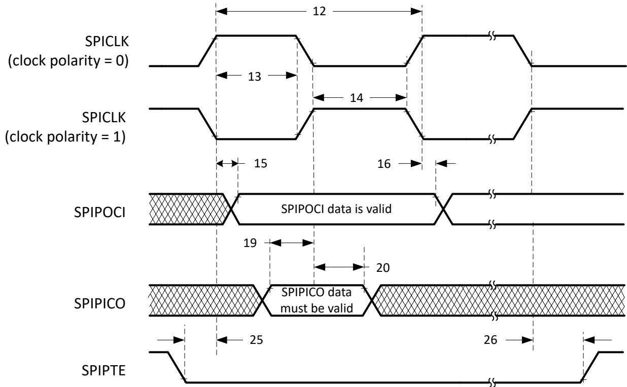
図 6-88. SPI ペリフェラル・モードの外部タイミング (クロック位相 = 0)
