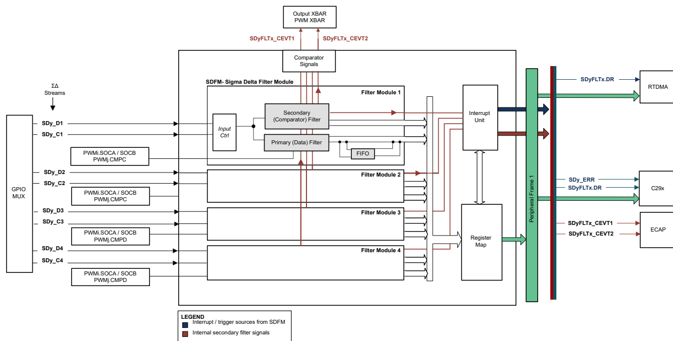
図 6-72. シグマ デルタ フィルタ モジュール (SDFM) のブロック図
