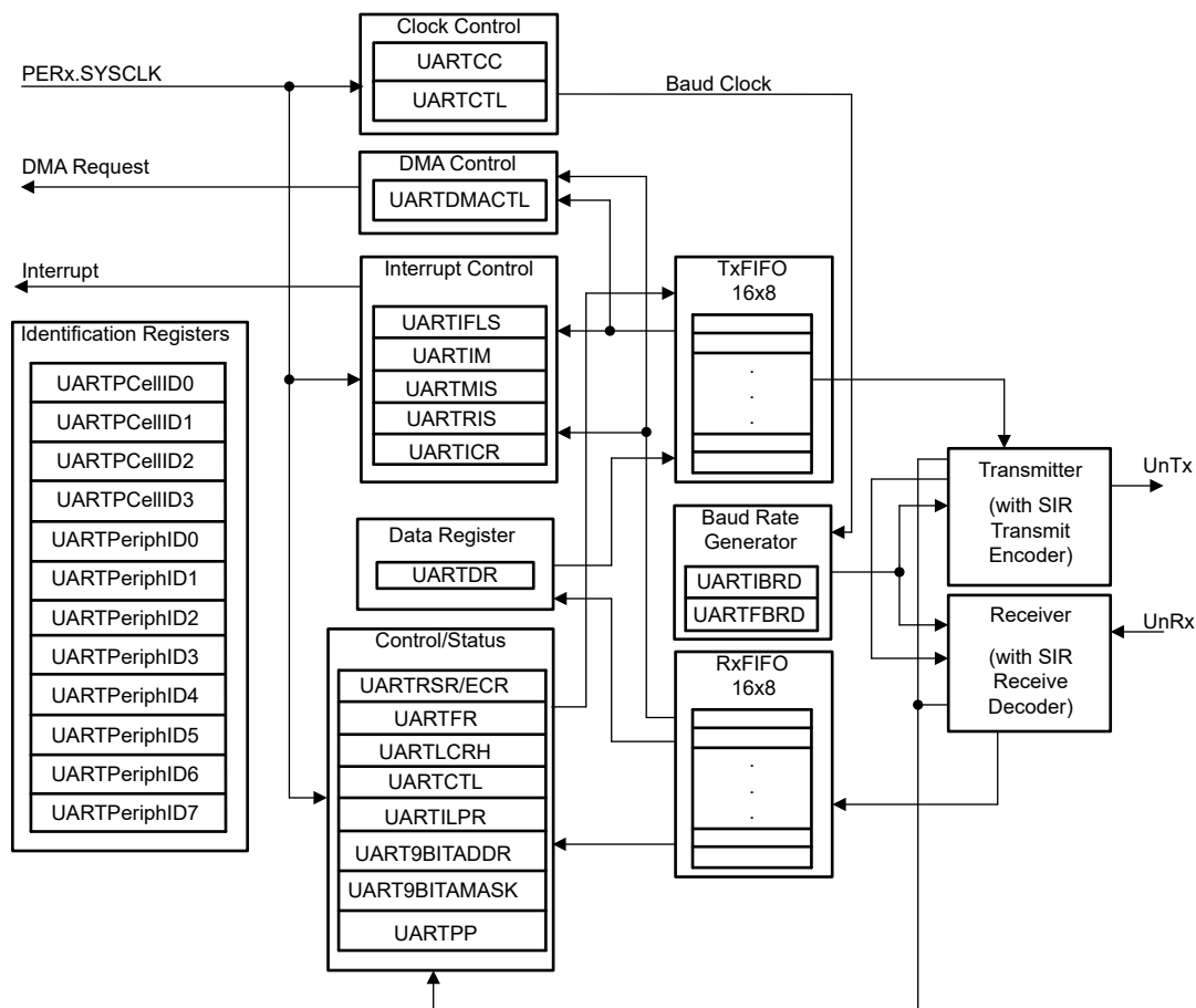
図 6-97. UART モジュールのブロック図
