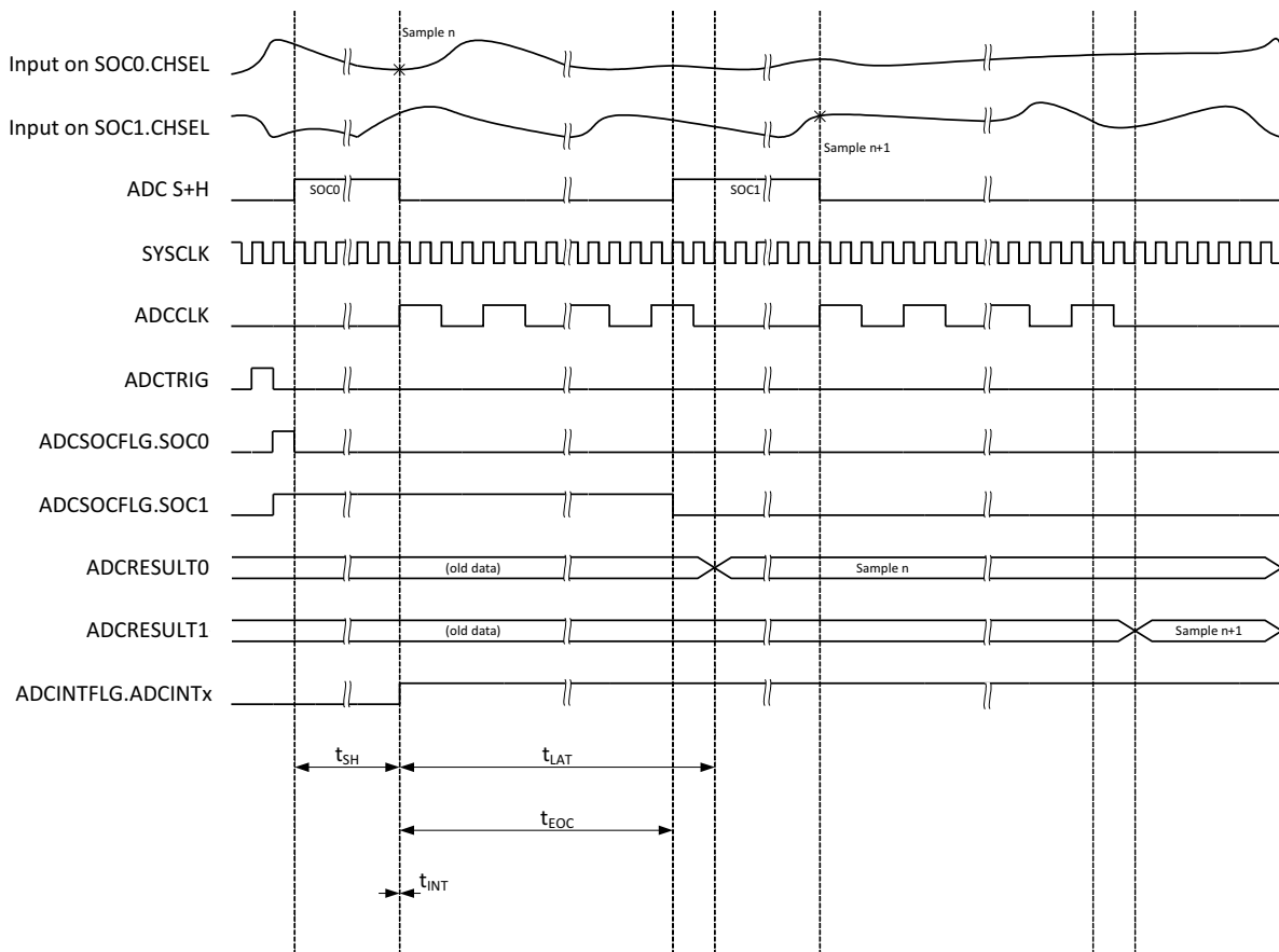
図 6-49. 12 ビット モードの Early 割り込みモードでの ADC タイミング
