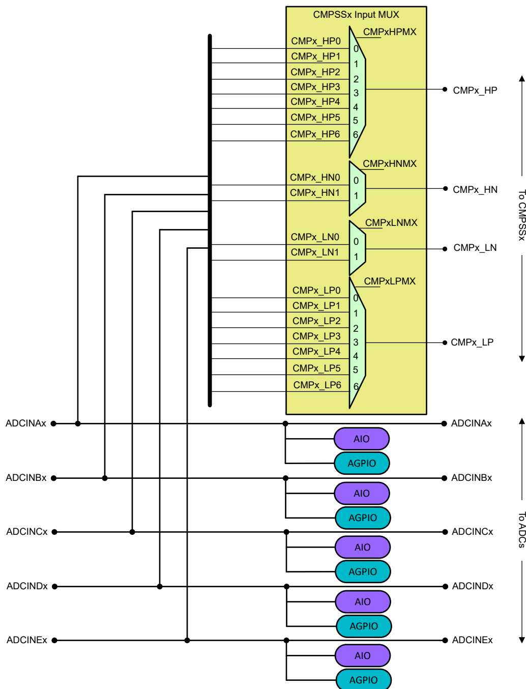
図 6-34. アナログ グループ接続
