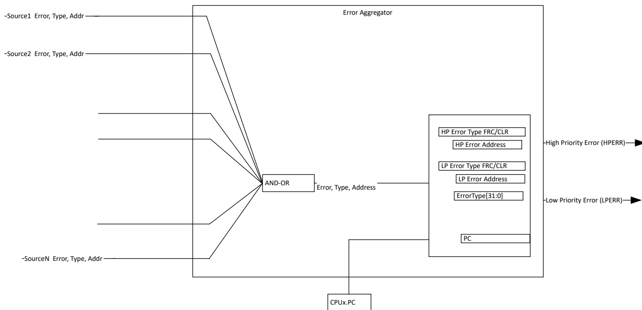
図 7-4. エラー アグリゲータのブロック図
