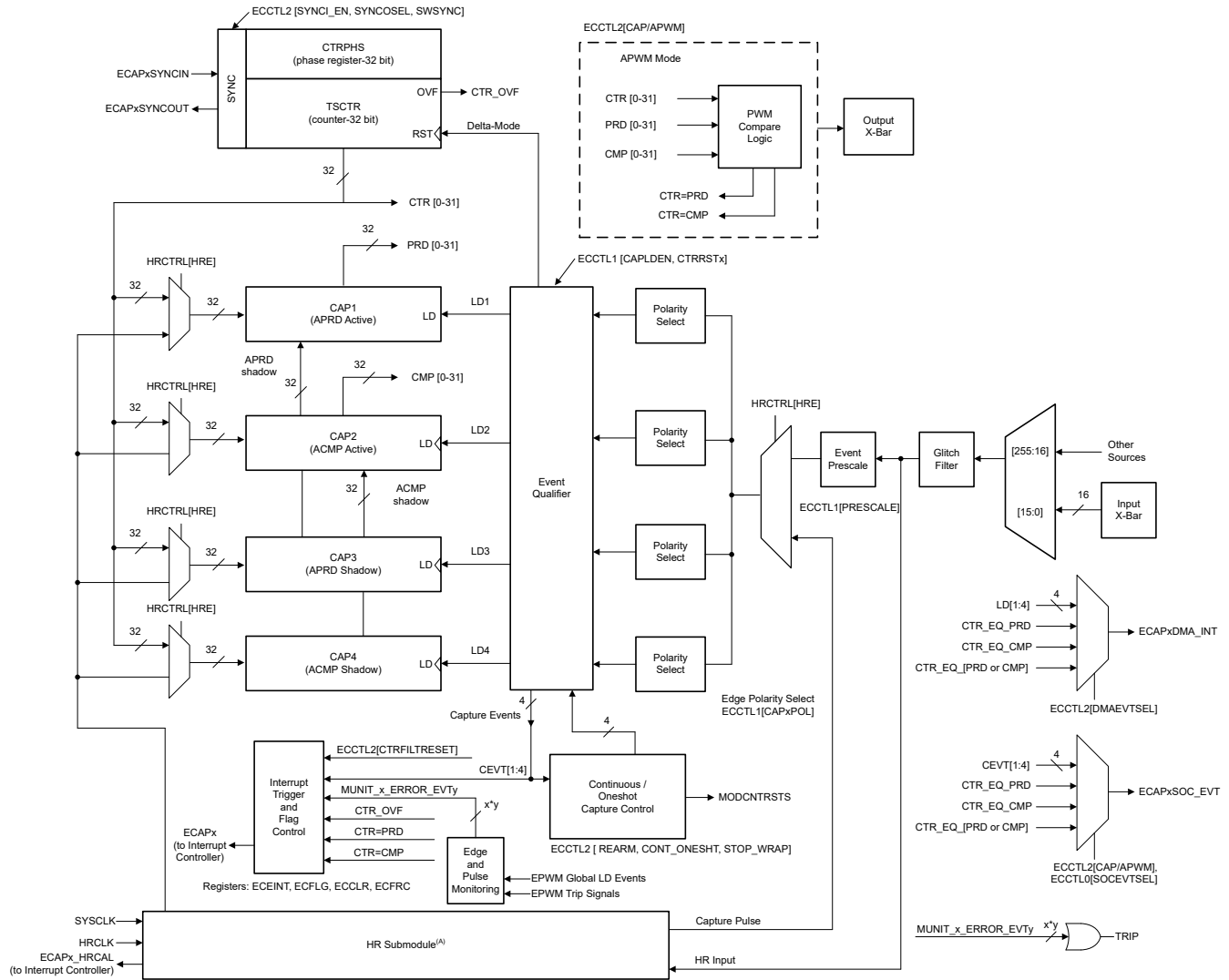
図 6-62. eCAP のブロック図
