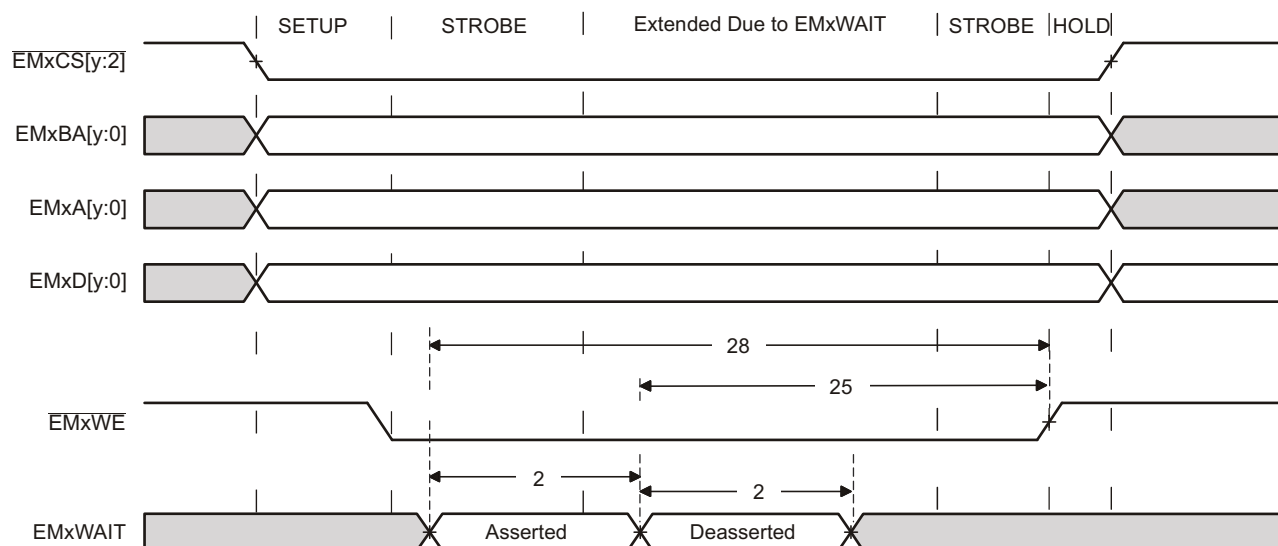
図 6-31. EMxWAIT 書き込みタイミング要件
