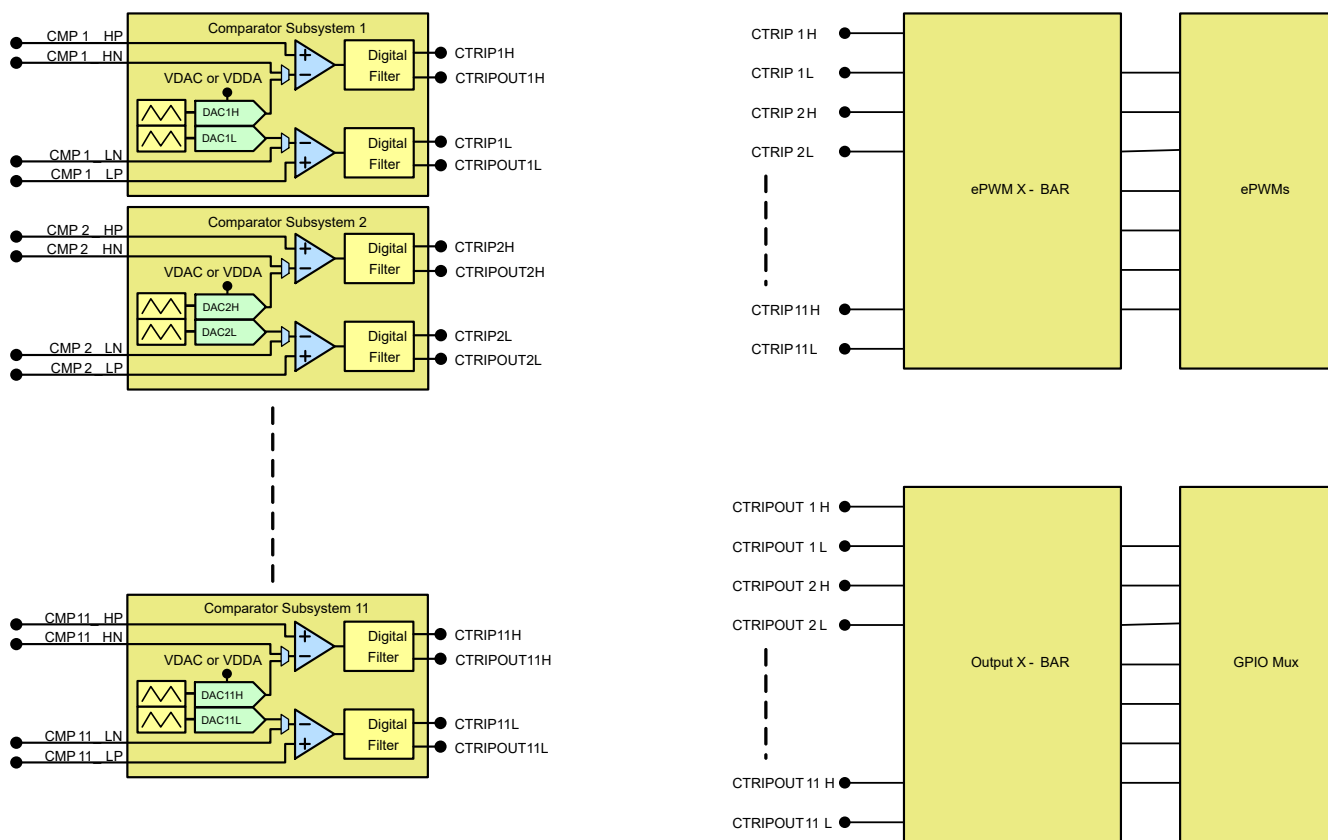
図 6-53. CMPSS の接続
