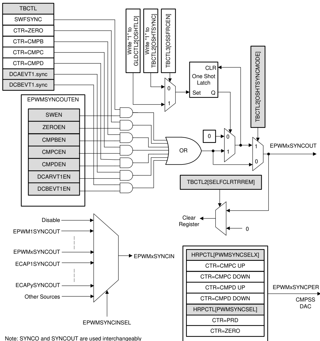
図 6-68. 同期チェーンのアーキテクチャ
