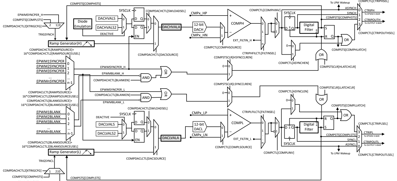
図 6-54. CMPSS モジュールのブロック図
