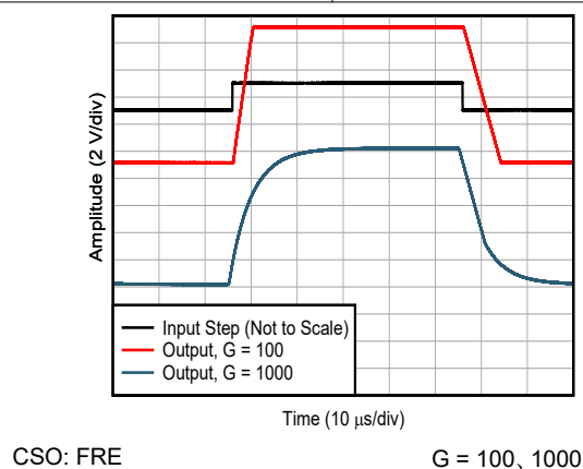
図 6-39. 大信号
