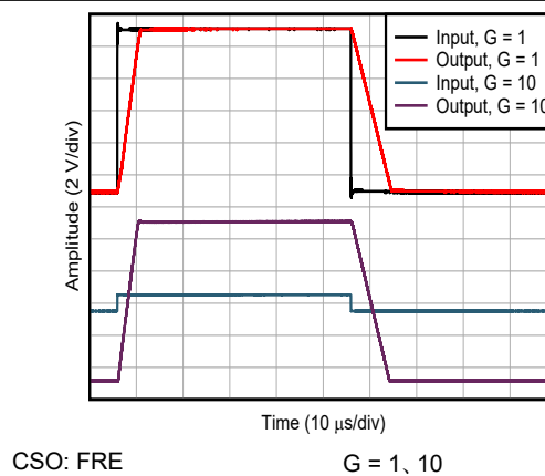
図 6-38. 大信号
