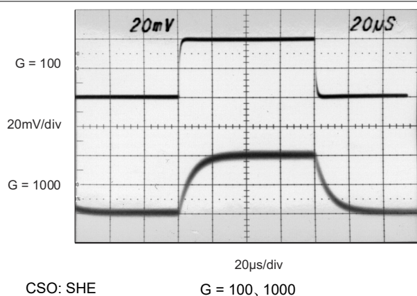
図 6-33. 小信号
