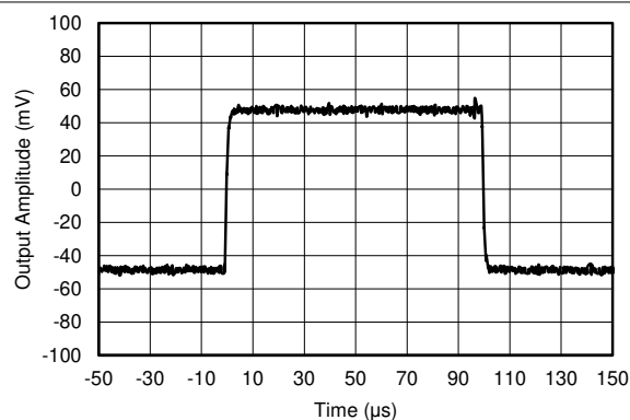
図 6-32. 小信号
