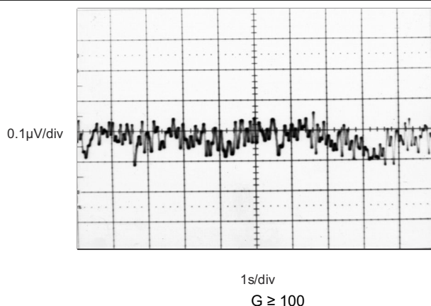
図 6-31. 0.1 ~ 10Hz 入力換算電圧ノイズ
