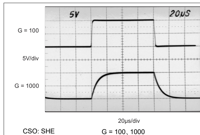
図 6-37. 大信号
