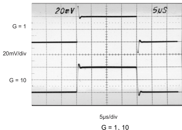
図 8-4. 小信号
