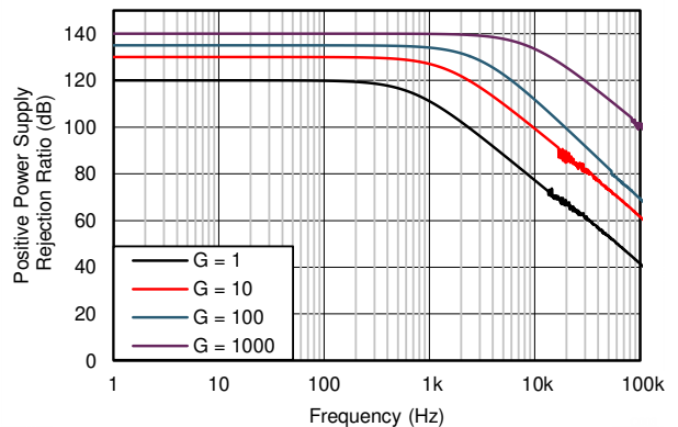
図 6-6. 正の電源除去比と周波数との関係
