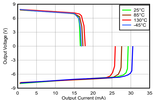
図 5-4. 出力電圧 対 負荷電流
