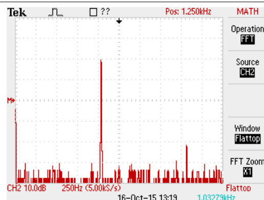
図 7-7. INA126 の出力の FFT は、60Hz 同相信号が除去されていることを示しています
