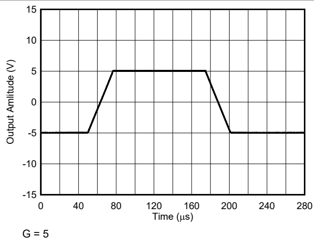
図 5-20. 大信号応答
