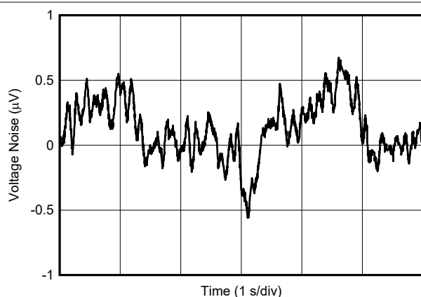
図 5-21. 0.1Hz~10Hz の電圧ノイズ
