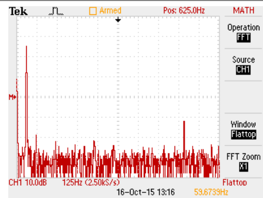
図 7-5. 前の図の信号の FFT は、60Hz の同相モードと 5kHz の差動信号の両方を示しています
