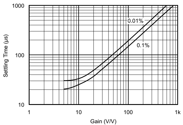
図 5-10. セトリングタイムとゲインとの関係
