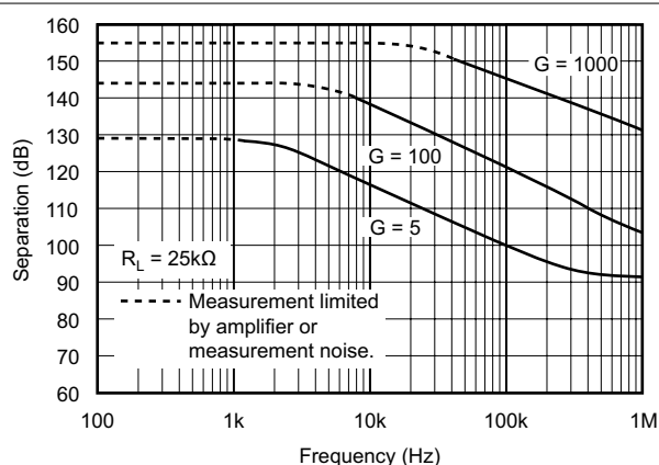
図 5-22. チャンネル セパレーションと周波数との関係、RTI (デュアルバージョンの場合)
