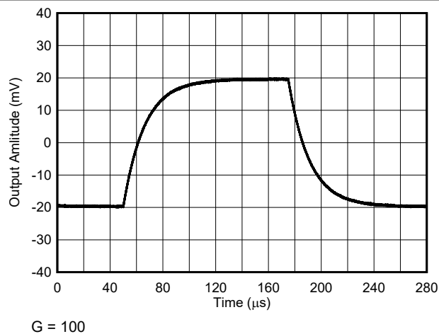
図 5-19. 小信号応答
