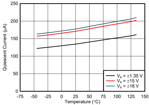
図 5-13. 静止電流と温度との関係
