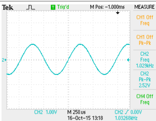
図 7-6. ゲイン 250 での INA126 の出力における復元差動信号
