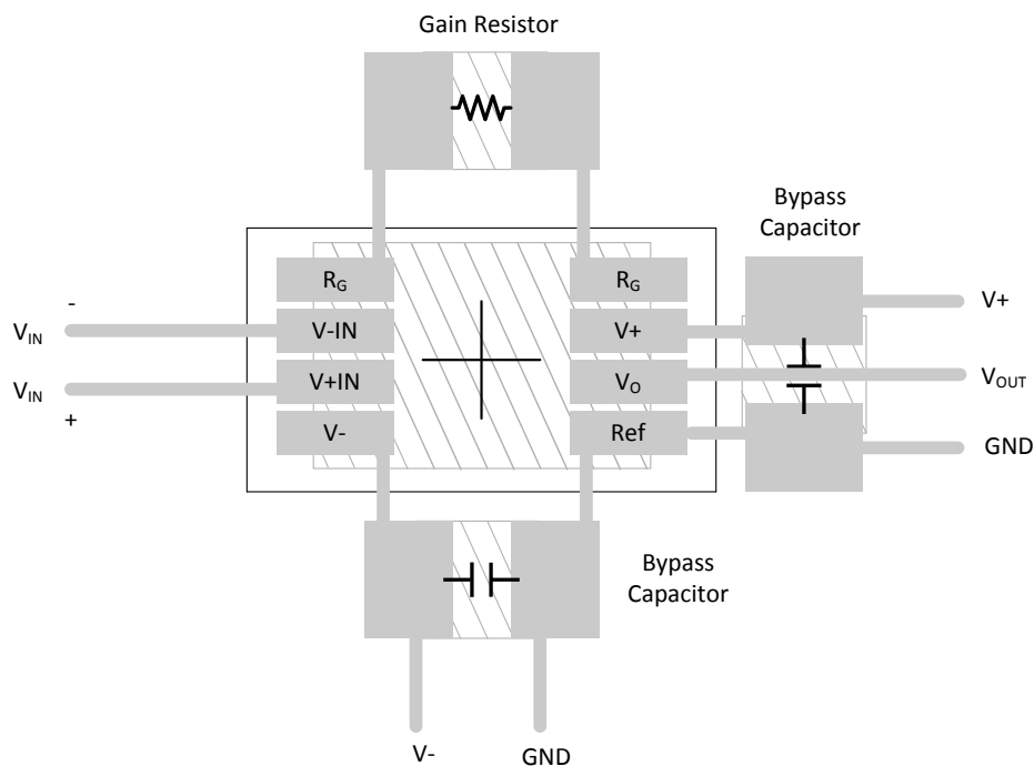
図 7-9. INA126 のレイアウト例
