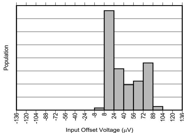
図 6-3. INA241A3-Q1 および INA241A4-Q1 の入力オフセットの製品分布
