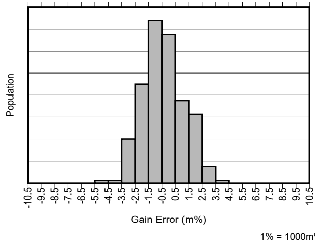
図 6-11. INA241A4-Q1 および INA241A5-Q1 のゲイン誤差の製品分布
