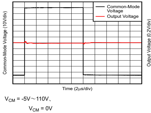
図 6-33. 同相電圧の高速過渡パルス
