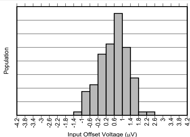
図 6-4. INA241A5-Q1 の入力オフセットの製品分布
