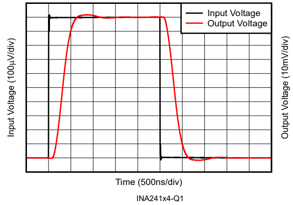
図 6-34. 小ステップ応答
