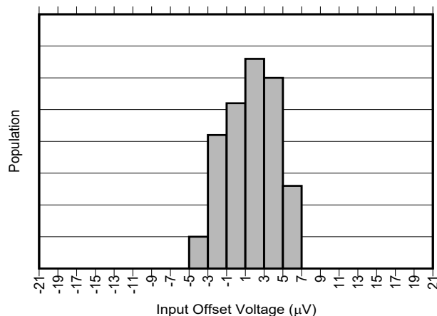
図 6-1. INA241A1-Q1 の入力オフセットの製品分布
