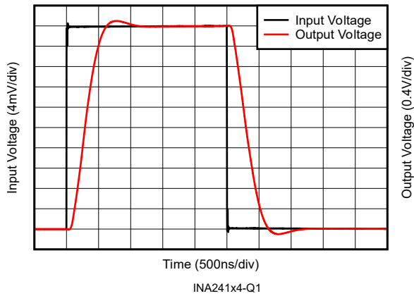
図 6-35. 大ステップ応答
