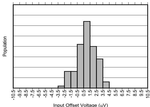
図 6-2. INA241A2-Q1 の入力オフセットの製品分布
