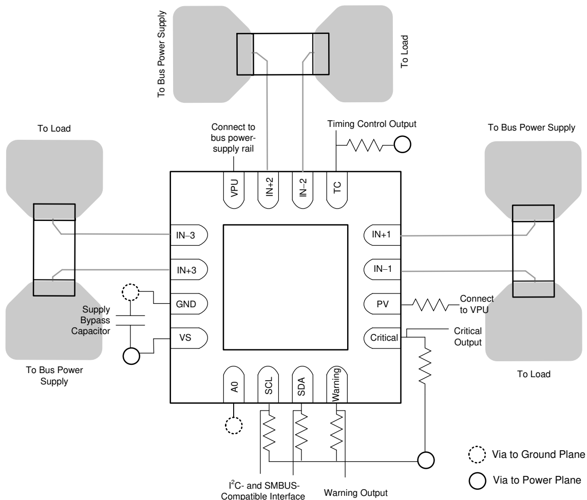
図 9-4. レイアウト例
