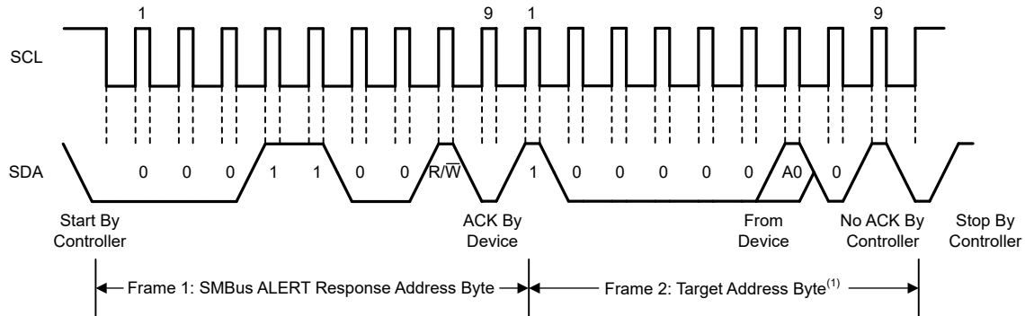
図 7-12. SMBus アラートのタイミング図
