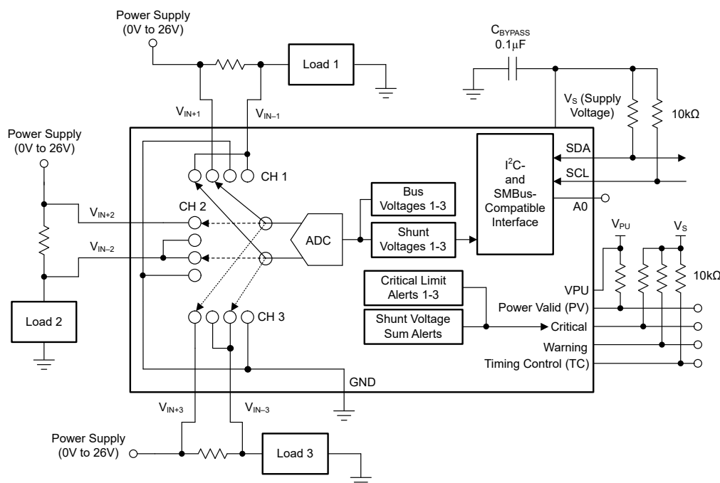
代表的なアプリケーション
