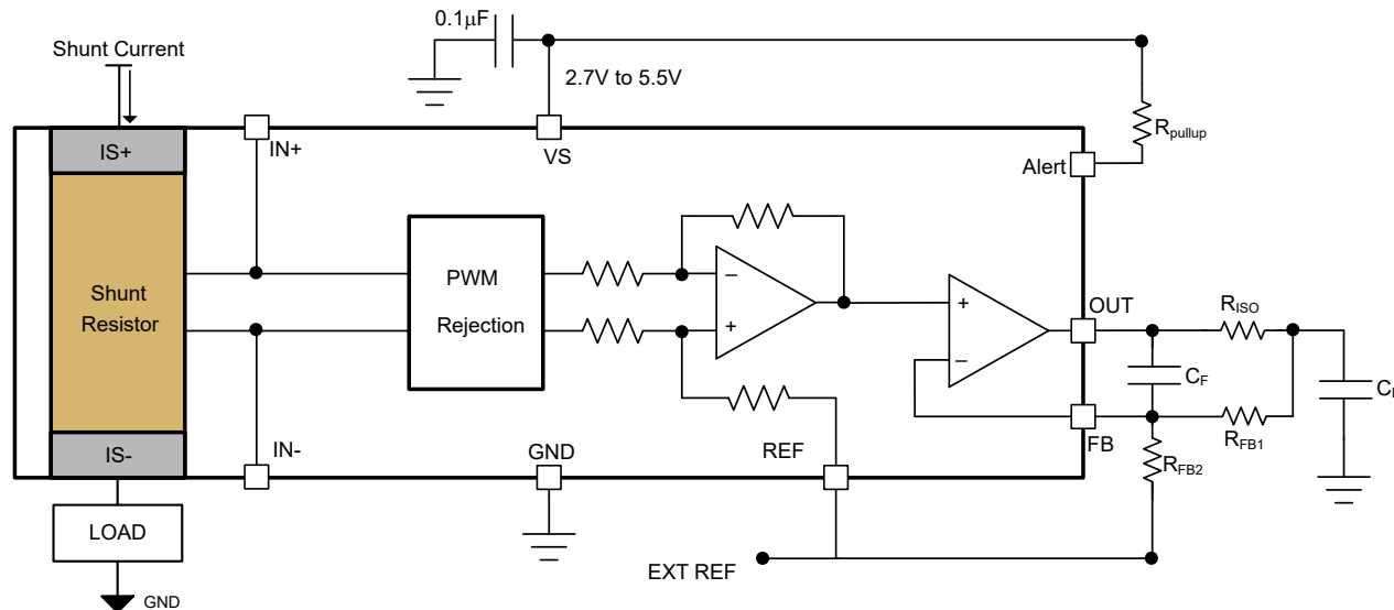
図 7-5. INA750x-Q1、RISO - デュアル フィードバック
