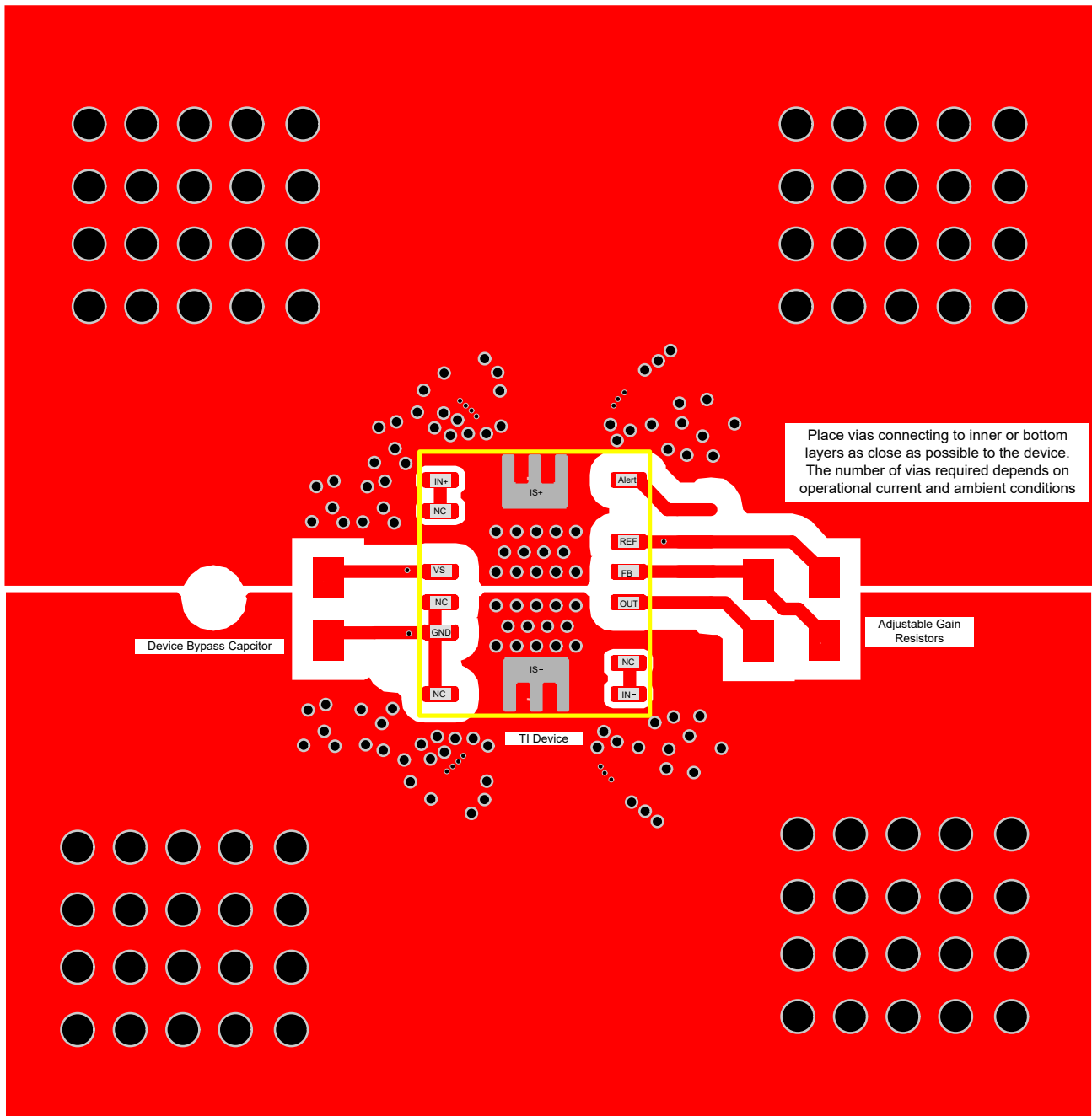
図 7-12. INA750x-Q1 レイアウト例
