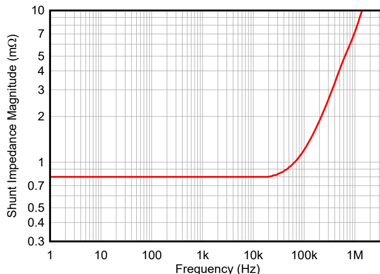
図 7-3. シャントインピーダンスと周波数との関係
