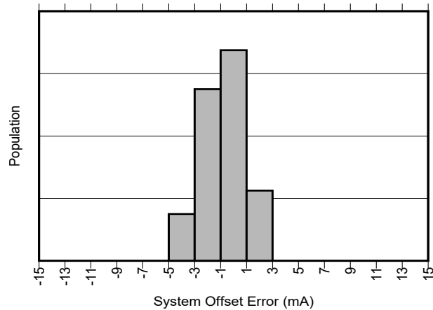
図 5-1. INA750A-Q1 入力オフセット電流の製品分布
