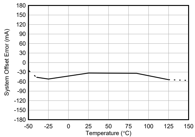
図 5-4. INA750B-Q1 の入力オフセット電流と温度との関係
