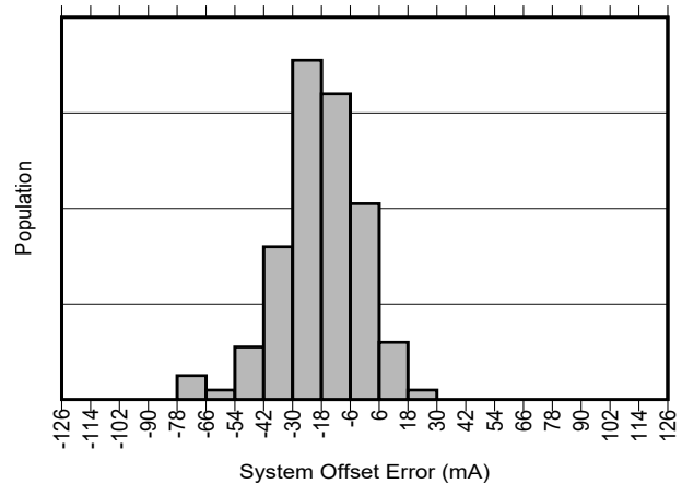
図 5-2. INA750B-Q1 入力オフセット電流の製品分布
