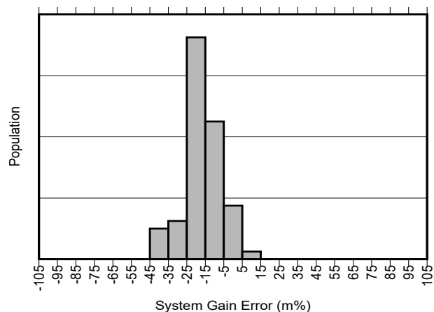
図 5-11. INA750A-Q1 ゲイン誤差の製品分布
