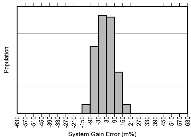
図 5-12. INA750B-Q1 ゲイン誤差の製品分布
