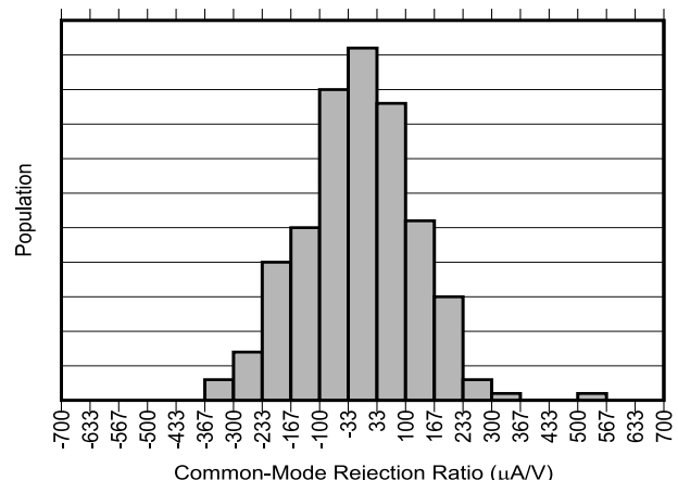
図 5-6. INA750B-Q1 同相除去比の製品分布
