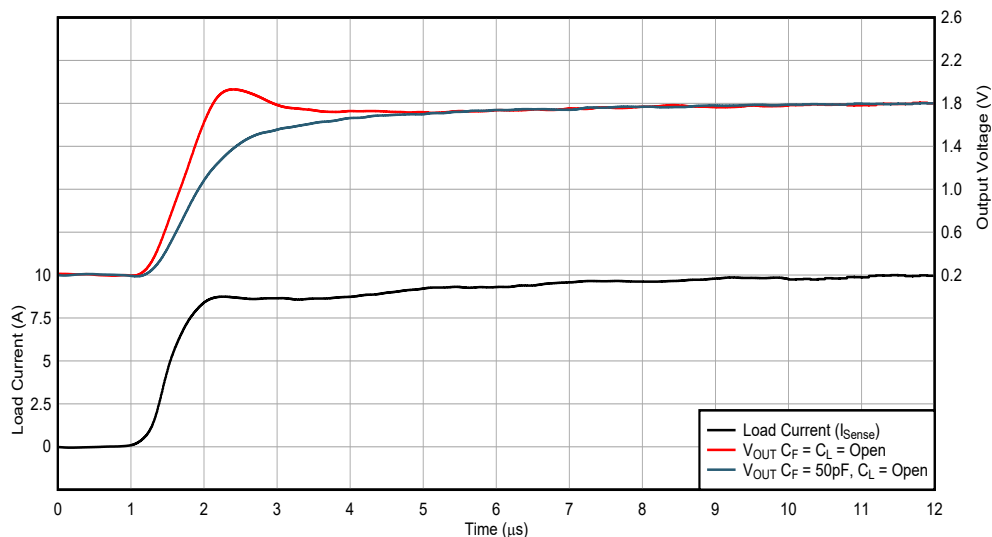
図 7-6. INA750x-Q1 RISO デュアル フィードバックの前後での負荷ステップ応答により、可変ゲイン 1 を実現
