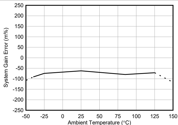
図 5-13. INA750A-Q1 ゲイン誤差と温度との関係
