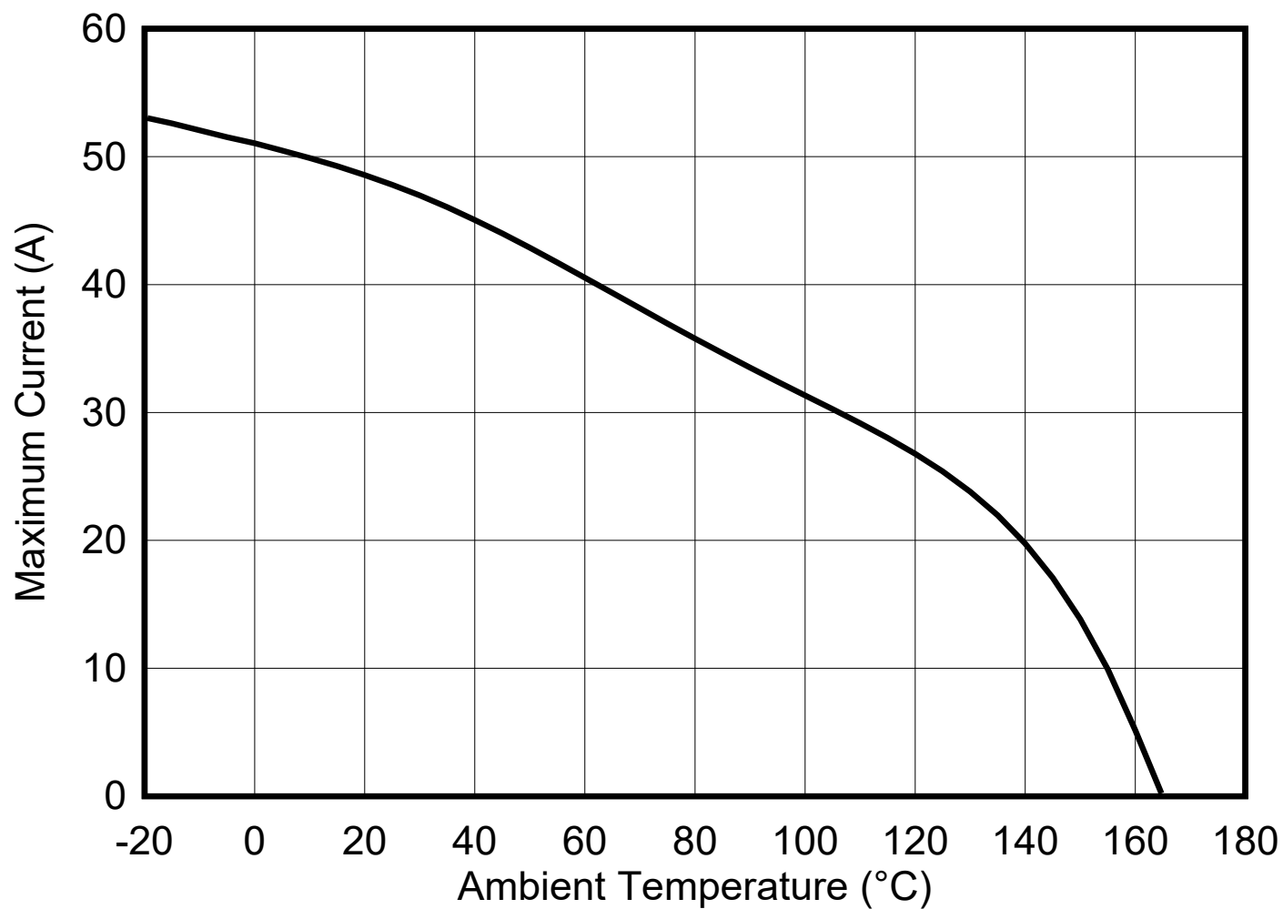
最大連続電流と周囲温度との関係
