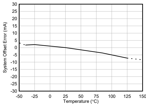
図 5-3. INA750A-Q1 の入力オフセット電流と温度との関係
