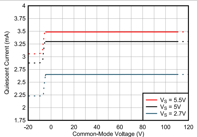
図 5-24. 静止電流と同相電圧との関係
