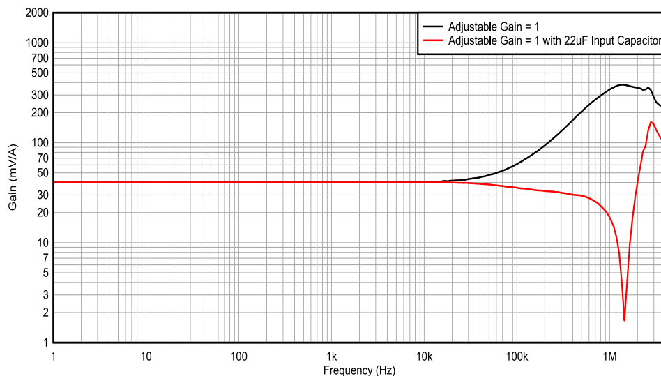
図 7-4. INA750x-Q1 のゲインと、22 \mu F 入力コンデンサの追加前後の周波数との関係
