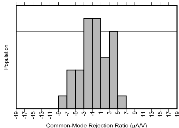
図 5-5. INA750A-Q1 同相除去比の製品分布
