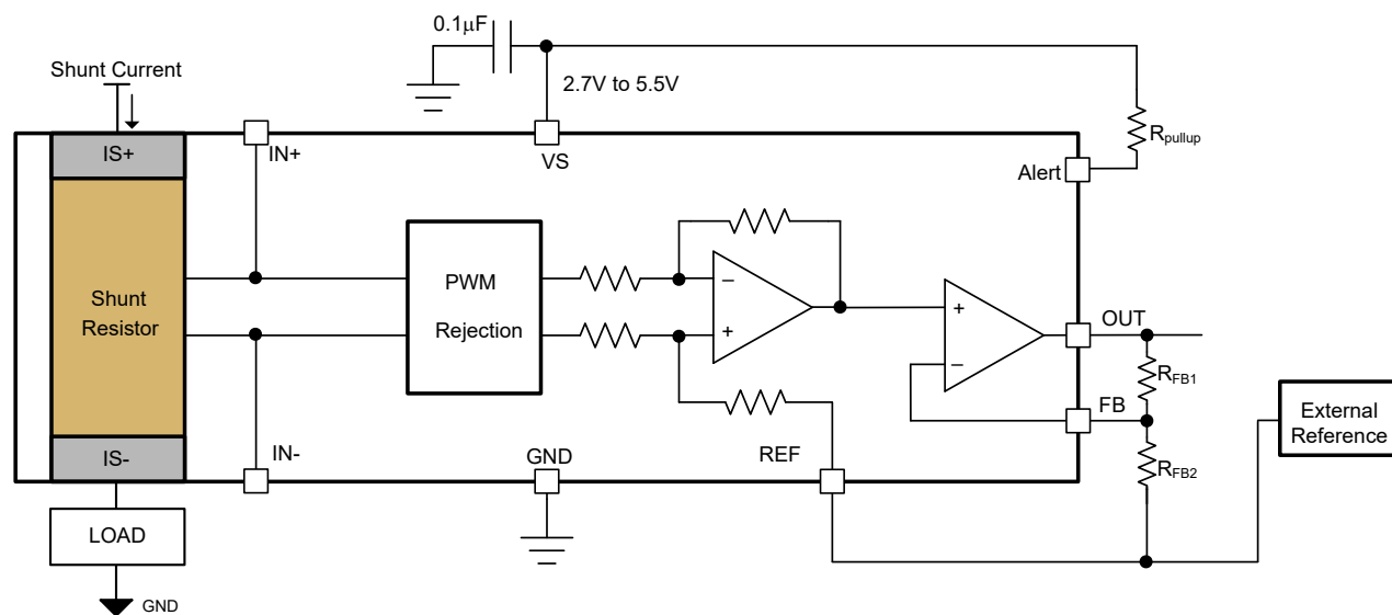
図 6-10. 熱アラート機能
