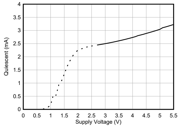
図 5-22. 静止電流と電源電圧との関係
