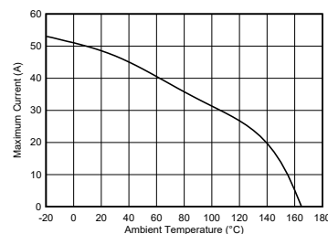
最大連続電流と周囲温度との関係
