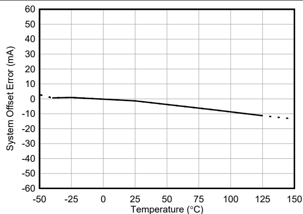
図 5-3. INA791A-Q1 の入力オフセット電流と温度との関係
