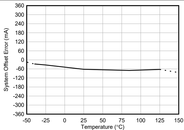
図 5-4. INA791B-Q1 の入力オフセット電流と温度との関係
