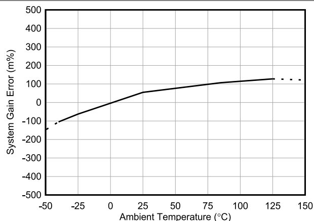
図 5-14. INA791B-Q1 ゲイン誤差と温度との関係
