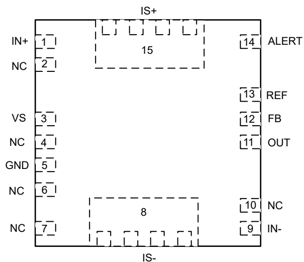
図 4-1. INA791x-Q1 ウェットブル DEK パッケージ 15 ピン VQFN 上面図
