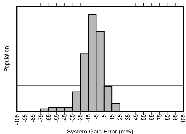
図 5-11. INA791A-Q1 ゲイン誤差の製品分布
