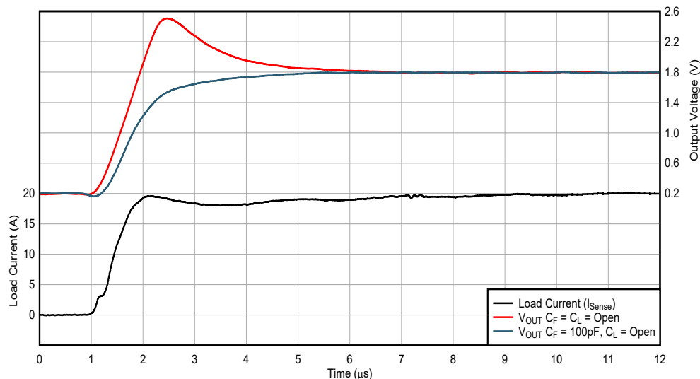
図 7-6. INA791x-Q1 RISO デュアル フィードバックの前後での負荷ステップ応答により、可変ゲイン 1 を実現
