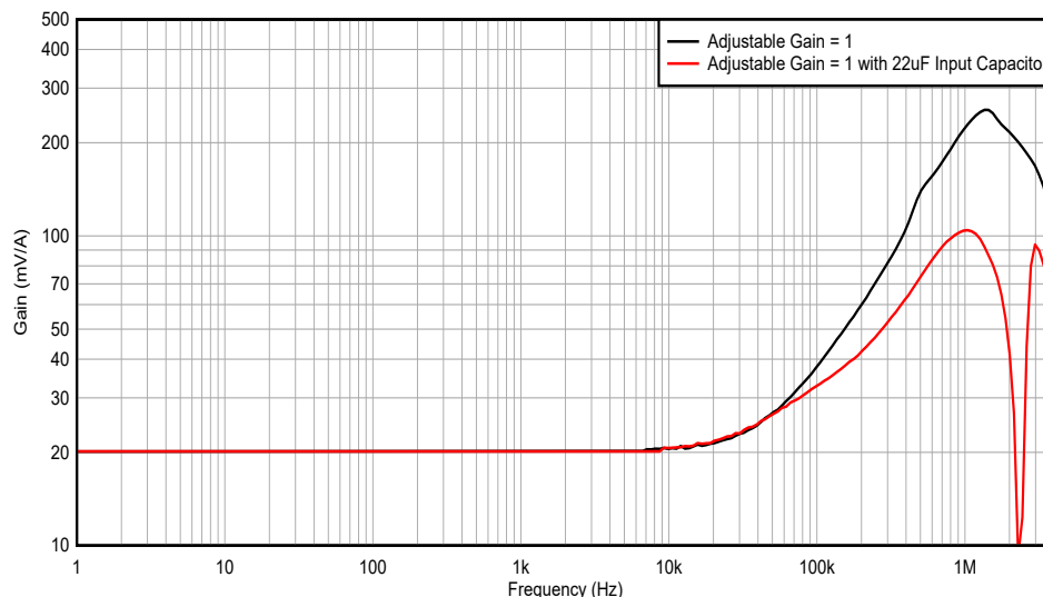
図 7-4. INA791x-Q1 のゲインと、22 \mu F 入力コンデンサの追加前後の周波数との関係
