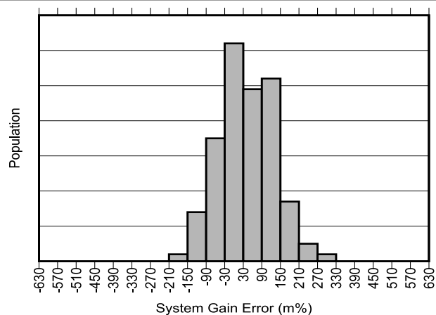
図 5-12. INA791B-Q1 ゲイン誤差の製品分布
