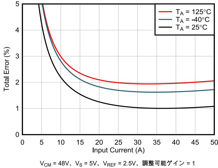
図 7-2. INA791B-Q1 総誤差と入力電流
