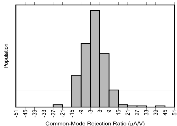
図 5-5. INA791A-Q1 同相除去比の製品分布
