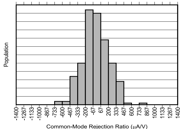
図 5-6. INA791B-Q1 同相除去比の製品分布
