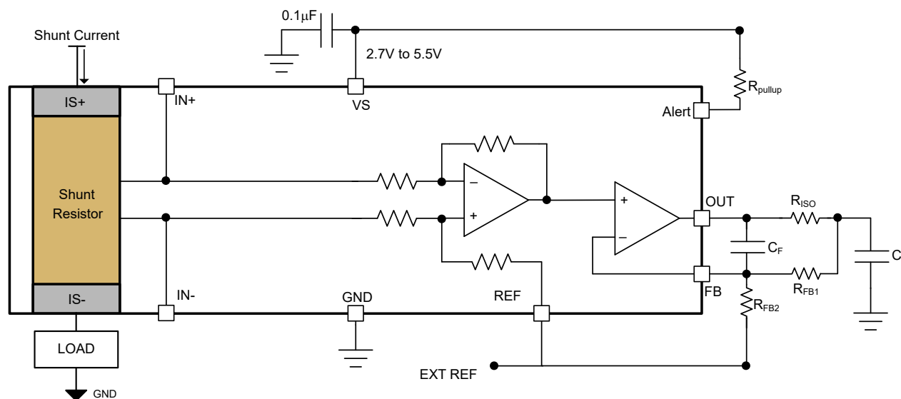
図 7-5. INA791x-Q1、RISO - デュアル フィードバック
