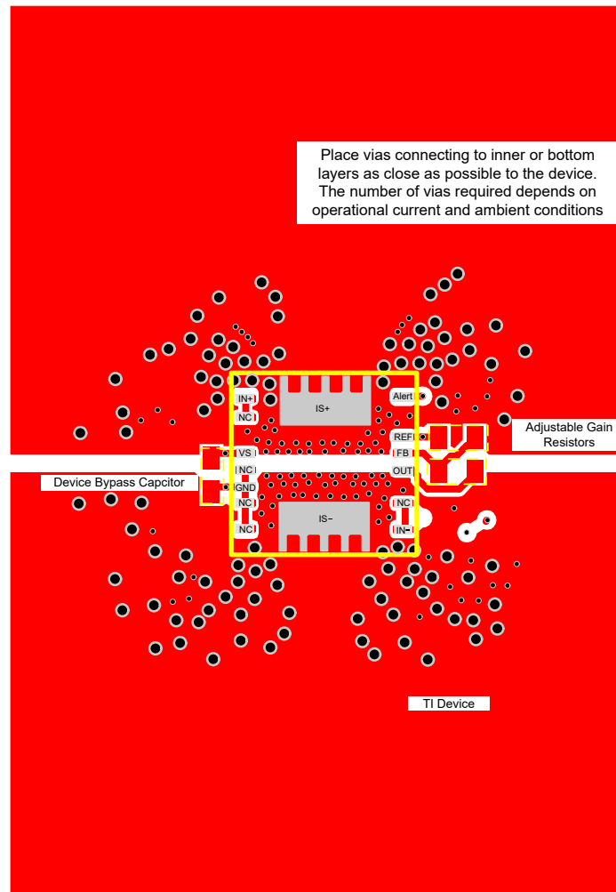
図 7-10. INA791x-Q1 レイアウト例
