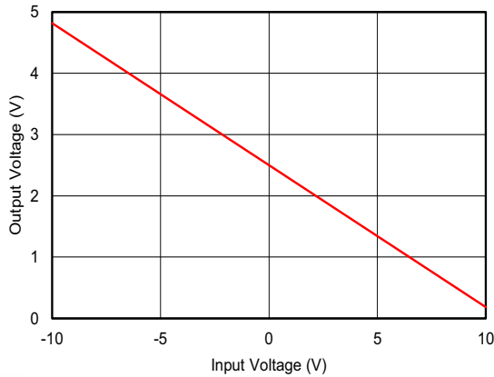
図 9-4. PLC の出力電圧と入力電圧との関係
