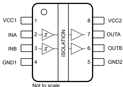
図 5-1. ISO6020H および ISO6020L の上面図
