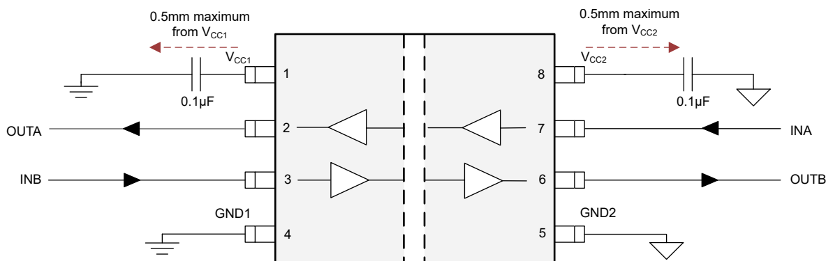
図 9-2. ISO602x の一般的な回路例
