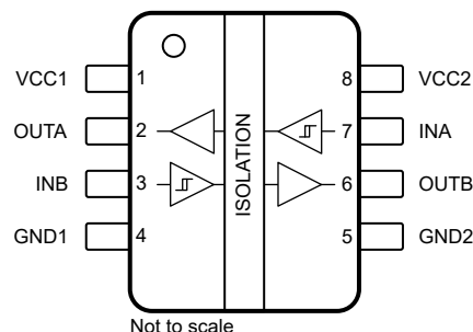
図 5-2. ISO6021H および ISO6021L の上面図
