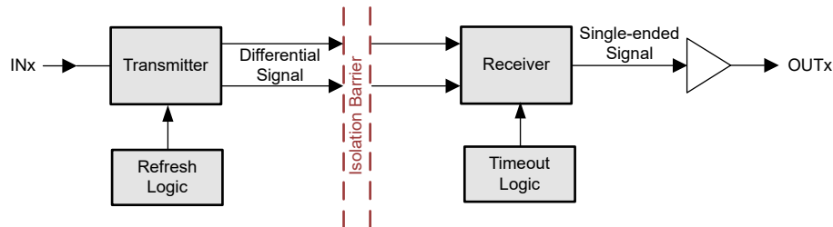
図 8-1. エッジベースのデジタルアイソレータの概念ブロック図
