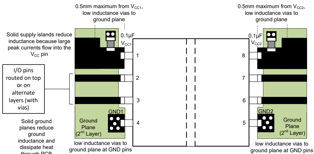
図 9-3. レイアウト例
