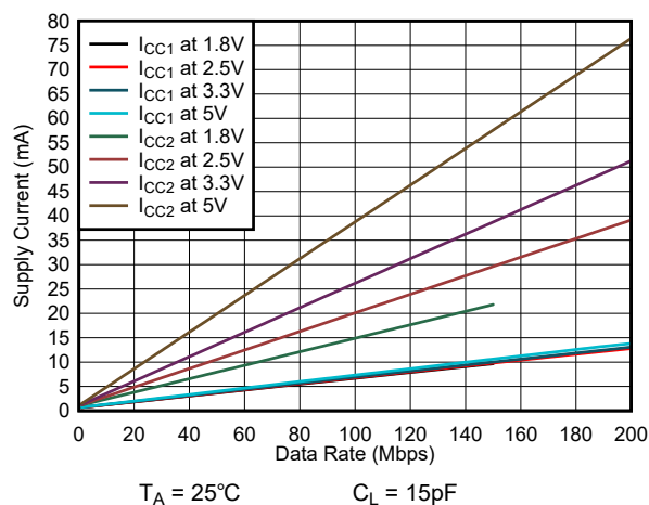
図 6-7. ISO6040H または ISO6040L の消費電流とデータレートとの関係 (15pF 負荷時)
