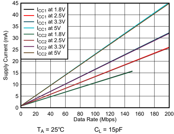
図 6-11. ISO6042H または ISO6042L の消費電流とデータレートとの関係 (15pF 負荷時)
