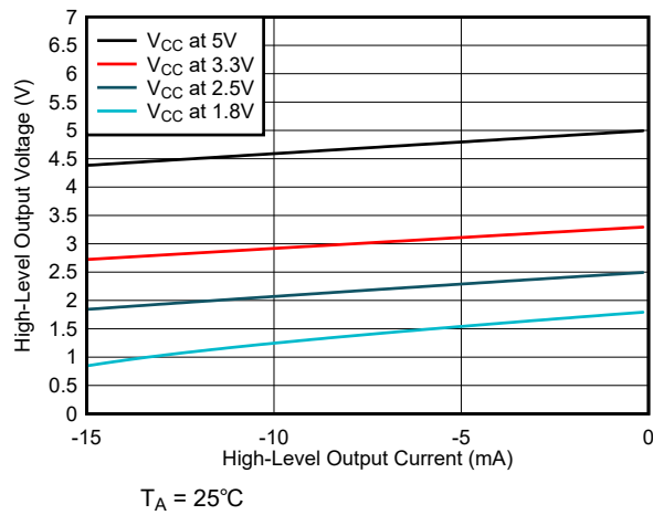
図 6-13. High レベル出力電圧と High レベル出力電流との関係
