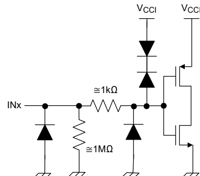
図 8-3. 入力 (INx) デフォルト High (接尾辞 L が付いたデバイス) 回路図
