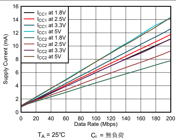
図 6-10. ISO6041H または ISO6041L の消費電流とデータレートとの関係 (無負荷時)
