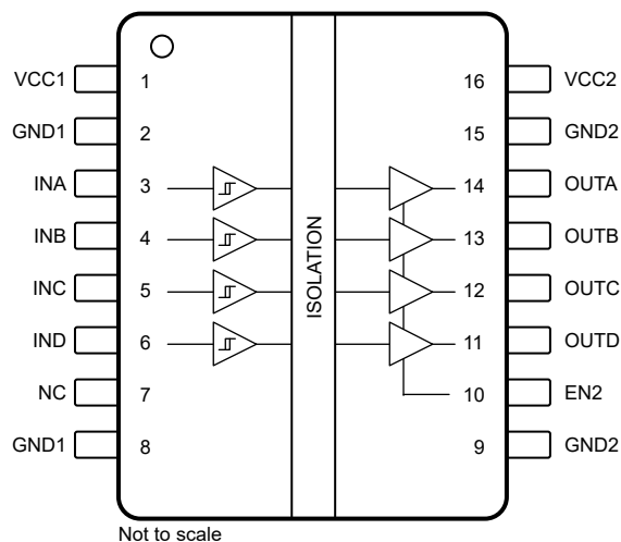
図 5-1. ISO6040H および ISO6040L の上面図
