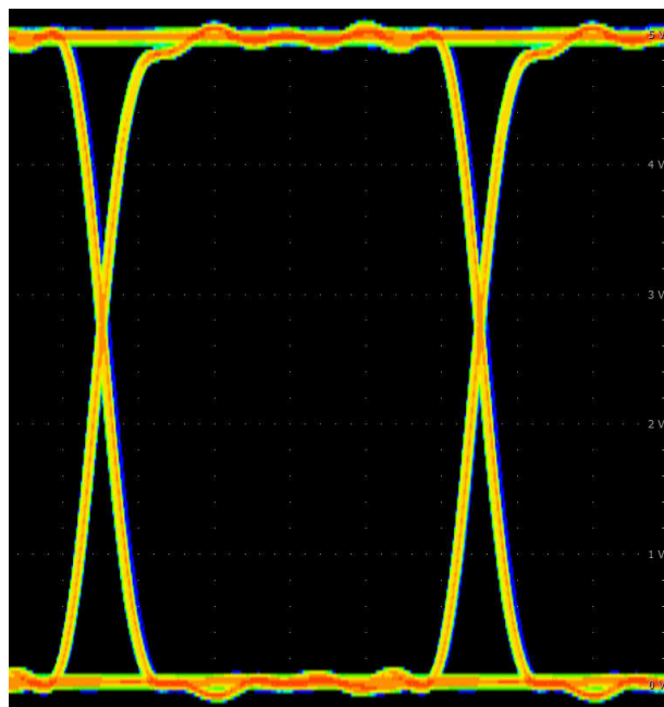
図 9-4. ISO604x アイダイアグラム (200Mbps PRBS 2^{16} - 1 , 5V, 25°C)
