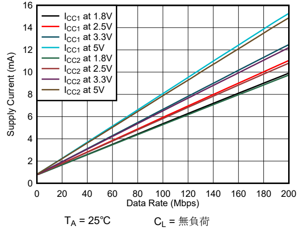
図 6-12. ISO6042H または ISO6042L の消費電流とデータレートとの関係 (無負荷時)
