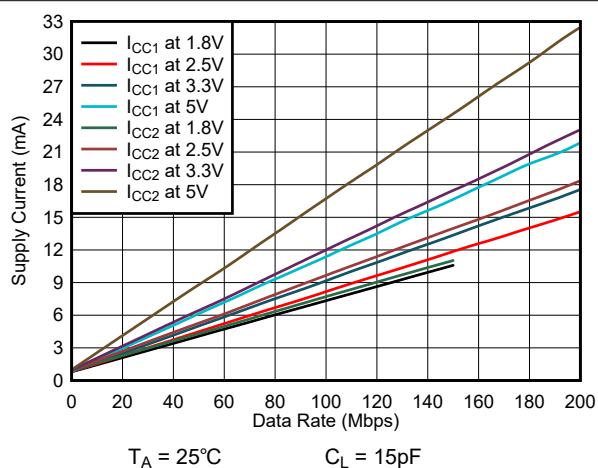
図 6-9. ISO6041H または ISO6041L の消費電流とデータレートとの関係 (15pF 負荷時)
