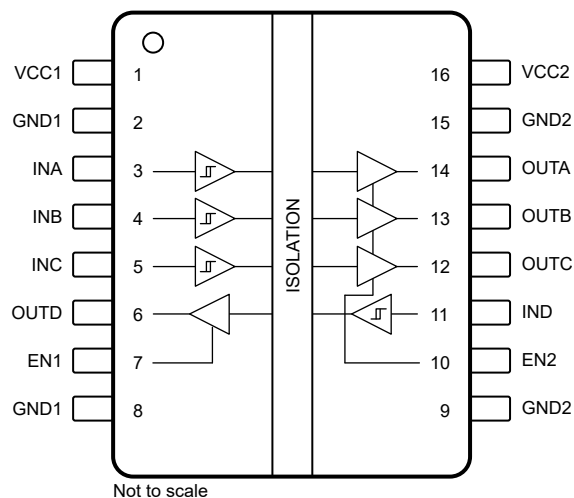
図 5-2. ISO6041H および ISO6041L の上面図
