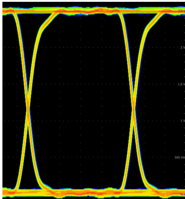
図 9-6. ISO604x アイダイアグラム (200Mbps PRBS 2^{16} - 1 、2.5V、25°C)
