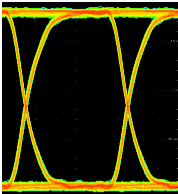
図 9-7. ISO604x アイダイアグラム (200Mbps PRBS 2^{16} - 1 、1.8V、25°C)
