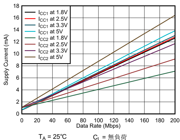
図 6-8. ISO6040H または ISO6040L の消費電流とデータレートとの関係 (無負荷時)
