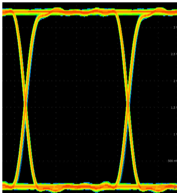
図 9-5. ISO604x アイダイアグラム (200Mbps PRBS 2^{16} - 1 , 3.3V, 25°C)
