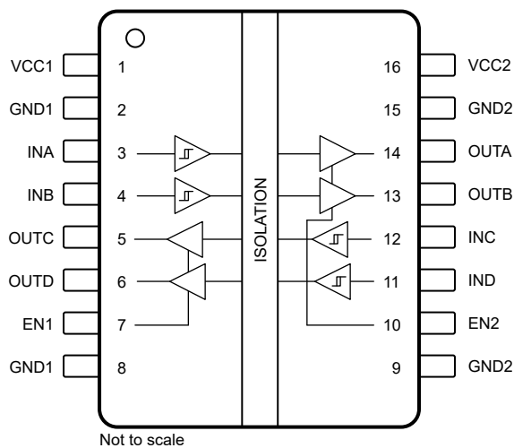
図 5-3. ISO6042H および ISO6042L の上面図
