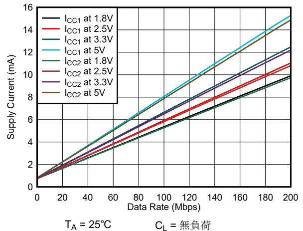
図 6-12. ISO6042H または ISO6042L の消費電流とデータレートとの関係 (無負荷時)
