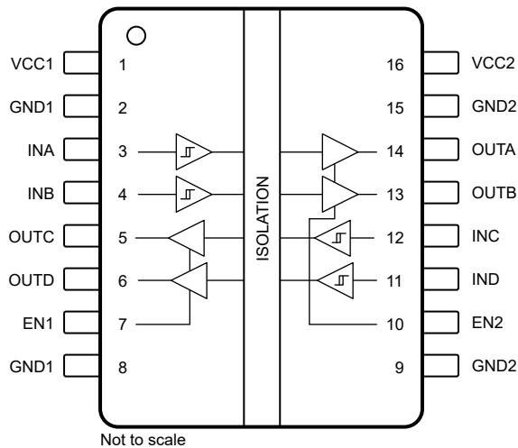
図 5-3. ISO6042H および ISO6042L の上面図
