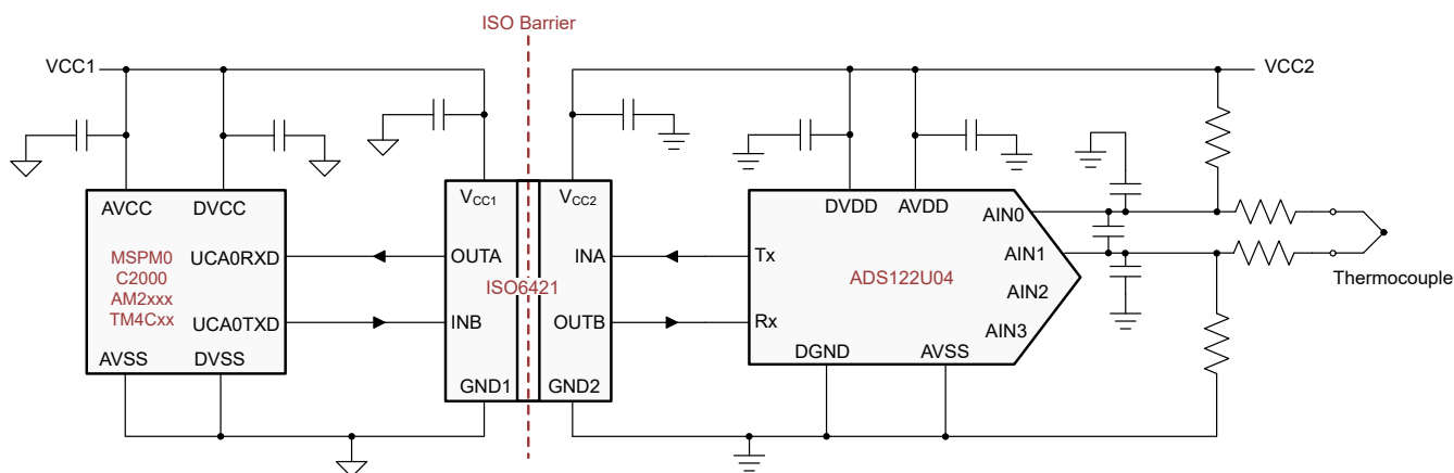
図 9-1. 2 チャネルの代表的なアプリケーション
