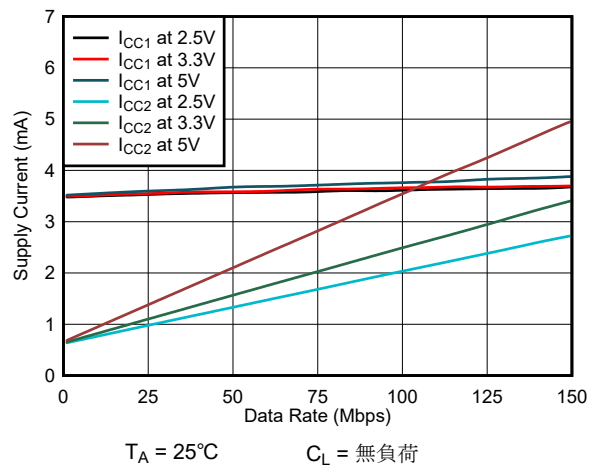
図 6-6. ISO6420-Q1 または ISO6420F-Q1 の消費電流とデータレートとの関係 (無負荷時)
