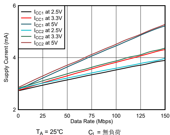
図 6-8. ISO6421-Q1 または ISO6421F-Q1 の消費電流とデータレートとの関係 (無負荷時)
