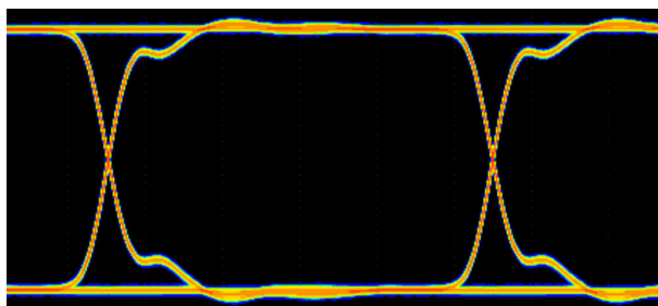
図 9-4. ISO642x-Q1 アイダイアグラム (100Mbps PRBS 2^{16} - 1 , 3.3V, 25°C)
