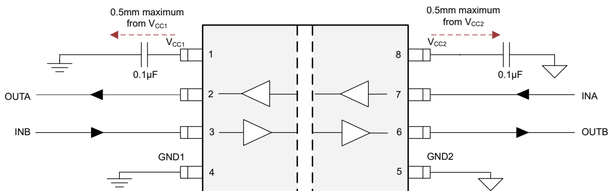
図 9-2. ISO642x-Q1 の一般的な回路例
