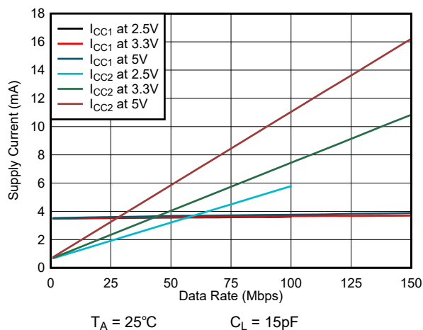
図 6-5. ISO6420-Q1 または ISO6420F-Q1 の消費電流とデータレートとの関係 (15pF 負荷時)
