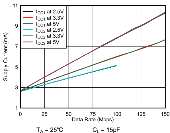
図 6-7. ISO6421-Q1 または ISO6421F-Q1 の消費電流とデータレートとの関係 (15pF 負荷時)
