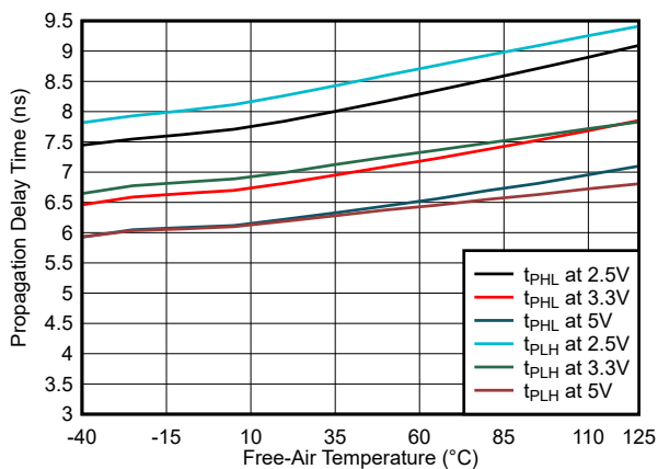
図 6-16. 伝搬遅延時間と周囲温度との関係
