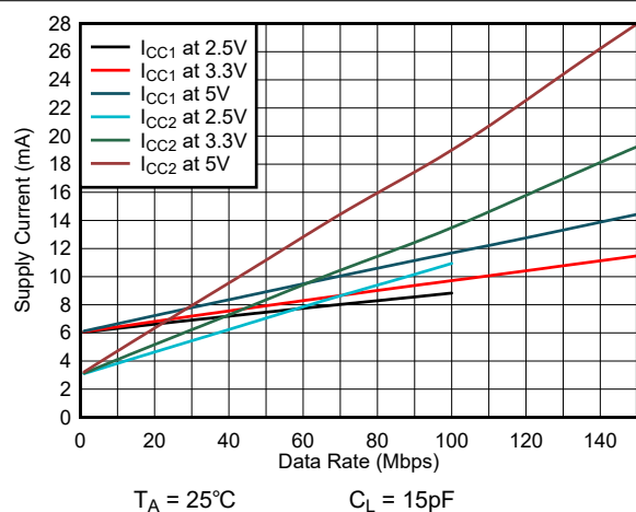
図 6-9. ISO6441-Q1 または ISO6441F-Q1 の消費電流とデータレートとの関係 (15pF 負荷時)
