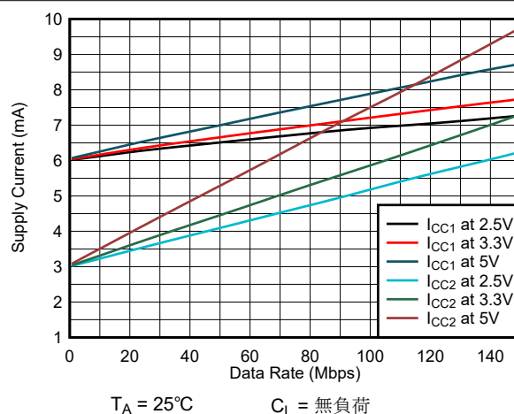
図 6-10. ISO6441-Q1 または ISO6441F-Q1 の消費電流とデータレートとの関係 (無負荷時)
