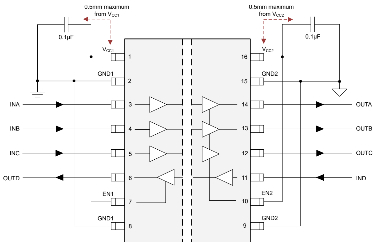
図 9-2. ISO644x-Q1 の一般的な回路例
