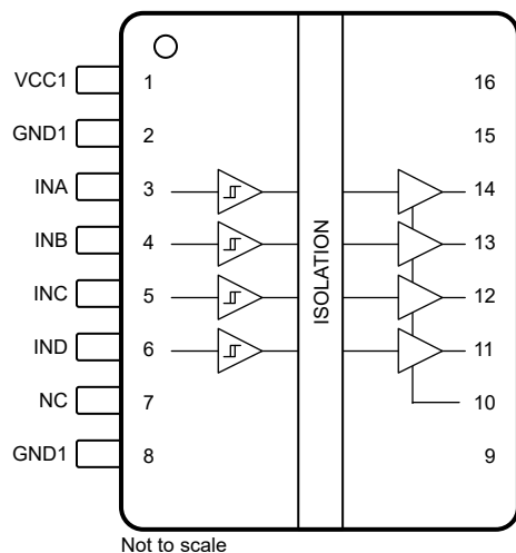
図 5-1. ISO6440-Q1 および ISO6440F-Q1 の上面図
