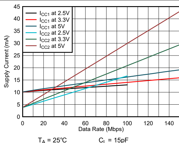
図 6-5. ISO6461 または ISO6461F の消費電流とデータレートとの関係 (15pF 負荷時)
