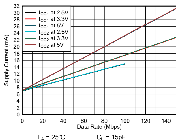
図 6-9. ISO6463 または ISO6463F の消費電流とデータレートとの関係 (15pF 負荷時)
