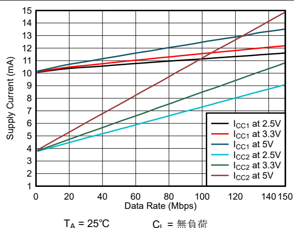
図 6-6. ISO6461 または ISO6461F の消費電流とデータレートとの関係 (無負荷時)
