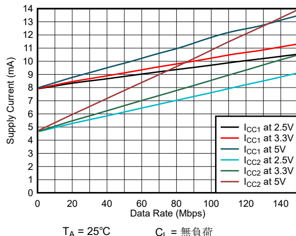
図 6-8. ISO6462 または ISO6462F の消費電流とデータレートとの関係 (無負荷時)
