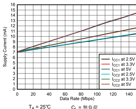
図 6-10. ISO6463 または ISO6463F の消費電流とデータレートとの関係 (無負荷時)
