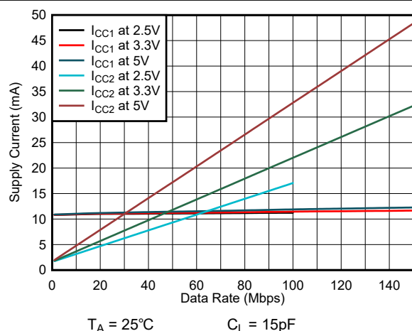
図 6-3. ISO6460 または ISO6460F の消費電流とデータレートとの関係 (15pF 負荷時)
