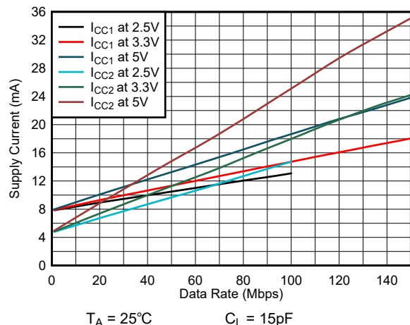
図 6-7. ISO6462 または ISO6462F の消費電流とデータレートとの関係 (15pF 負荷時)
