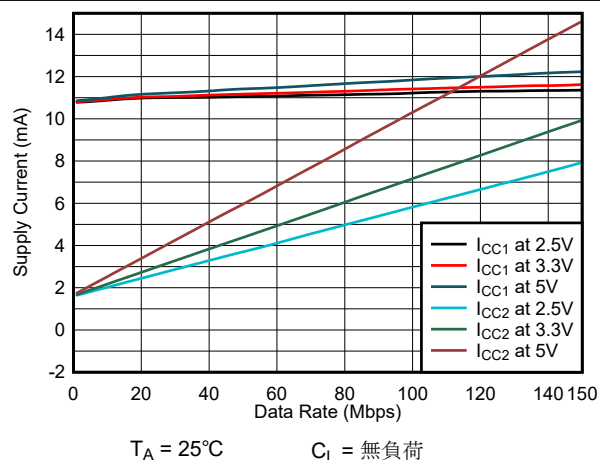
図 6-4. ISO6460 または ISO6460F の消費電流とデータレートとの関係 (無負荷時)
