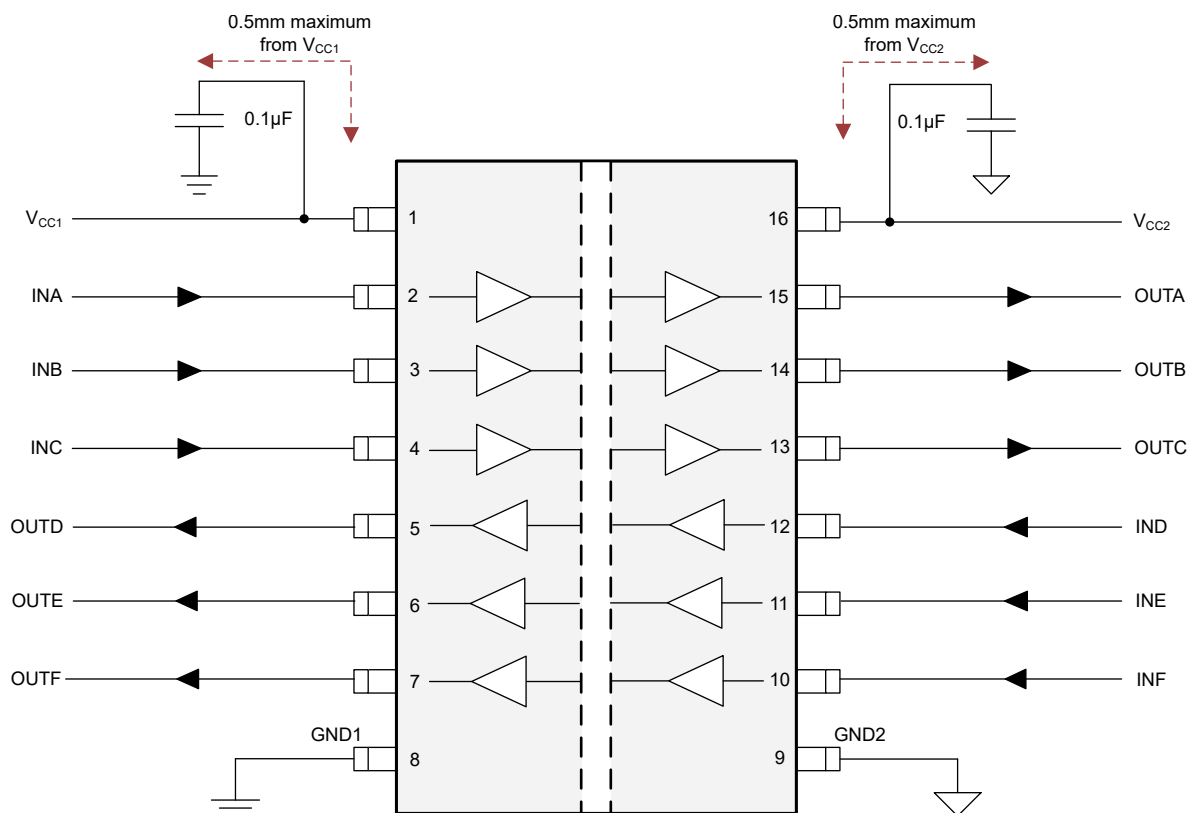
図 9-2. ISO646x の一般的な回路例
