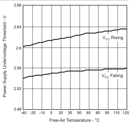
図 5-10. V CC 低電圧スレシヨルドと自由気流温度との関係
