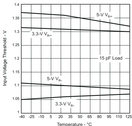
図 5-8. ISO722xA、ISO722xB、および ISO722xC の入力電圧 Low から High スwitchングスレシヨルドと自由気流温度との関係
