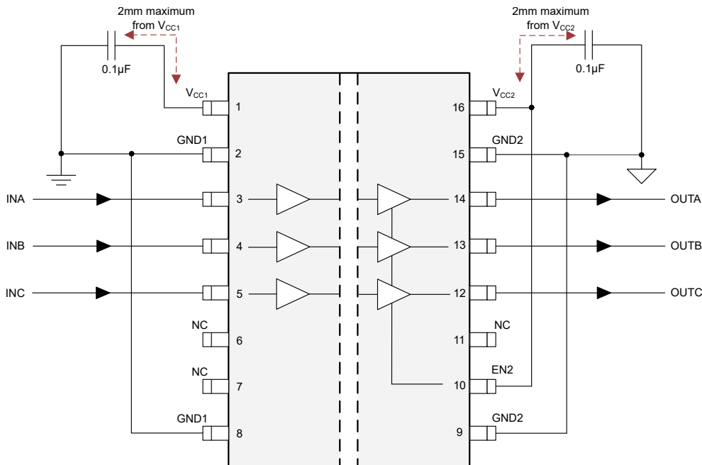
図 8-2. ISO7830 の標準の回路接続図
