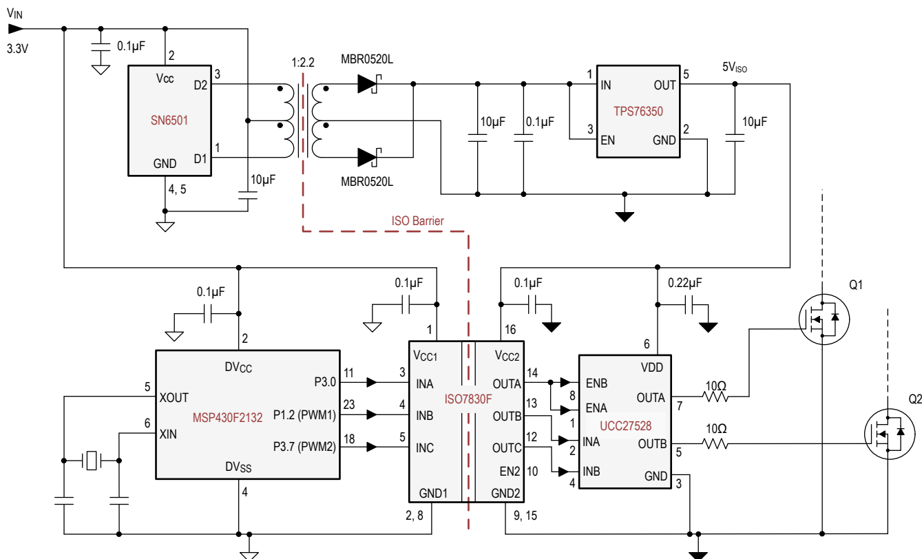
図 8-1. 絶縁型デュアル MOSFET/IGBT ゲート ドライブ回路
