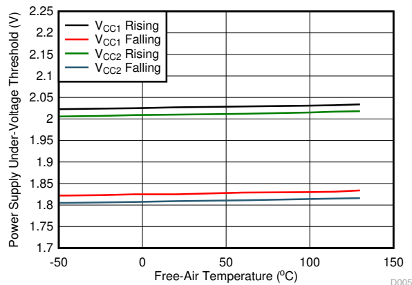
図 5-9. 電源低電圧スレッシュドと周囲温度との関係
