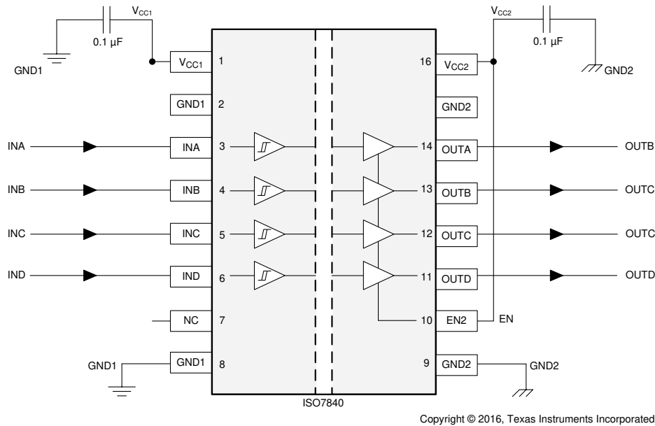
図 8-2. 標準的な ISO7840 回路フックアップ
