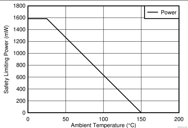
図 5-4. VDE に従う制限電力の熱特性低下曲線
