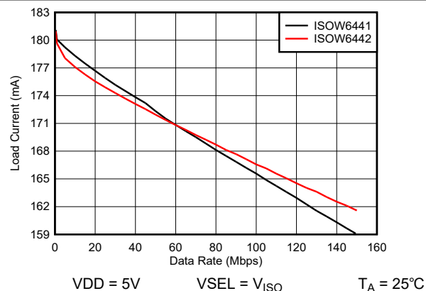
図 5-14. C_L = 15\text{pF} に負荷電流 ( I_{ISO} ) とデータ レートとの関係
