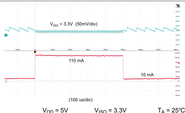
図 5-22. 10mA から 110mA への負荷過渡応答
