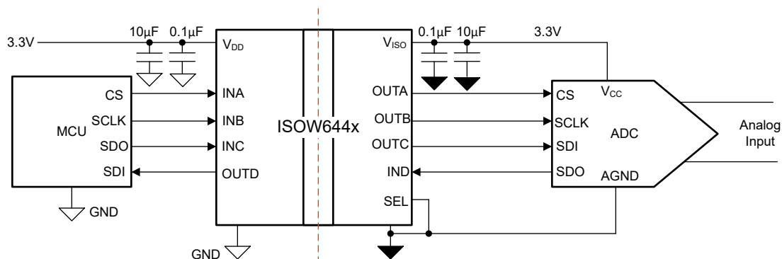
図 8-1. ISOW6441Q1 を使用する ADC センシング アプリケーション向けの絶縁電源および SPI
