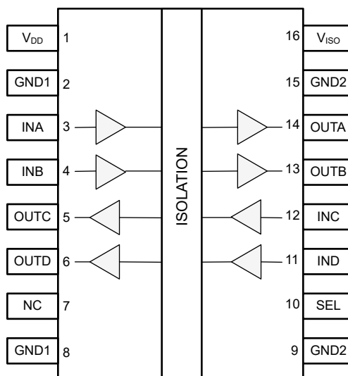
図 4-1. ISOW6442Q1 DWE パッケージ 16 ピン SOIC-WB 上面図
