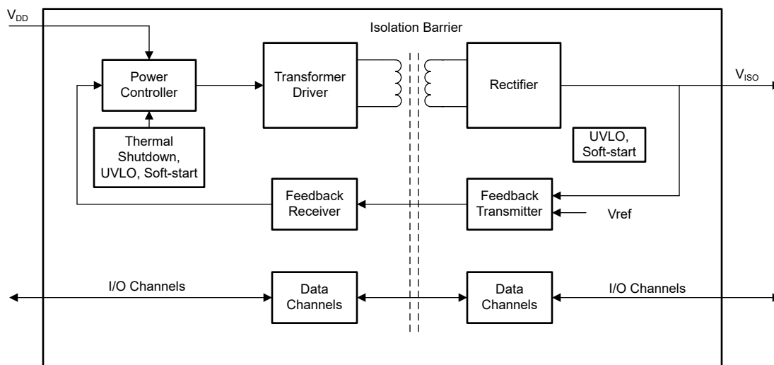
図 7-1. ISOW644x-Q1 のブロック図
