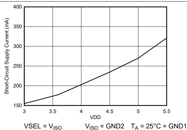
図 5-10. 短絡時電源電流 ( I_{DD} ) と電源電圧 (VDD) との関係
