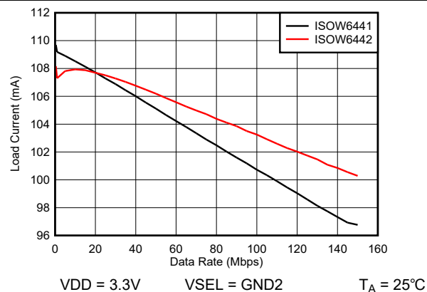
図 5-16. C_L = 15\text{pF} に負荷電流 ( I_{ISO} ) とデータ レートとの関係
