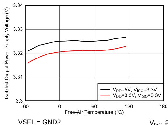
図 5-8. 3.3V 絶縁電源電圧 ( V_{ISO} ) と周囲温度との関係
