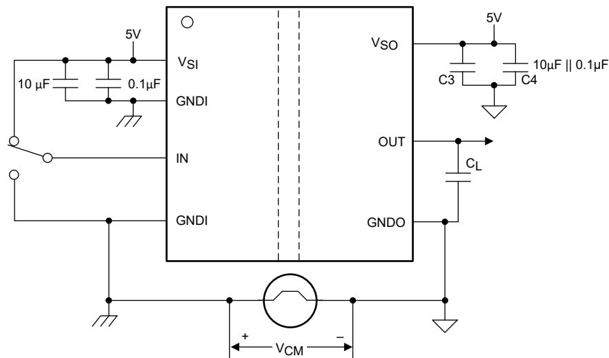
図 8-2. 標準的な ISOW6441Q1 回路のフックアップ
