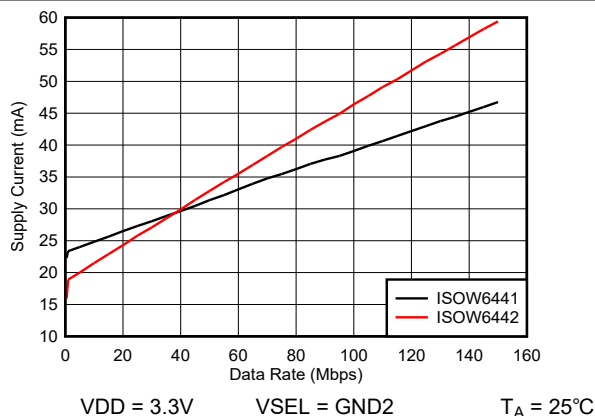
図 5-13. C_L = 15\text{pF} に電源電流 ( I_{DD} ) とデータ レートとの関係
