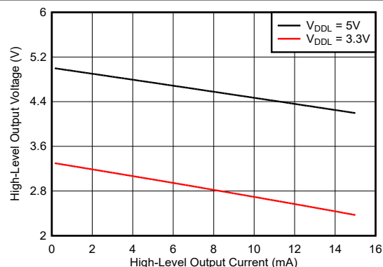
図 5-20. HIGH レベル出力電圧と HIGH レベル出力電流との関係
