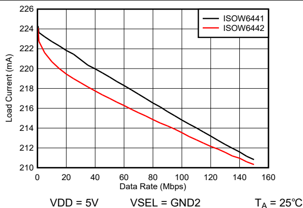
図 5-15. C_L = 15\text{pF} に負荷電流 ( I_{ISO} ) とデータ レートとの関係
