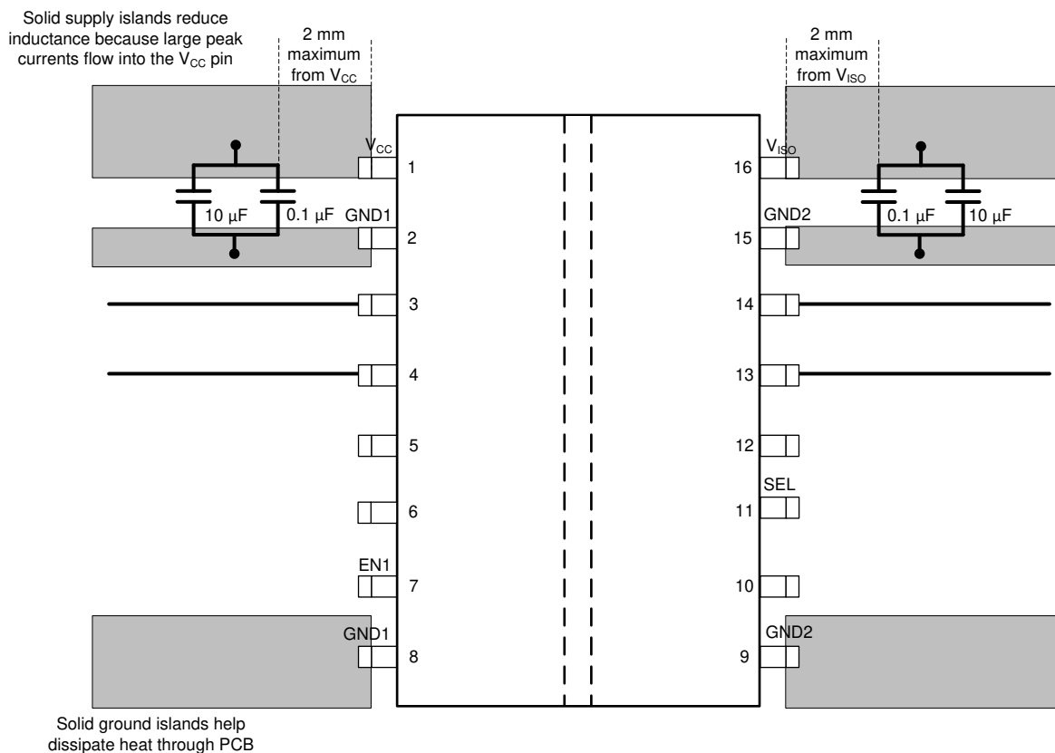
图 35. Layout Example
