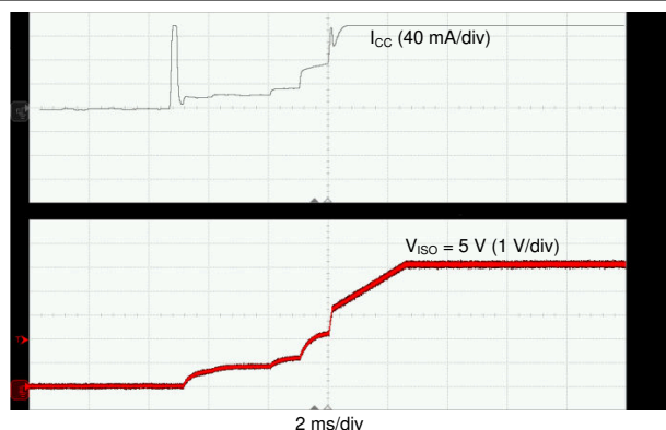
図 7-27. 120mA 負荷でのソフトスタート
