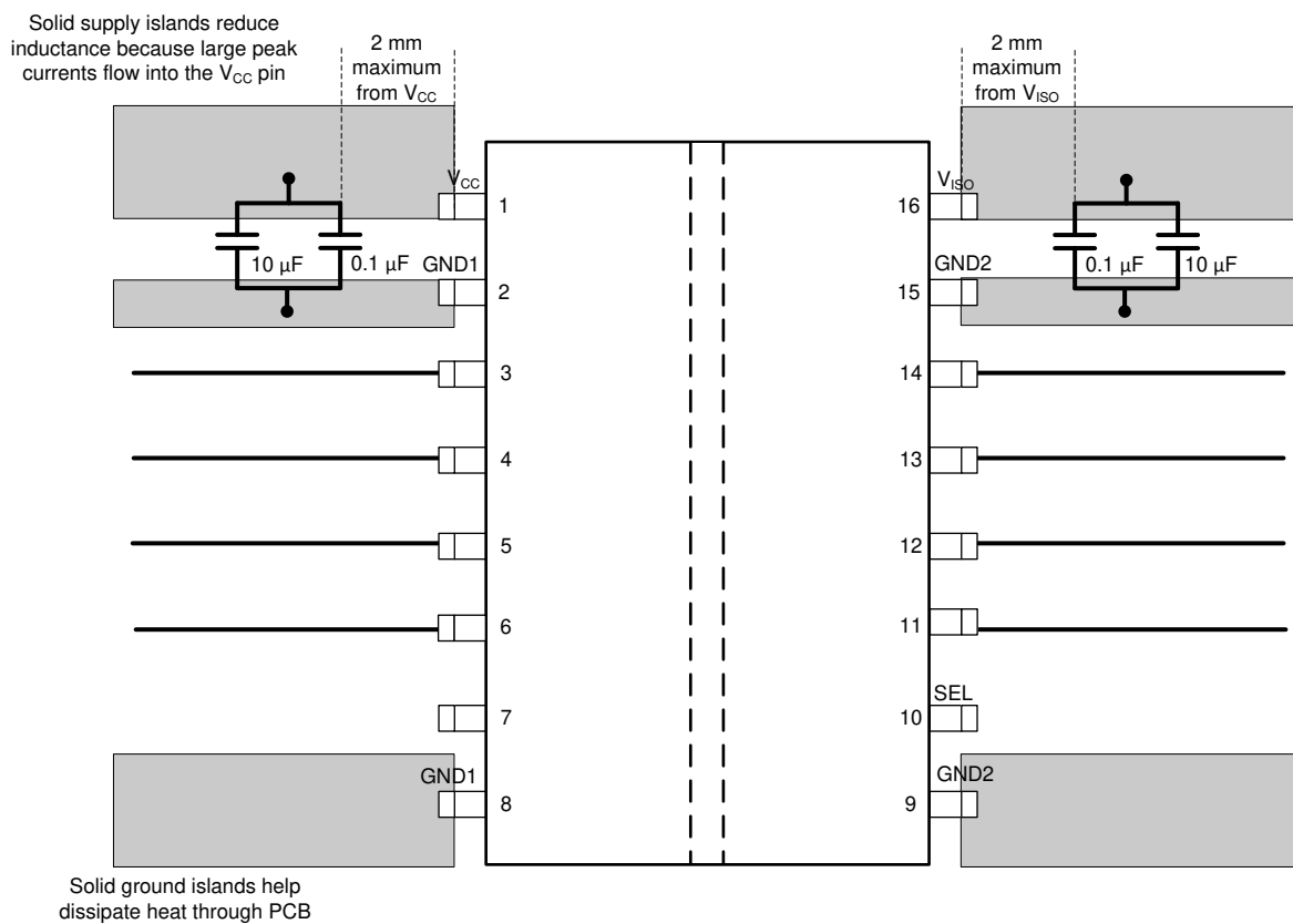
図 12-1. レイアウト例
