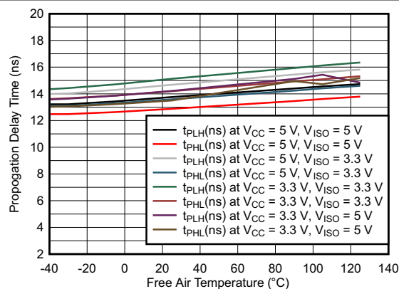
図 7-22. 伝播遅延時間と周囲温度との関係
