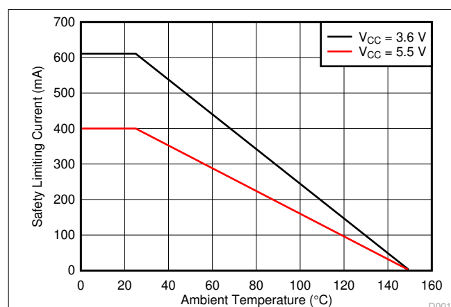
図 7-1. VDE による安全限界電流の熱特性低下曲線
