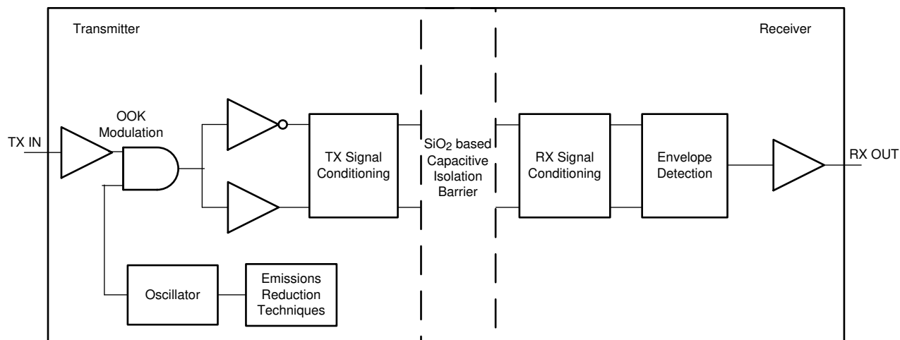
図 9-2. 容量性データチャネルの概念ブロック図
