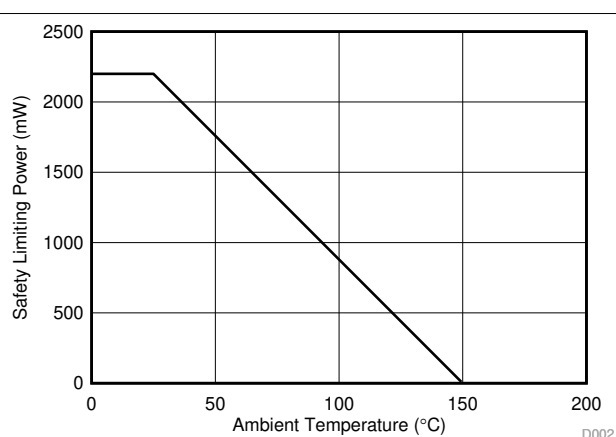
図 7-2. VDE による安全限界電力の熱特性低下曲線
