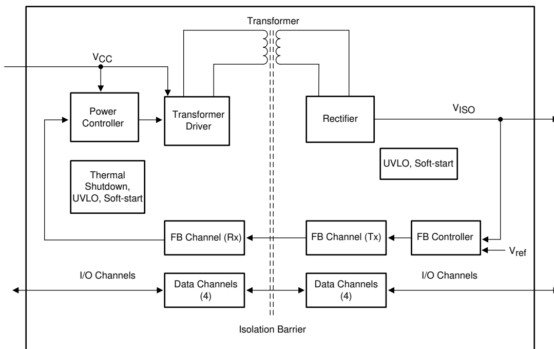
図 9-1. ブロック図
