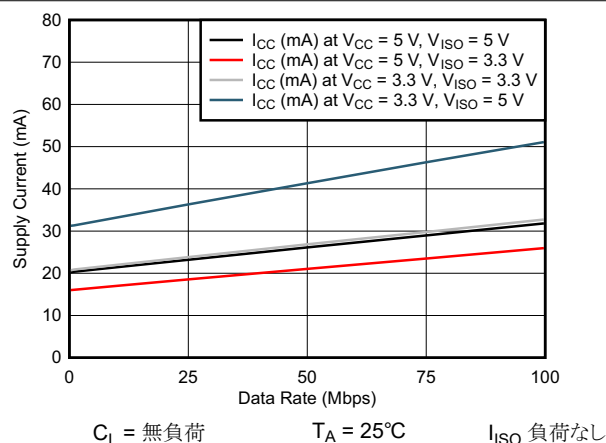
図 7-14. ISOW7841 電源電流とデータ・レートとの関係
