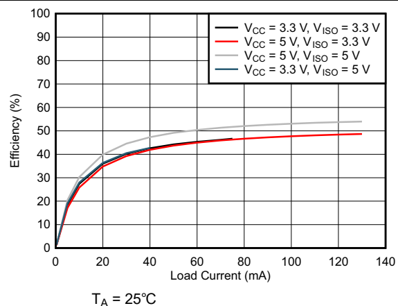
図 7-6. ISOW7841 効率と負荷電流 ( I_{ISO} ) との関係
