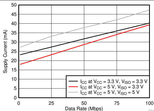
図 7-17. ISOW7843 消費電流とデータ・レートとの関係
