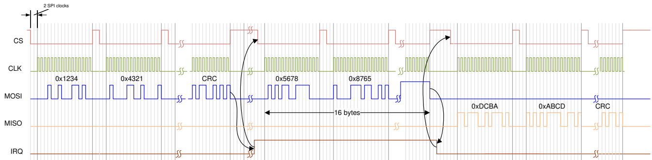
図 7-11. SPI 通信
