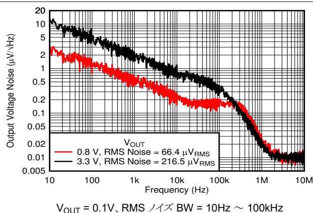
図 5-19. 出力ノイズ ( V_N ) と V_{OUT} との関係
