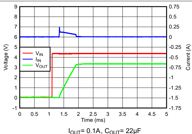
図 5-20. 22\mu\text{F} の C_{OUT} を使用した場合の突入電流
