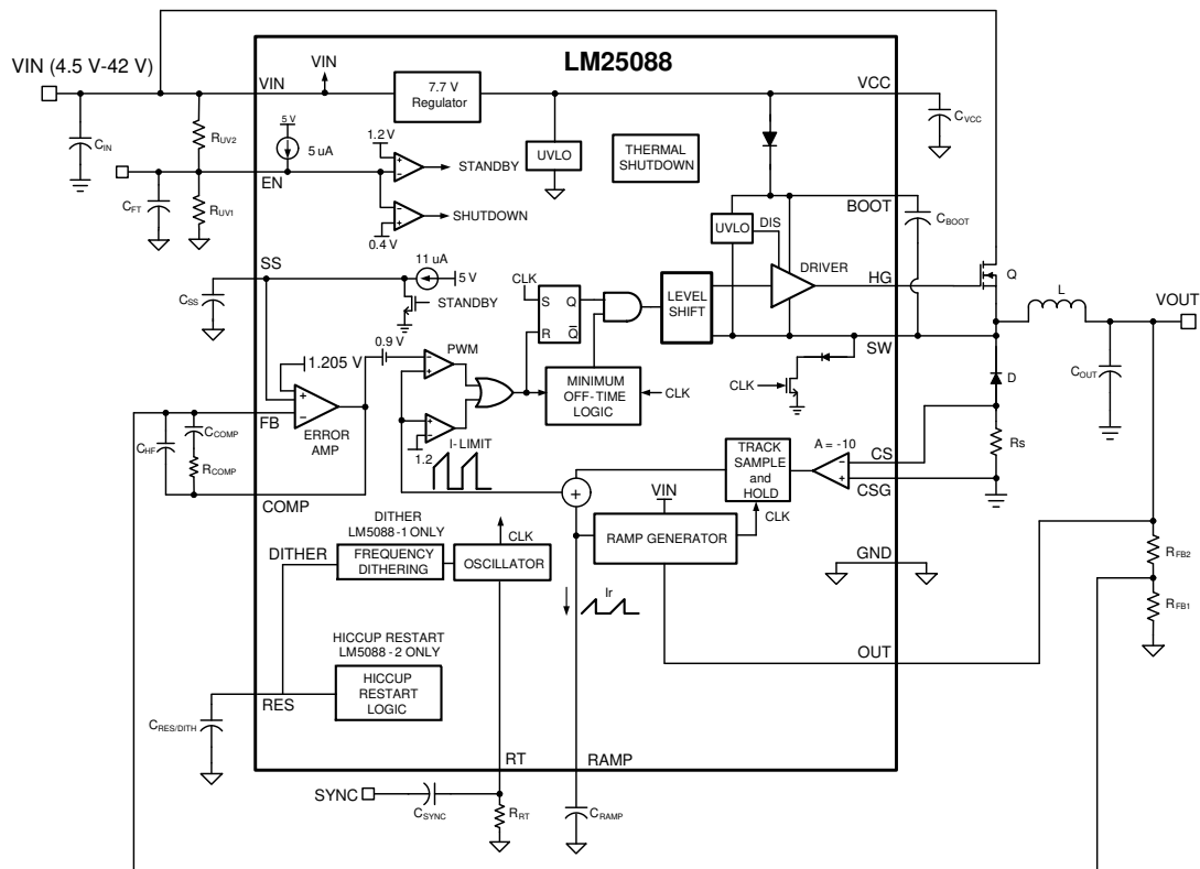
图 7-1. LM25088 功能块图
