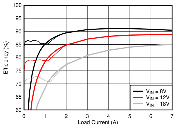
図 10-4 を参照してください。 図 8-2. 効率と負荷との関係 V_{OUT} = 3.3V f_{SW} = 2.1MHz
