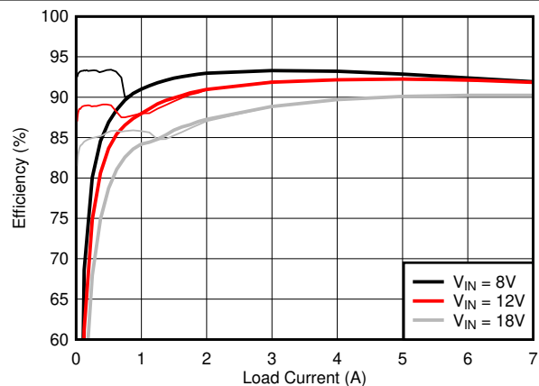
図 10-4 を参照してください。 図 8-1. 効率と負荷との関係 V_{OUT} = 5V f_{SW} = 2.1MHz
