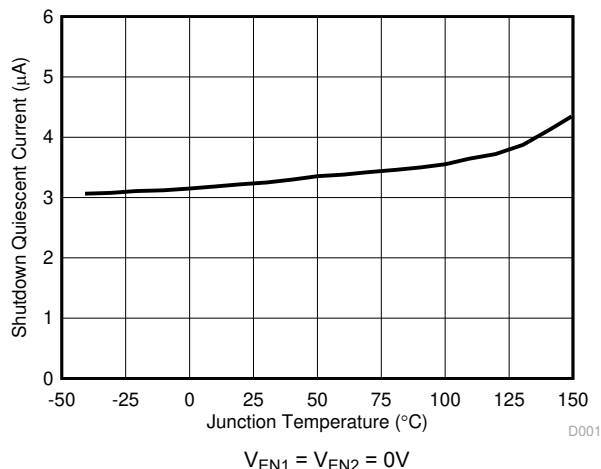
図 8-6. シャットダウン電流と温度との関係 V_{EN1} = V_{EN2} = 0V
