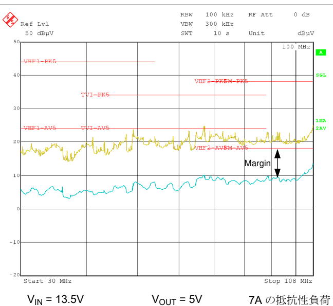
図 10-20. CISPR 25 Class 5 伝導 EMI、30MHz~108MHz
