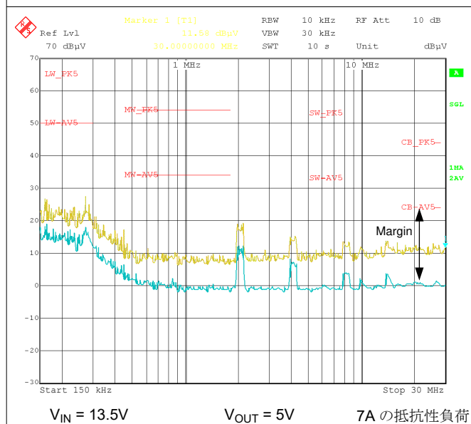
図 10-19. CISPR 25 Class 5 伝導 EMI、150kHz~30MHz
