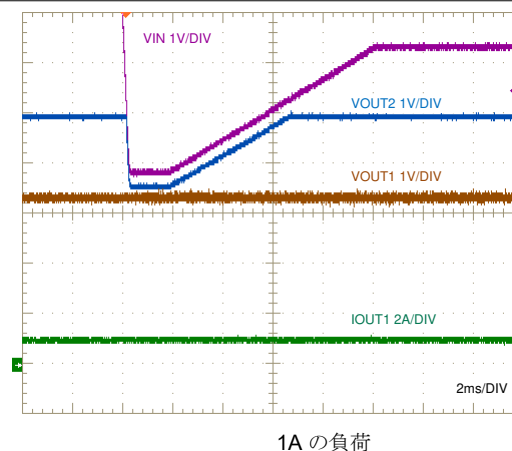
図 10-10. V_{IN} = 3.8V までのコールド・クランク応答
