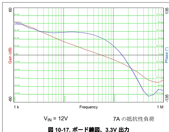
図 10-17. ボード線図、3.3V 出力
