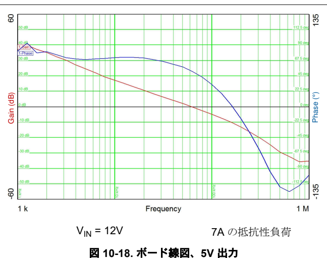
図 10-18. ボード線図、5V 出力
