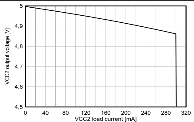
図 6-12. VCC2 LDO 出力電圧と VCC2 負荷電流との関係 V_{(VIN)} = 3.5\text{V} 、 V_{(BIAS)} = 12\text{V}
