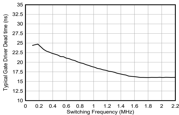
図 6-23. ゲートドライバ遅延 (デッド) 時間とスイッチング周波数との関係 SEL_MIN_DEADTIME_GDRV = 0b01、SEL_SCALE_DT = 0b0、 EN_CONST_TDEAD = 0b0
