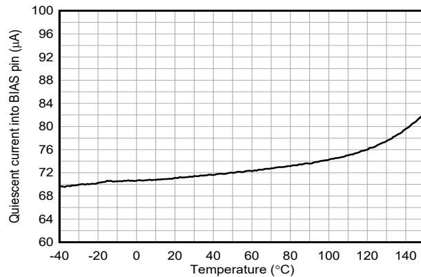
図 6-9. BIAS と BIAS の間の静止電流 V_{(BIAS)} = 12\text{V} 、 V_{(VIN)} = 3.5\text{V}
