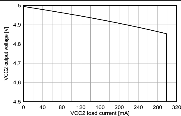
図 6-11. VCC2 LDO 出力電圧と VCC2 負荷電流との関係 V_{(VIN)} = 12\text{V} 、 V_{(BIAS)} = 0\text{V}
