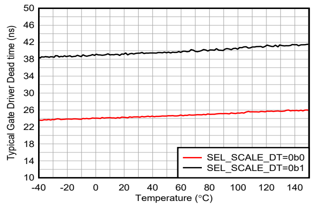
図 6-24. ゲートドライバ遅延 (デッド) 時間とスイッチング周波数との関係 f (sw) = 100kHz、SEL_MIN_DEADTIME_GDRV = 0b01、 EN_CONST_TDEAD = 0b0、ローサイド オフ、ハイサイドをオンに します
