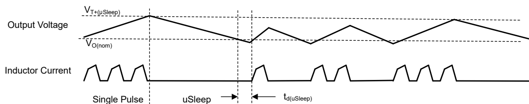
図 8-7. パワーセーブモード (µSleep 有効) のタイミング図
