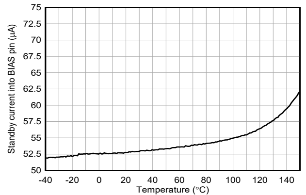
図 6-10. BIAS へのスタンバイ電流と温度との関係 V_{(VIN)} = 3.5\text{V} V_{(VIN)} = 12\text{V}
