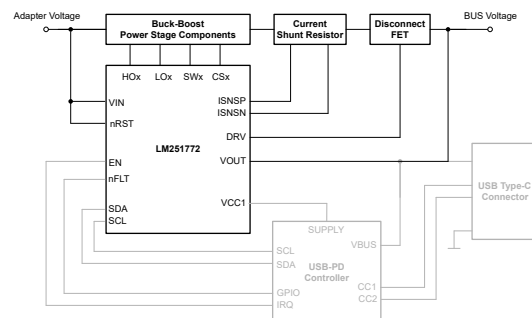
代表的なアプリケーション回路図
