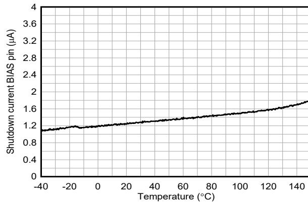
図 6-7. BIAS に流れ込むシャットダウン電流と温度との関係 V_{EN/UVLO} = 0\text{V} 、 V_{(VIN)} = 3.5\text{V} 、 V_{(BIAS)} = 12\text{V}
