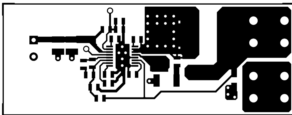
図 7-11. コンポーネント側
