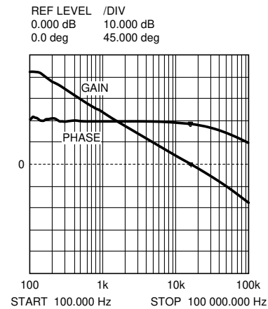
図 7-8. 全体的なループのゲインおよび位相
