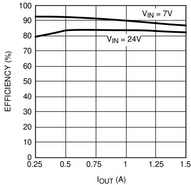
図 7-7. デモボード効率と I_{OUT} および V_{IN} との関係
