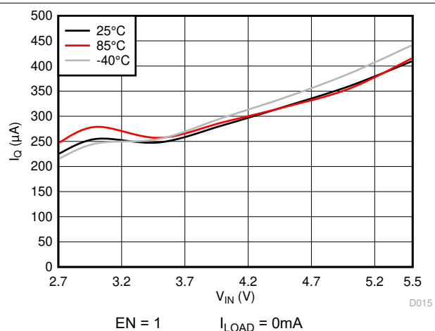
図 5-3. 静止電流
