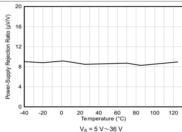
図 6-11. 電源除去比と温度との関係
