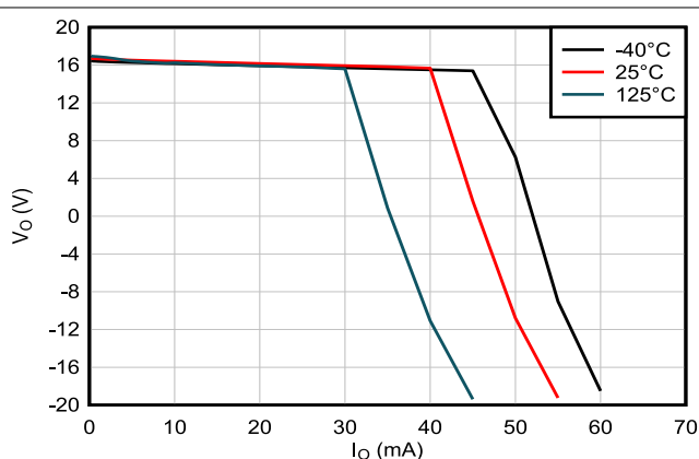
図 6-7. 出力電圧スイングと出力電流との関係 (ソース)
