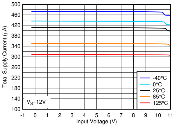
図 5-5. 合計電源電流と入力電圧との関係、12V
