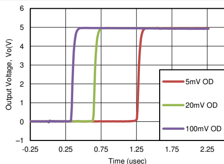
図 7-2. 各種オーバードライブの応答時間 (正の遷移)
