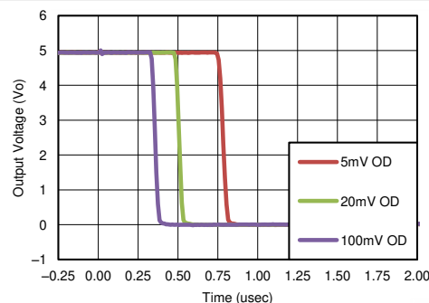
図 7-3. 各種オーバードライブの応答時間 (負の遷移)
